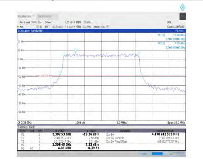
1-N30--15-5-M-9-CP-256QAM-Outer_Full-25@0-Ant1 1-4.471-4.880-≤5-PASS
