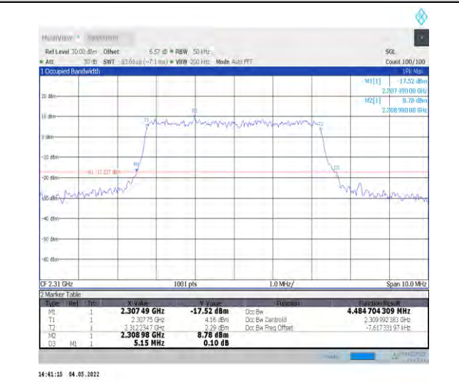
1-N30--15-5-M-7-CP-16QAM-Outer_Full-25@0-Ant1 -4.485-5.150-≤5-PASS
