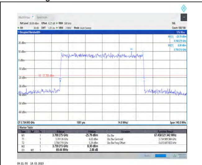
1-N78-3700-3800-30-70-L-7-CP-16QAM-Outer_Full-189@0-Ant1-67.458-69.440-≤70-PASS
