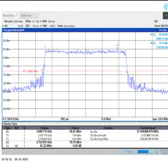
1-N78-3700-3800-30-60-L-5-DFT-256QAM-Outer_Fu II-162@0-Ant1-8.56-9.720-≤60-PASS
