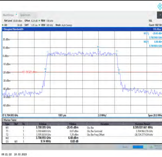
1-N78-3700-3800-30-10-L-9-CP-256QAM-Outer_Full -24@0-Ant1-8.595-9.140-≤10-PASS
