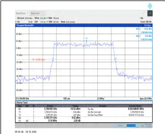
1-N78-3700-3800-30-10-L-5-DFT-256QAM-Outer_Fu II-24@0-Ant1-8.566-9.160-≤10-PASS
