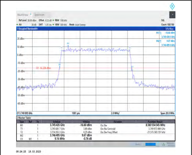
1-N78-3700-3800-30-10-M-7-CP-16QAM-Outer_Full -24@0-Ant1-8.584-9.160-≤10-PASS
