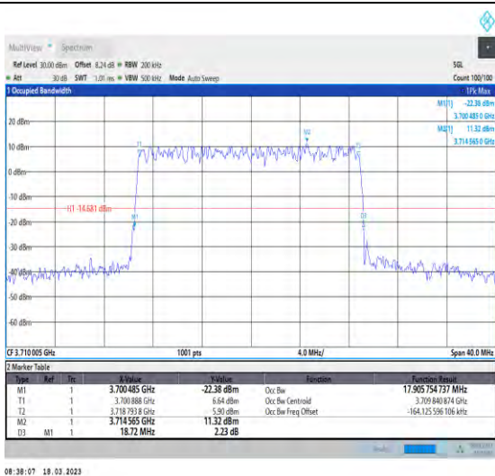
1-N78-3700-3800-30-20-L-3-DFT-16QAM-Outer_Full -50@0-Ant1-17.906-18.720-≤20-PASS
