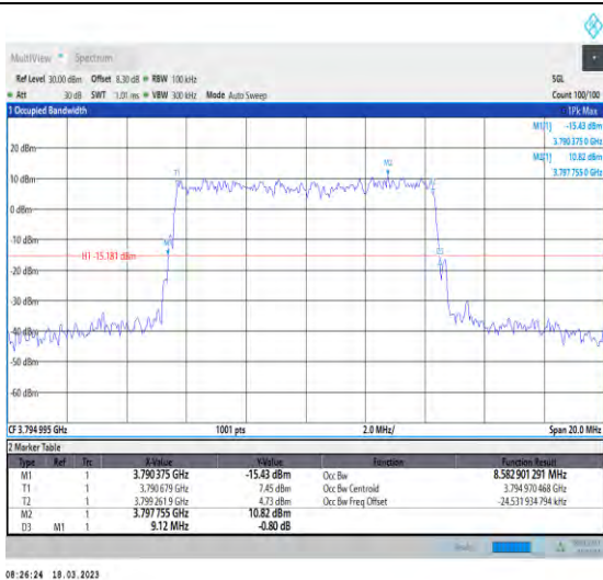
1-N78-3700-3800-30-10-H-3-DFT-16QAM-Outer_Ful I-24@0-Ant1-8.583-9.120-≤10-PASS
