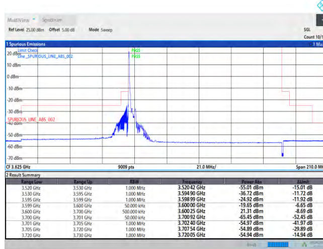
Band43-5MHz-QPSK-43615-1RB#0
