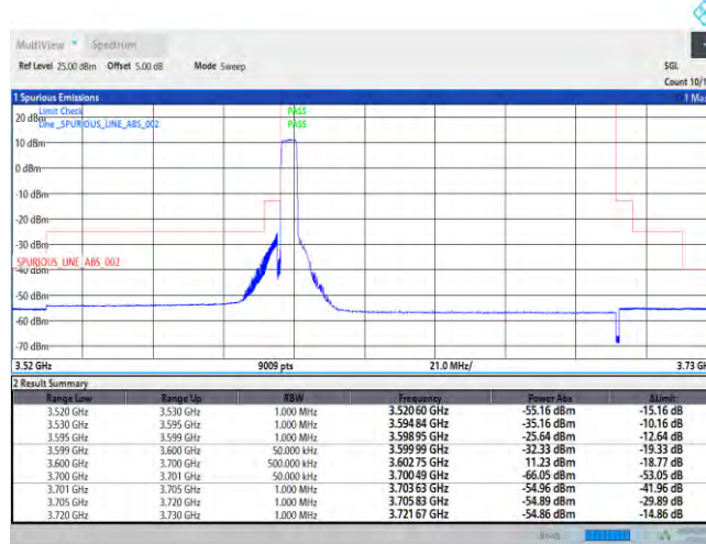
Band43-5MHz-QPSK-43615-25RB#0
