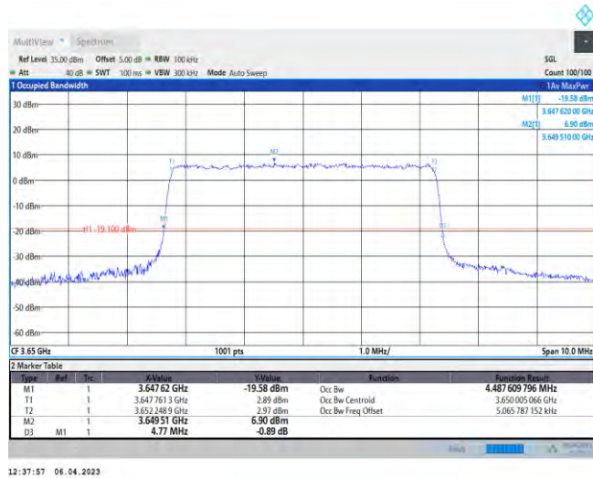
Band43-5MHz-QPSK-44090-25RB#0
