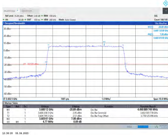
Band43-5MHz-QPSK-44090-25RB#0
