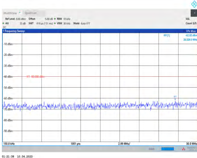
Band43-20MHz-QPSK-43690-1RB#0-Range2:0.15~30MHz
