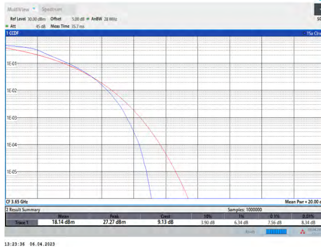
Band43-20MHz-QPSK-44090-100RB#0
