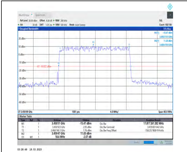
1-N78-3450-3550-30-20-L-3-DFT-16QAM-Outer_Full -50@0-Ant1-17.817-18.600-≤20-PASS
