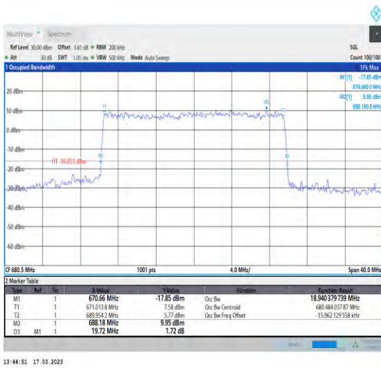
1-N71-PC3-15-20-M-8-CP-64QAM-Outer_Full-106@ 0-Ant1-18.94-19.720-≤20-PASS
