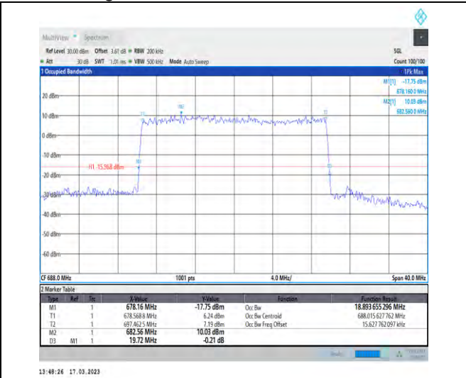
1-N71-PC3-15-20-H-8-CP-64QAM-Outer_Full-106@ 0-Ant1-18.894-19.720-≤20-PASS
