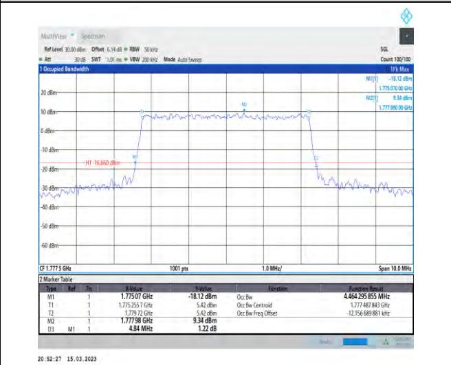
1-N66-PC3-15-5-H-6-CP-QPSK-Outer_Full-25@0-A nt1-4.464-4.840-≤5-PASS
