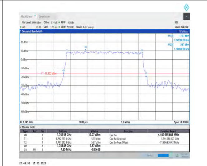
1-N66-PC3-15-5-M-7-CP-16QAM-Outer_Full-25@0- Ant1-4.45-4.850-≤5-PASS
