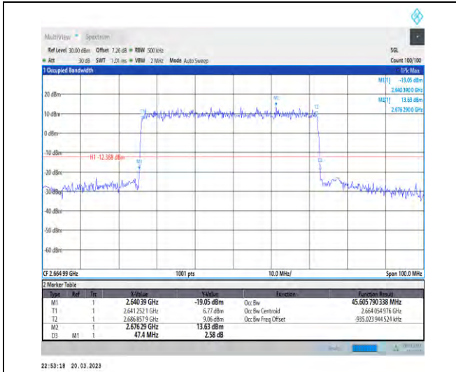
1-N41-30-50-H-4-DFT-64QAM-Outer_Full-128@0-A nt1-45.606-47.400-≤50-PASS
