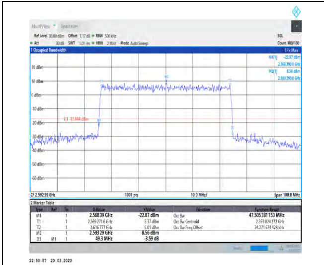
1-N41-30-50-M-9-CP-256QAM-Outer_Full-133@0-A nt1-47.505-49.300-≤50-PASS
