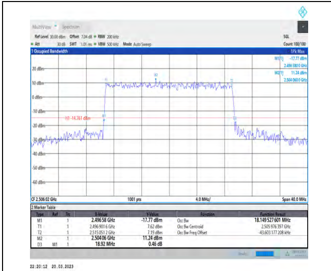
1-N41-30-20-L-7-CP-16QAM-Outer_Full-51@0-Ant1 -18.15-18.920-≤20-PASS
