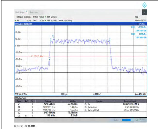
1-N41-30-20-L-5-DFT-256QAM-Outer_Full-50@0-A nt1-17.843-18.600-≤20-PASS
