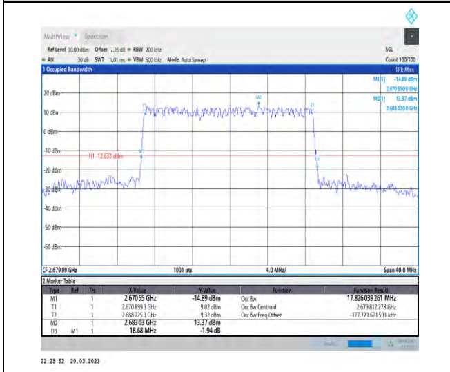
1-N41-30-20-H-3-DFT-16QAM-Outer_Full-50@0-Ant1 1-17.826-18.680-≤20-PASS
