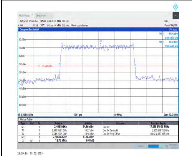
1-N41-30-20-L-1-DFT-QPSK-Outer_Full-50@0-Ant1 -17.813-18.760-≤20-PASS
