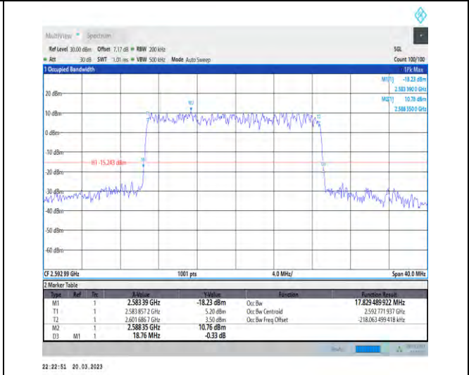
1-N41-30-20-M-5-DFT-256QAM-Outer_Full-50@0-A nt1-17.829-18.760-≤20-PASS
