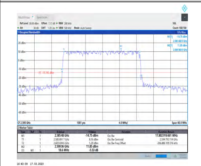
1-N38-30-20-M-5-DFT-256QAM-Outer_Full-50@0-A nt1-17.803-18.600-≤20-PASS
