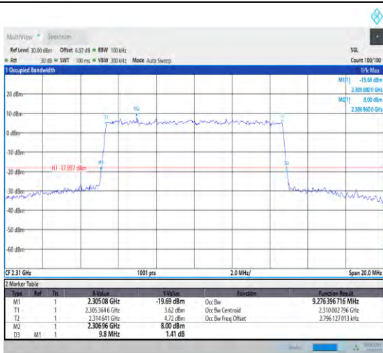
1-N30-PC3-15-10-M-9-CP-256QAM-Outer_Full-52@ 0-Ant1-9.276-9.800-≤10-PASS
