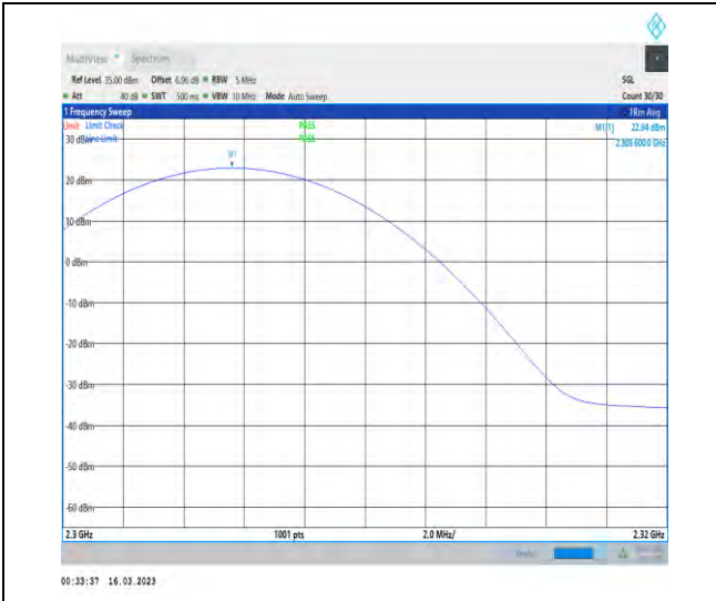
1-N30-PC3-15-10-M-1-DFT-PI2BPSK-Inner_1RB_L eft-1@1-2300-2320-Ant1-2305.60-22.94-99-PASS
