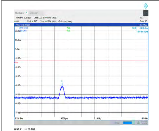
1-N14-PC3-15-10-M-1-DFT-PI2BPSK-Inner_1RB_L eft-1@1-1559-1610-Ant1-1577.21--38.68--13-PASS
