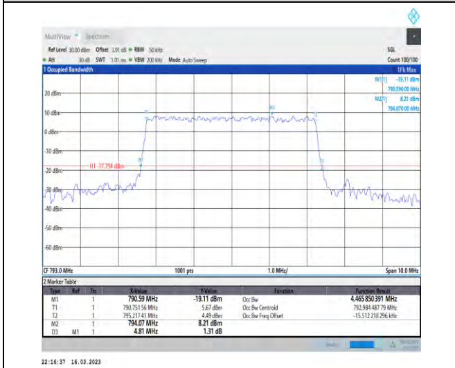
1-N14-PC3-15-5-M-6-CP-QPSK-Outer_Full-25@0-A nt1-4.466-4.810-≤5-PASS
