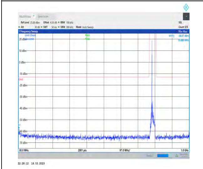
1-N14-PC3-15-10-M-1-DFT-PI2BPSK-Inner_1RB_L eft-1@1-30-1000-Ant1-33.88--58.07--13-PASS
