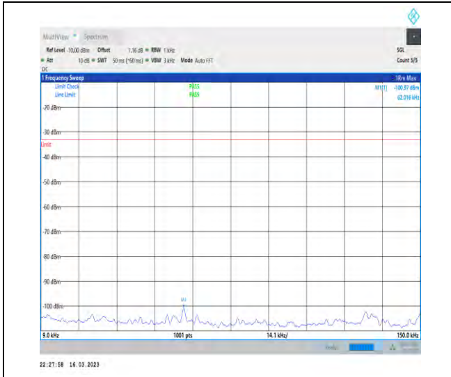
1-N14-PC3-15-10-M-1-DFT-PI2BPSK-Inner_1RB_L eft-1@1-0.009-0.15-Ant1-0.06--100.97--33-PASS
