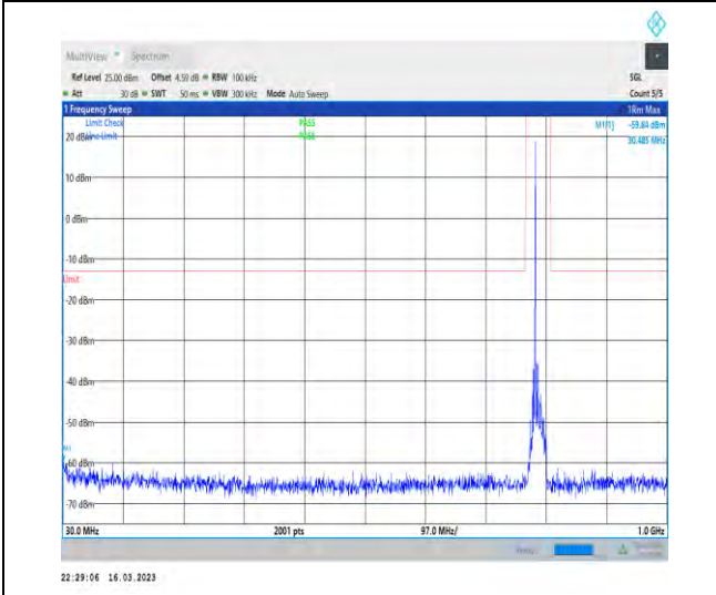
1-N14-PC3-15-10-H-1-DFT-PI2BPSK-Inner_1RB_L eft-1@1-30-1000-Ant1-30.49--59.84--13-PASS
