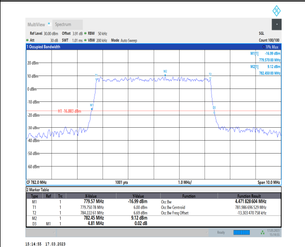
1-N13-PC3-15-5-M-7-CP-16QAM-Outer_Full-25@0- Ant1-4.472-4.810-≤5-PASS
