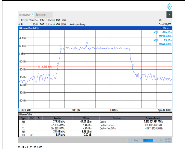
1-N13-PC3-15-5-M-6-CP-QPSK-Outer_Full-25@0-A Ant1-4.477-4.870-≤5-PASS
