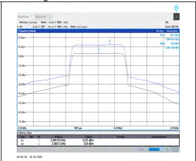
1-N7-PC3-15-20-H-2-CP-256QAM-Outer_Full-106@ 0-Ant1-9.56-100%-0.00-9.56-PASS-≤13
