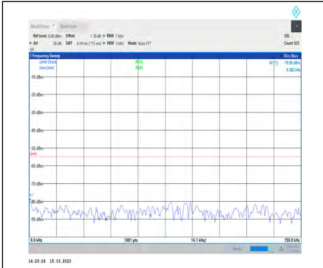
1-N7-PC3-15-20-H-1-DFT-PI2BPSK-Inner_1RB_Lef t-1@1-0.009-0.15-Ant1-0.01--79.95--55-PASS
