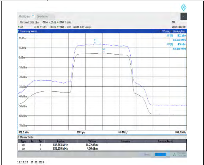
1-N5-PC3-15-20-H-2-CP-256QAM-Outer_Full-106@ 0-Ant1-9.72-100%-0.00-9.72-PASS≤13
