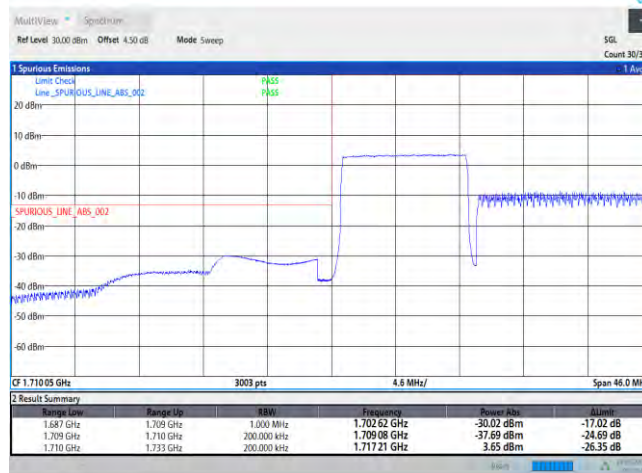
66-66-10MHz-15MHz-QPSK-QPSK-132025-132145-50RB#0-75RB#0
