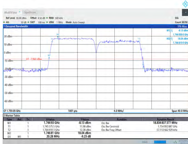
66-66-10MHz-10MHz-QPSK-QPSK-132373-132472-50RB#0-50RB#0
