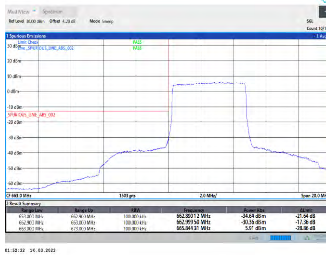
Band71-5MHz-QPSK-133147-25RB#0
