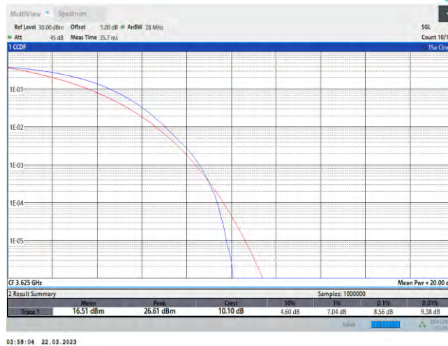
48-48-20MHz-20MHz-QPSK-QPSK-55891-56089-100RB#0-100RB#0
