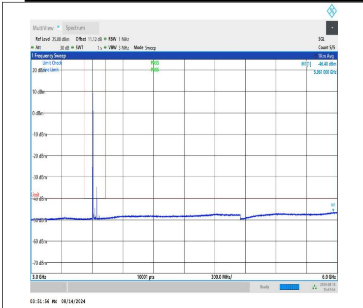
NTNV-n48-PC3-30-40-M-CP-QPSK-Edge_1RB_Left-3000-6000-P ASS
