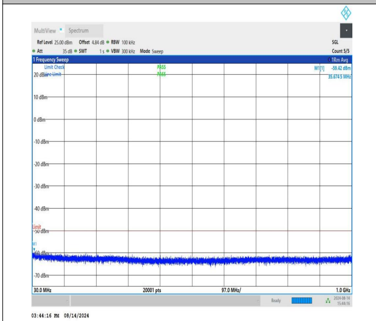
NTNV-n48-PC3-30-20-L-CP-QPSK-Edge_1RB_Left-30-1000-PAS S
