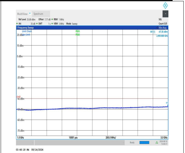
NTNV-n48-PC3-30-20-M-CP-QPSK-Edge_1RB_Left-1000-3000-PA SS
