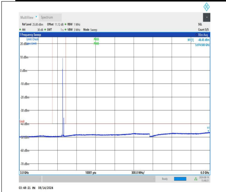
NTNV-n48-PC3-30-20-H-CP-QPSK-Edge_1RB_Left-3000-6000-P ASS
