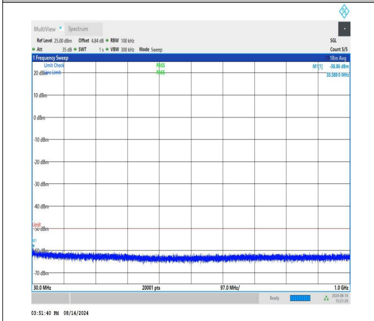
NTNV-n48-PC3-30-40-M-CP-QPSK-Edge_1RB_Left-30-1000-PASS
