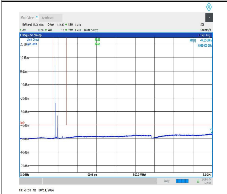
NTNV-n48-PC3-30-40-L-CP-QPSK-Edge_1RB_Left-3000-6000-P ASS
