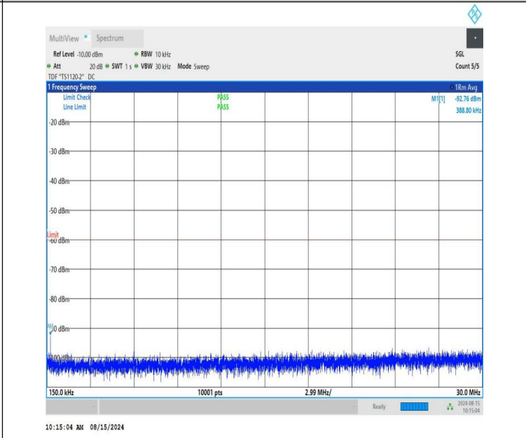
NTVN-n48-PC3-30-40-L-CP-QPSK-Edge_1RB_Left-0.15-30-PASS
