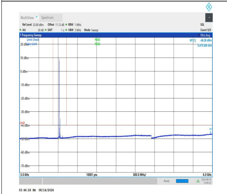
NTNV-n48-PC3-30-20-M-CP-QPSK-Edge_1RB_Left-3000-6000-P ASS
