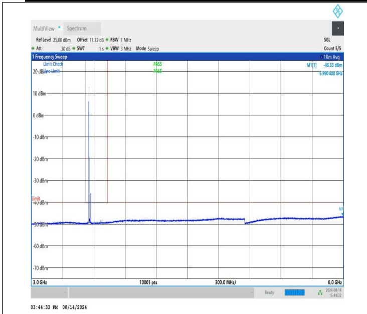
NTNV-n48-PC3-30-20-L-CP-QPSK-Edge_1RB_Left-3000-6000-P ASS
