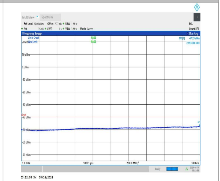
NTNV-n48-PC3-30-20-L-CP-QPSK-Edge_1RB_Left-1000-3000-PASS
