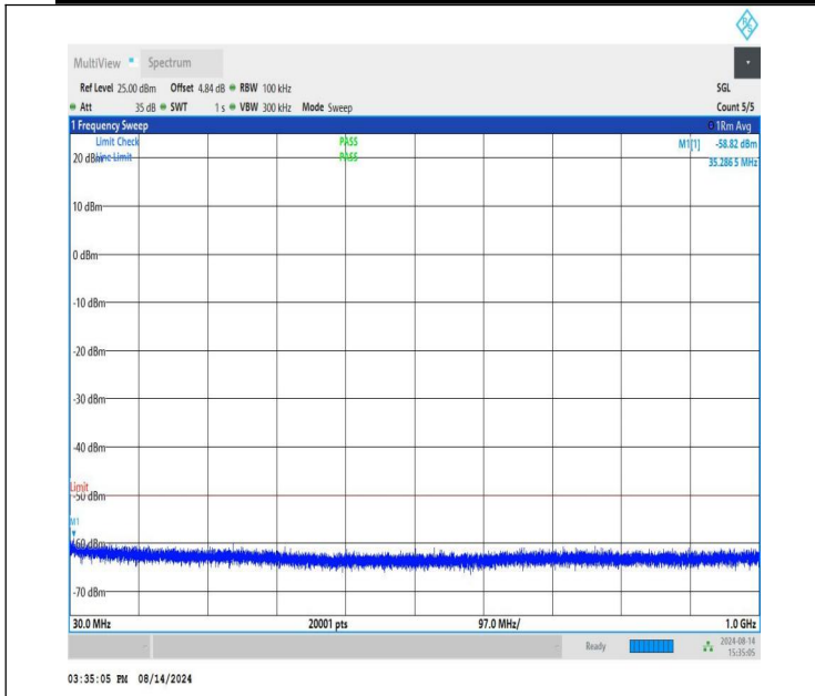
NTNV-n48-PC3-30-10-M-CP-QPSK-Edge_1RB_Left-30-1000-PA SS
