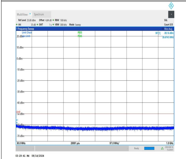
NTNV-n48-PC3-30-40-M-CP-QPSK-Edge_1RB_Left-30-1000-PASS
