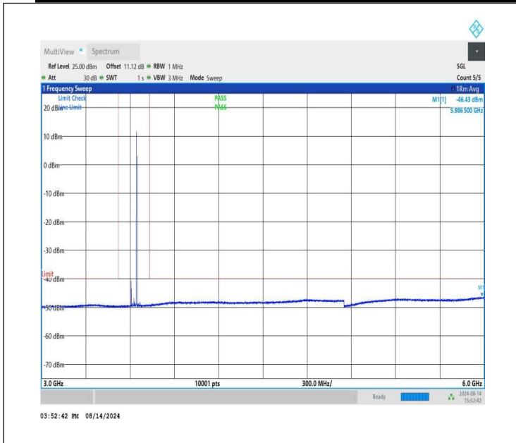
NTNV-n48-PC3-30-20-H-CP-QPSK-Edge_1RB_Left-3000-6000-P ASS
