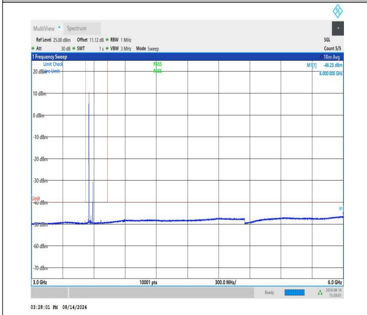
NTNV-n48-PC3-30-40-L-CP-QPSK-Edge_1RB_Left-3000-6000-P ASS
