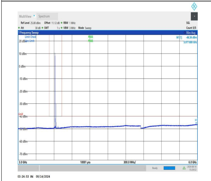
NTNV-n48-PC3-30-20-M-CP-QPSK-Edge_1RB_Left-3000-6000-P ASS
