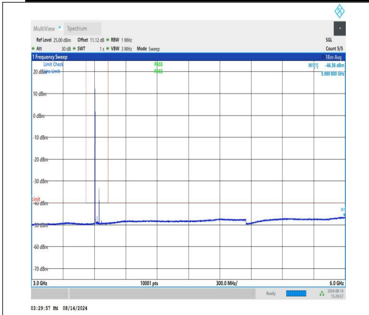
NTNV-n48-PC3-30-40-M-CP-QPSK-Edge_1RB_Left-3000-6000-P ASS
