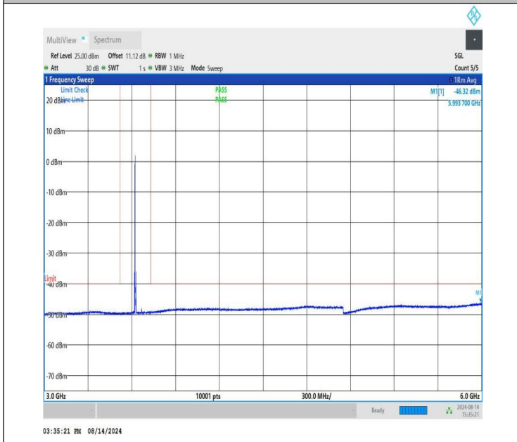
NTNV-n48-PC3-30-10-M-CP-QPSK-Edge_1RB_Left-3000-6000-P ASS
