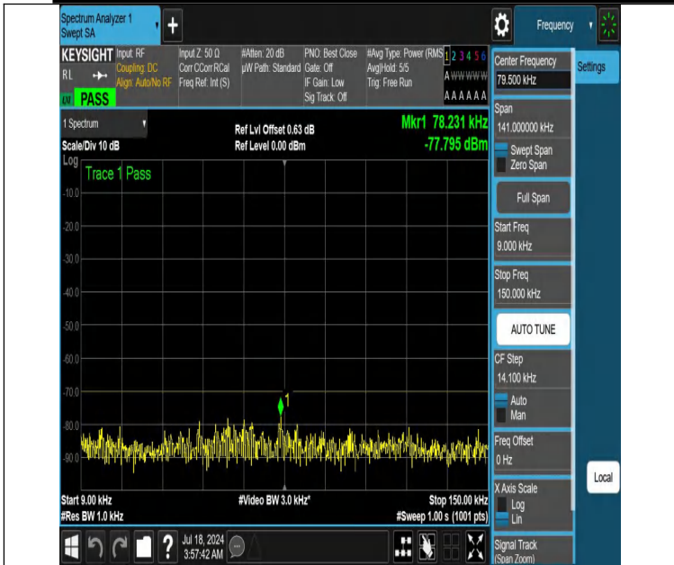
NTNV-DC_13A_n48A-PC3-30-5+30-M+L-N/A-N/A-DFT-PI2BPSK-Edge_1RB_Left-0.009-0.15-PASS
