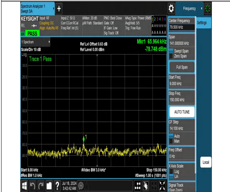
NTNV-DC_13A_n48A-PC3-30-5+20-M+L-N/A-N/A-DFT-QPSK-Edge_1RB_Left-0.009-0.15-PASS
