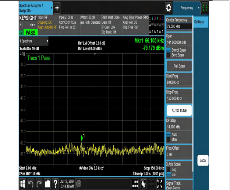
NTNV-DC_13A_n48A-PC3-30-5+20-M+L-N/A-N/A-DFT-QPSK-Edge _1RB_Right-0.009-0.15-PASS
