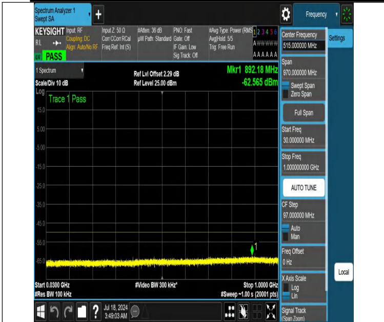
NTNV-DC_13A_n48A-PC3-30-5+20-M+M-N/A-N/A-DFT-QPSK-Edge_1RB_Left-30-1000-PASS
