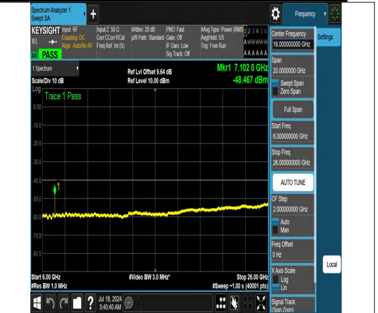
NTNV-DC_13A_n48A-PC3-30-5+20-M+L-N/A-N/A-DFT-PI2BPSK-E dge_1RB_Left-6000-26000-PASS
