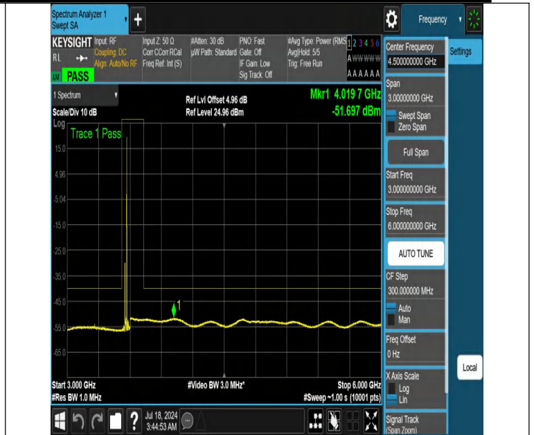
NTNV-DC_13A_n48A-PC3-30-5+20-M+L-N/A-N/A-DFT-QPSK-Edge _1RB_Right-3000-6000-PASS
