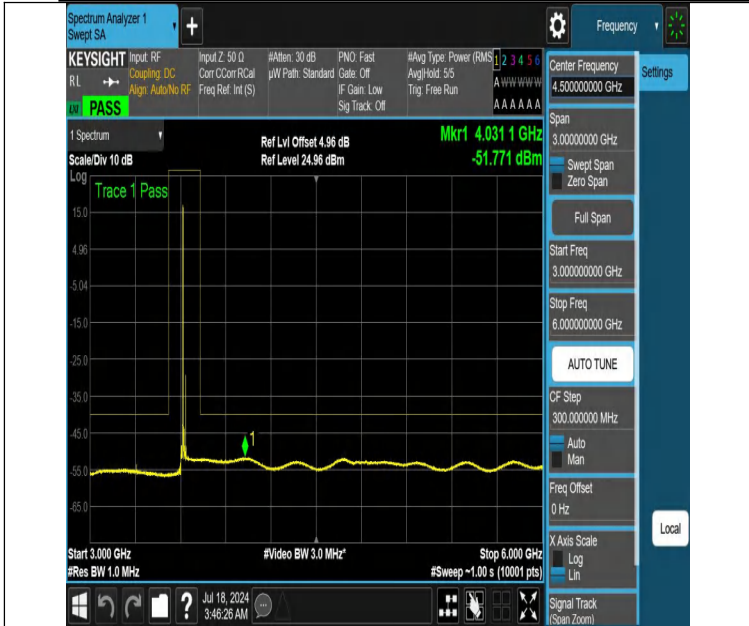
NTVN-DC_13A_n48A-PC3-30-5+20-M+M-N/A-N/A-DFT-PI2BPSK-Edge_1RB_Left-3000-6000-PASS
