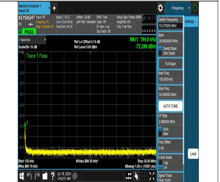
NTNV-DC_13A_n48A-PC3-30-5+20-M+L-N/A-N/A-DFT-QPSK-Edge_1RB_Left-0.15-30-PASS
