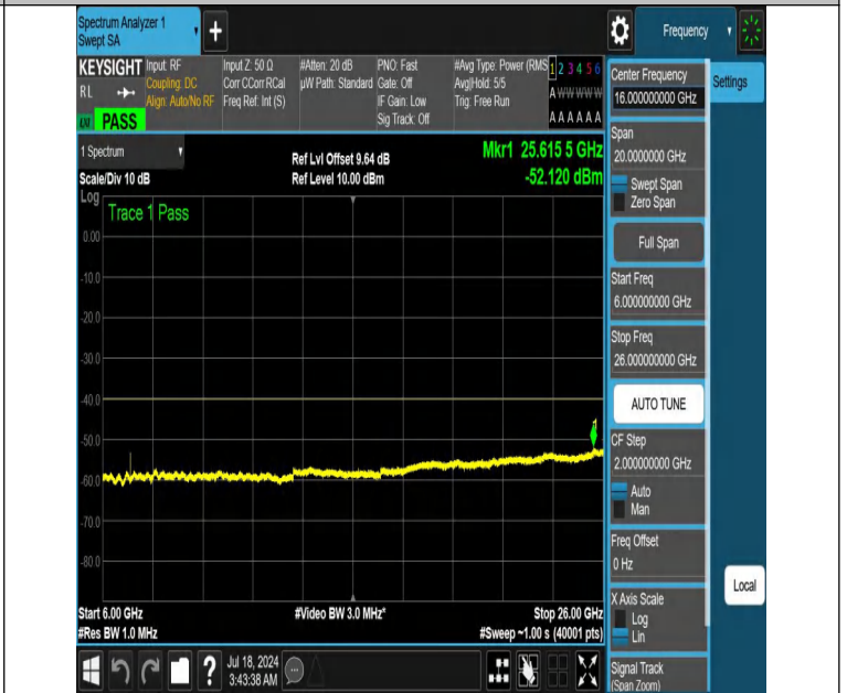
NTNV-DC_13A_n48A-PC3-30-5+20-M+L-N/A-N/A-DFT-QPSK-Edge _1RB_Left-6000-26000-PASS
