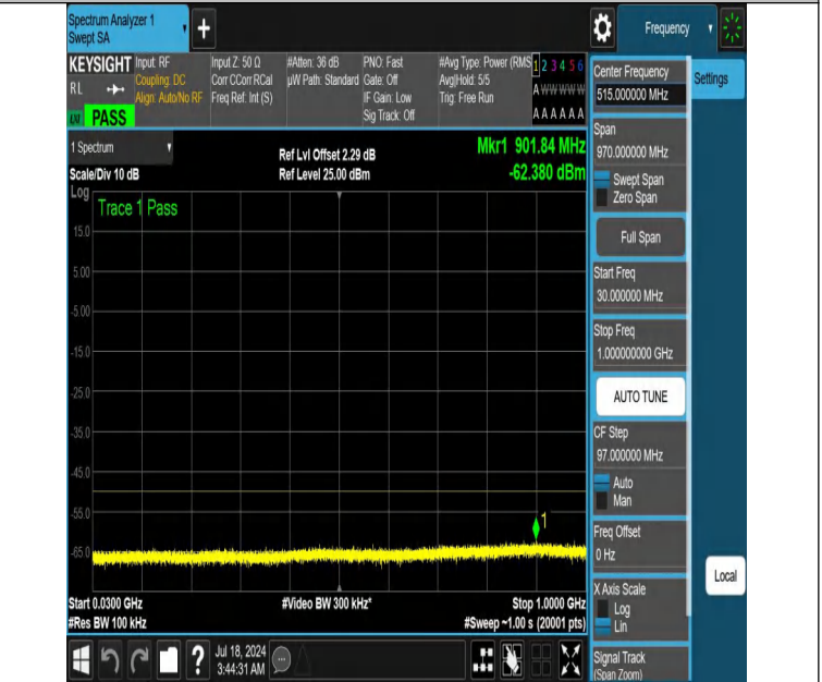
NTNV-DC_13A_n48A-PC3-30-5+20-M+L-N/A-N/A-DFT-QPSK-Edge _1RB_Right-30-1000-PASS
