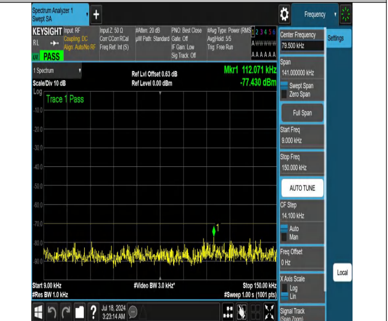
NTNV-DC_13A_n48A-PC3-30-5+15-M+L-N/A-N/A-DFT-PI2BPSK-E dge_1RB_Right-0.009-0.15-PASS
