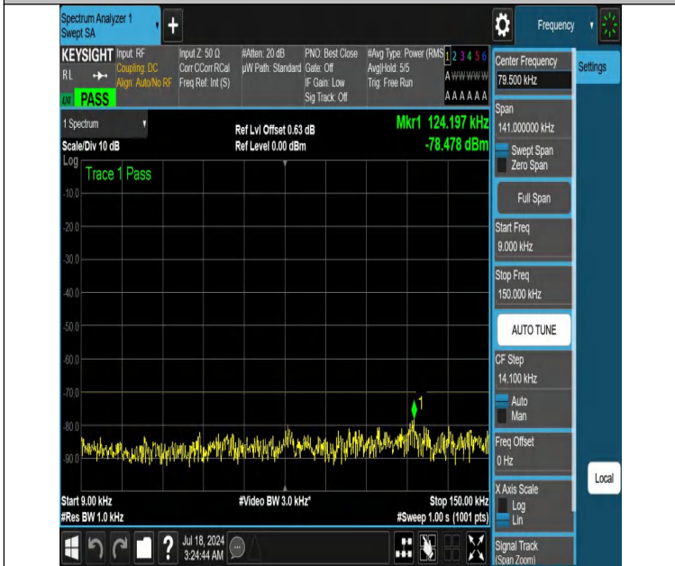
NTNV-DC_13A_n48A-PC3-30-5+15-M+L-N/A-N/A-DFT-QPSK-Edge_1RB_Left-0.009-0.15-PASS
