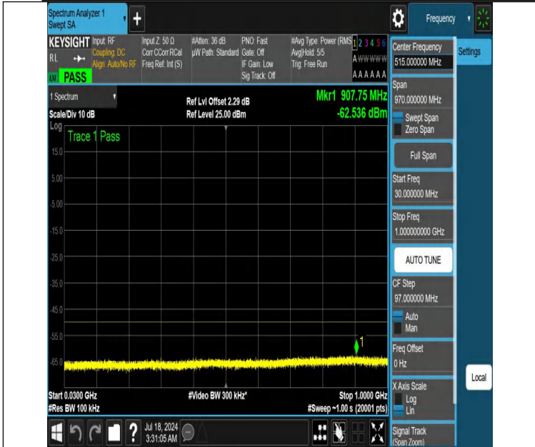
NTNV-DC_13A_n48A-PC3-30-5+15-M+M-N/A-N/A-DFT-QPSK-Edge_1RB_Left-30-1000-PASS
