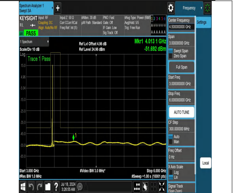
NTNV-DC_13A_n48A-PC3-30-5+15-M+L-N/A-N/A-DFT-QPSK-Edge _1RB_Right-3000-6000-PASS
