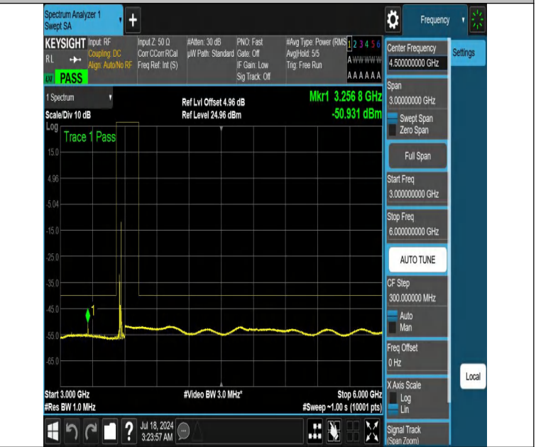
NTNV-DC_13A_n48A-PC3-30-5+15-M+L-N/A-N/A-DFT-PI2BPSK-E dge_1RB_Right-3000-6000-PASS
