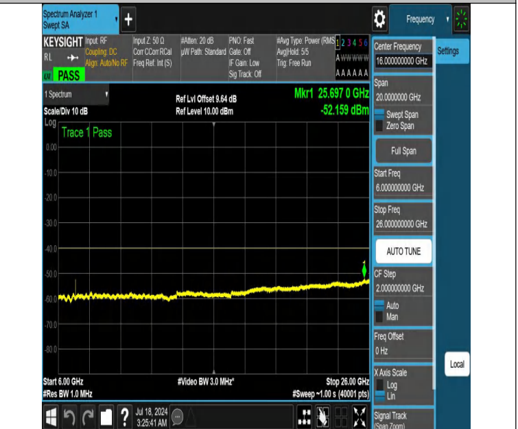
NTNV-DC_13A_n48A-PC3-30-5+15-M+L-N/A-N/A-DFT-QPSK-Edge _1RB_Left-6000-26000-PASS
