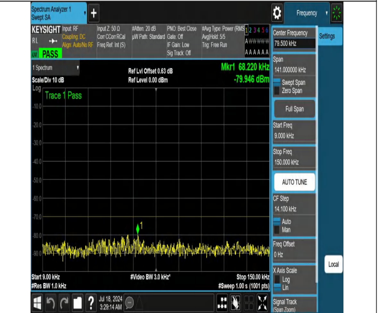
NTVN-DC_13A_n48A-PC3-30-5+15-M+M-N/A-N/A-DFT-PI2BPSK-E dge_1RB_Right-0.009-0.15-PASS
