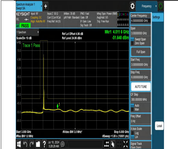
NTVN-DC_13A_n48A-PC3-30-5+15-M+M-N/A-N/A-DFT-PI2BPSK-Edge_1RB_Left-3000-6000-PASS
