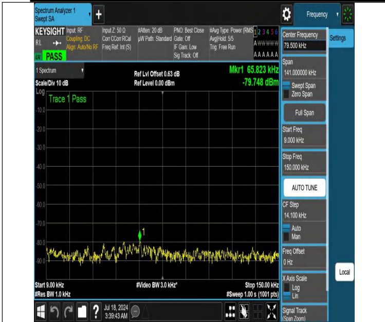
NTNV-DC_13A_n48A-PC3-30-5+20-M+L-N/A-N/A-DFT-PI2BPSK-Edge_1RB_Left-0.009-0.15-PASS
