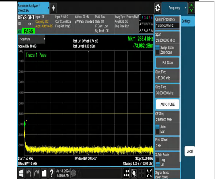
NTNV-DC_13A_n48A-PC3-30-5+20-M+L-N/A-N/A-DFT-PI2BPSK-E dge_1RB_Left-0.15-30-PASS
