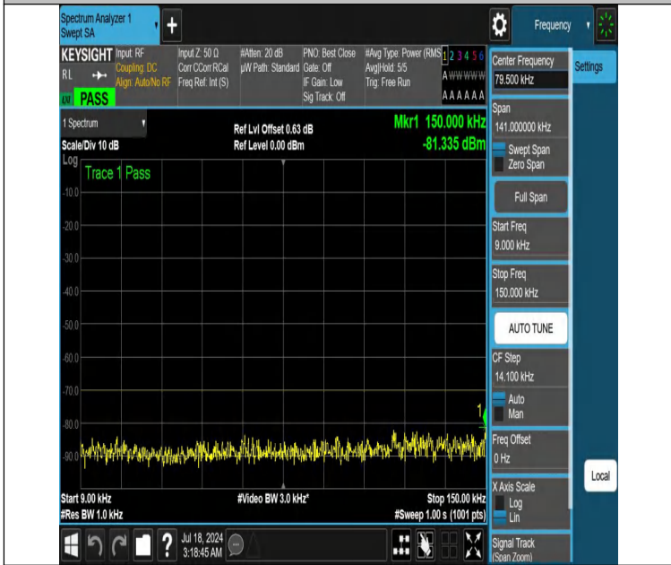
NTNV-DC_13A_n48A-PC3-30-5+10-M+H-N/A-N/A-DFT-QPSK-Edge_1RB_Left-0.009-0.15-PASS
