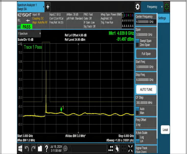
NTVN-DC_13A_n48A-PC3-30-5+10-M+M-N/A-N/A-DFT-PI2BPSK-E_dge_1RB_Right-3000-6000-PASS
