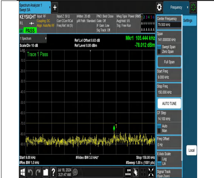
NTNV-DC_13A_n48A-PC3-30-5+15-M+L-N/A-N/A-DFT-PI2BPSK-Edge_1RB_Left-0.009-0.15-PASS
