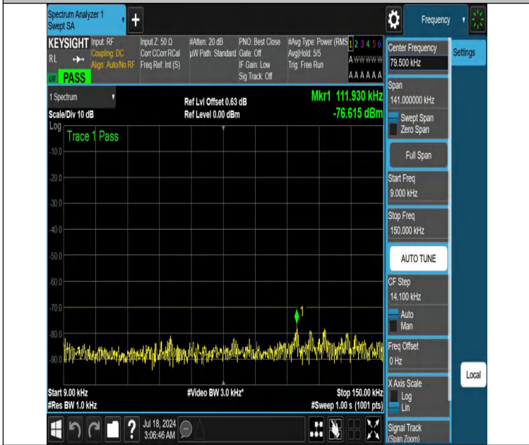
NTNV-DC_13A_n48A-PC3-30-5+10-M+L-N/A-N/A-DFT-QPSK-Edge_1RB_Left-0.009-0.15-PASS
