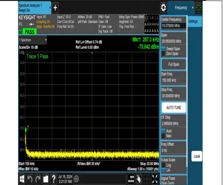
NTNV-DC_13A_n48A-PC3-30-5+15-M+L-N/A-N/A-DFT-PI2BPSK-E dge_1RB_Left-0.15-30-PASS
