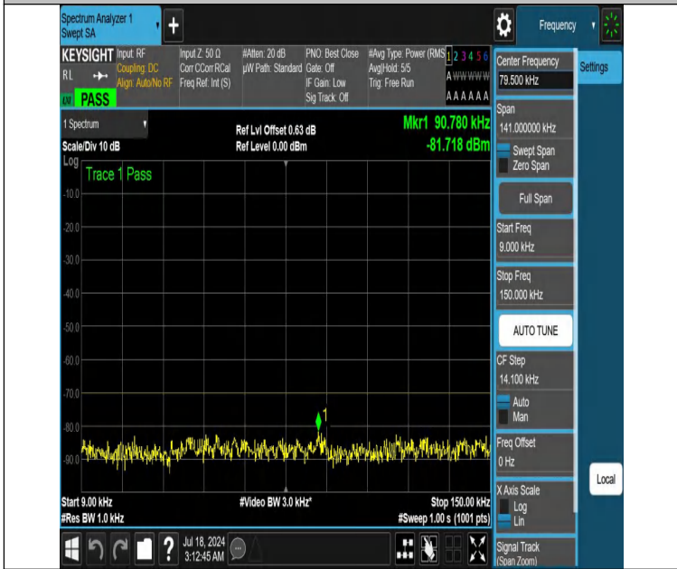
NTNV-DC_13A_n48A-PC3-30-5+10-M+M-N/A-N/A-DFT-QPSK-Ed ge_1RB_Left-0.009-0.15-PASS
