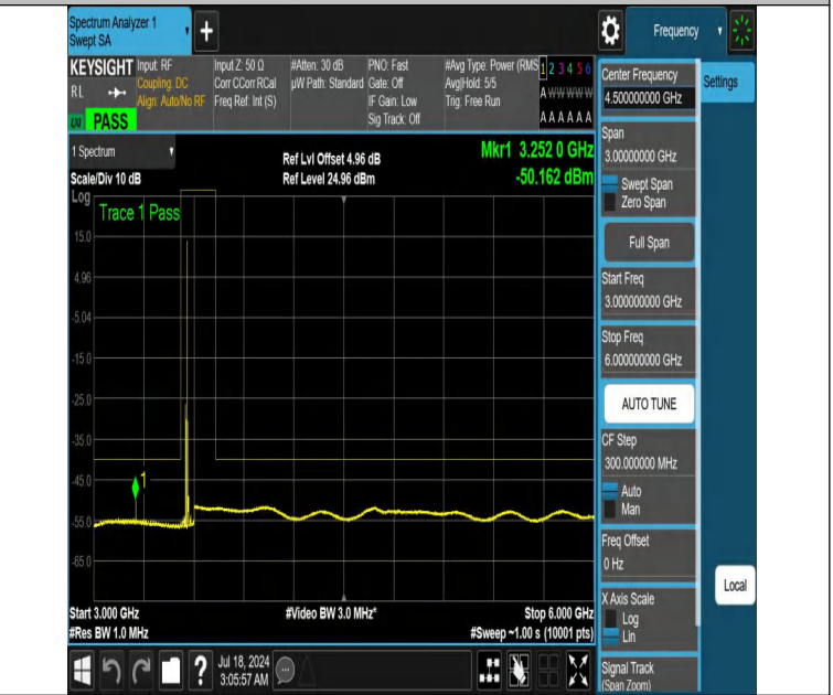
NTNV-DC_13A_n48A-PC3-30-5+10-M+L-N/A-N/A-DFT-PI2BPSK-E dge_1RB_Right-3000-6000-PASS
