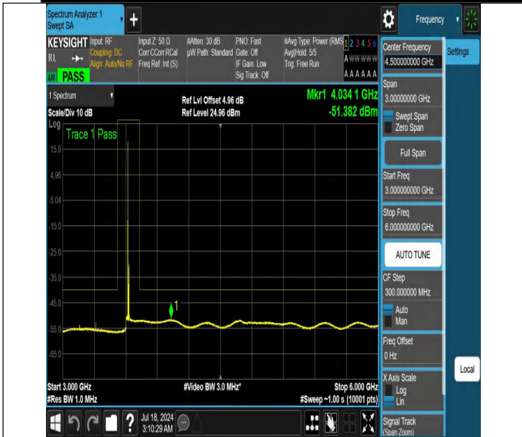
NTVN-DC_13A_n48A-PC3-30-5+10-M+M-N/A-N/A-DFT-PI2BPSK-Edge_1RB_Left-3000-6000-PASS
