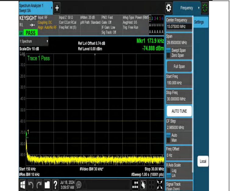
NTNV-DC_13A_n48A-PC3-30-5+10-M+M-N/A-N/A-DFT-PI2BPSK-E dge_1RB_Left-0.15-30-PASS
