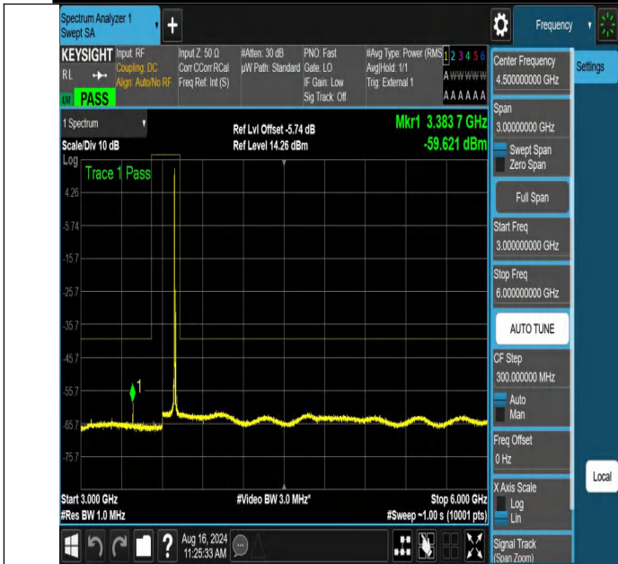
NTNV-DC_13A_n48A-PC3-30-5+10-M+H-N/A-N/A-DFT-PI2BPSK-Edge_1RB_Left-3000-6000-PASS
