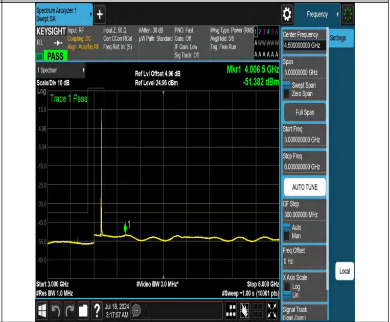
NTNV-DC_13A_n48A-PC3-30-5+10-M+H-N/A-N/A-DFT-PI2BPSK-E dge_1RB_Right-3000-6000-PASS
