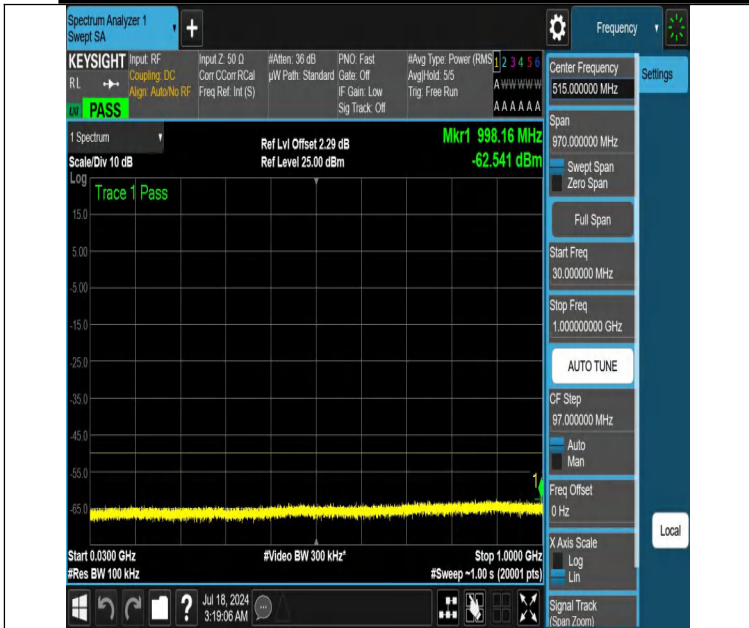
NTNV-DC_13A_n48A-PC3-30-5+10-M+H-N/A-N/A-DFT-QPSK-Edg e_1RB_Left-30-1000-PASS
