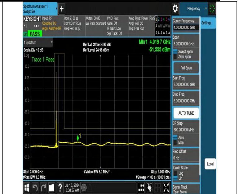
NTNV-DC_13A_n48A-PC3-30-5+10-M+L-N/A-N/A-DFT-QPSK-Edge _1RB_Right-3000-6000-PASS
