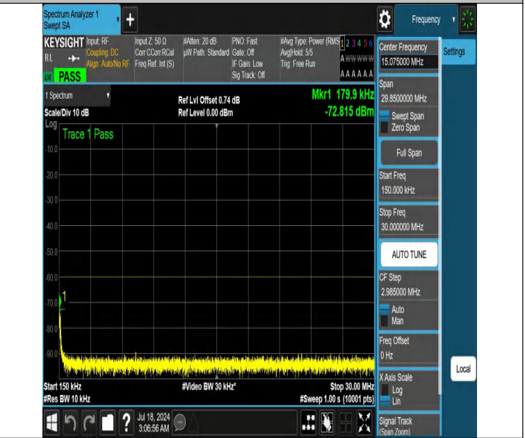
NTNV-DC_13A_n48A-PC3-30-5+10-M+L-N/A-N/A-DFT-QPSK-Edge_1RB_Left-0.15-30-PASS
