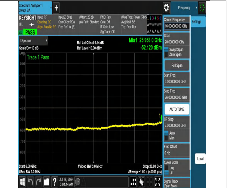
NTNV-DC_13A_n48A-PC3-30-5+10-M+L-N/A-N/A-DFT-PI2BPSK-E dge_1RB_Left-6000-26000-PASS
