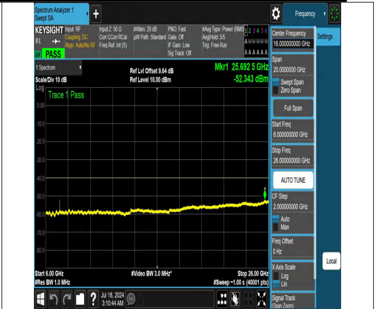
NTVN-DC_13A_n48A-PC3-30-5+10-M+M-N/A-N/A-DFT-PI2BPSK-E_dge_1RB_Left-6000-26000-PASS
