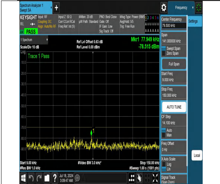
NTNV-DC_13A_n48A-PC3-30-5+10-M+M-N/A-N/A-DFT-PI2BPSK-Edge_1RB_Left-0.009-0.15-PASS
