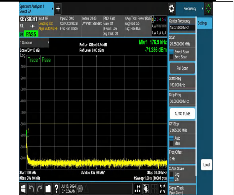
NTNV-DC_13A_n48A-PC3-30-5+10-M+H-N/A-N/A-DFT-PI2BPSK-E dge_1RB_Left-0.15-30-PASS
