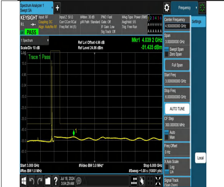
NTNV-DC_13A_n48A-PC3-30-5+10-M+L-N/A-N/A-DFT-PI2BPSK- Edge_1RB_Left-3000-6000-PASS
