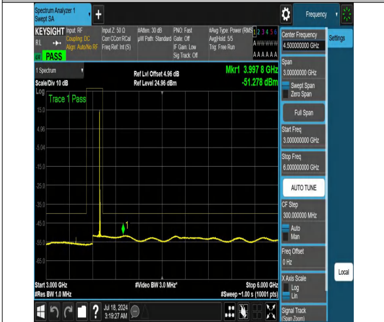
NTNV-DC_13A_n48A-PC3-30-5+10-M+H-N/A-N/A-DFT-QPSK-Edg e_1RB_Left-3000-6000-PASS
