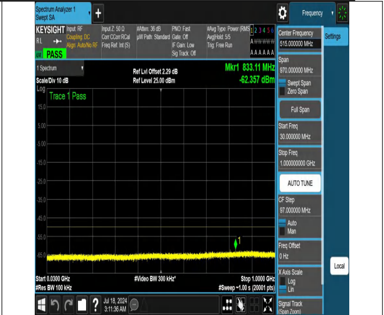
NTVN-DC_13A_n48A-PC3-30-5+10-M+M-N/A-N/A-DFT-PI2BPSK-E_dge_1RB_Right-30-1000-PASS
