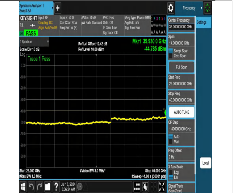
NTNV-DC_13A_n48A-PC3-30-5+10-M+L-N/A-N/A-DFT-PI2BPSK-E dge_1RB_Right-26000-40000-PASS
