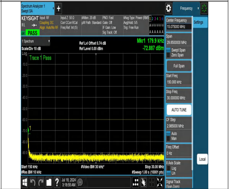
NTNV-DC_13A_n48A-PC3-30-5+10-M+H-N/A-N/A-DFT-QPSK-Edge_1RB_Left-0.15-30-PASS
