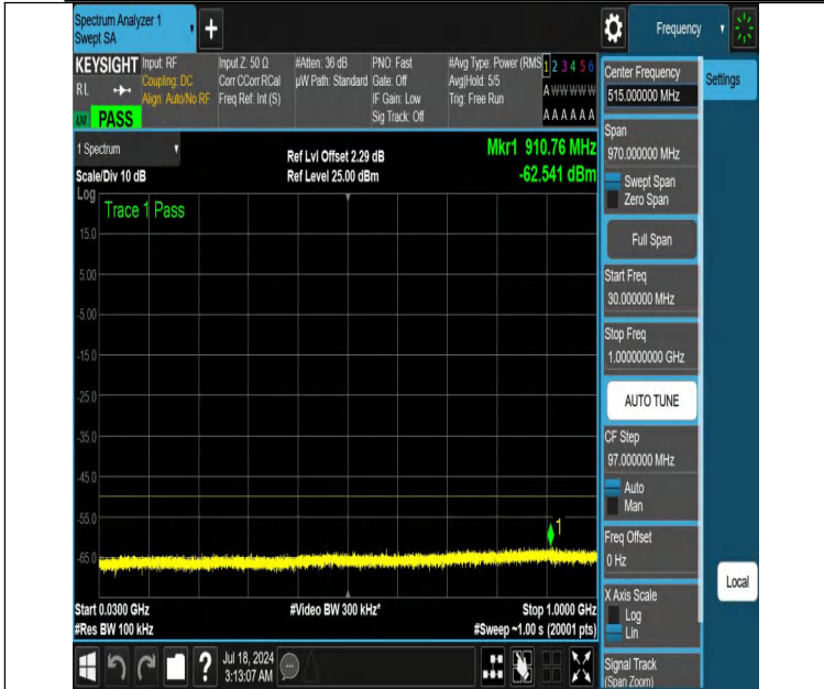
NTNV-DC_13A_n48A-PC3-30-5+10-M+M-N/A-N/A-DFT-QPSK-Edge_1RB_Left-30-1000-PASS
