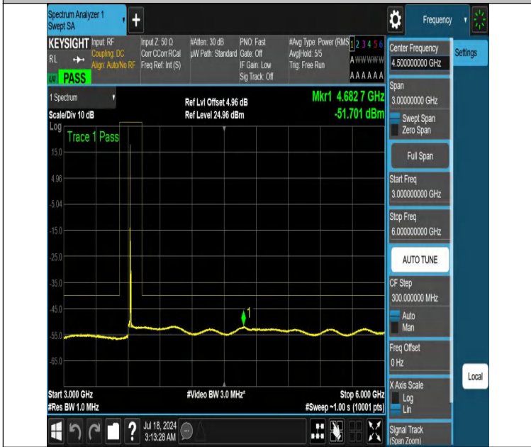
NTNV-DC_13A_n48A-PC3-30-5+10-M+M-N/A-N/A-DFT-QPSK-Edge_1RB_Left-3000-6000-PASS
