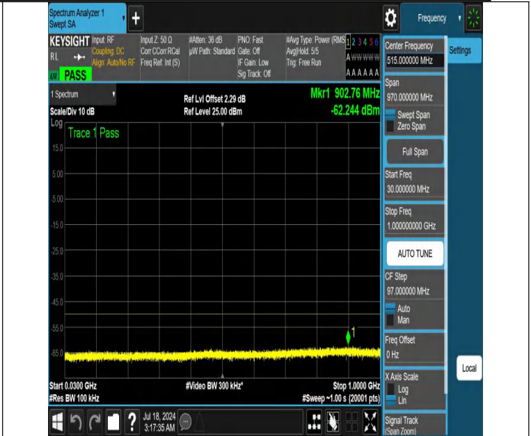
NTNV-DC_13A_n48A-PC3-30-5+10-M+H-N/A-N/A-DFT-PI2BPSK-E dge_1RB_Right-30-1000-PASS
