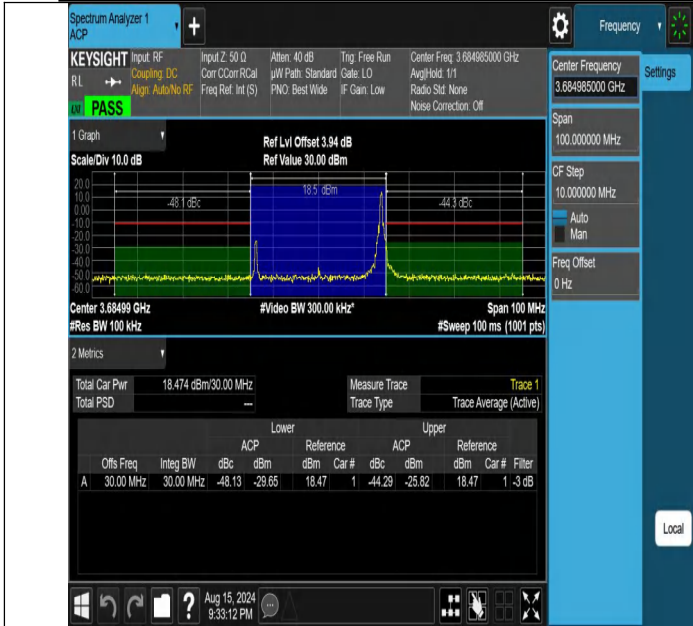
NTNV-DC_13A_n48A-PC3-30-5+30-M+H-N/A-N/A-CP-QPSK-Edge _1RB_Right-PASS
