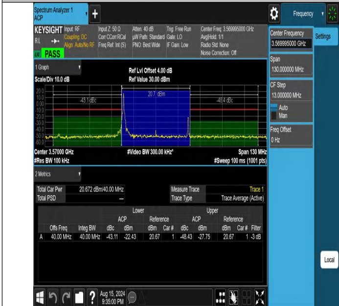
NTNV-DC_13A_n48A-PC3-30-5+40-M+L-N/A-N/A-DFT-PI2BPSK-Edge_1RB_Left-PASS
