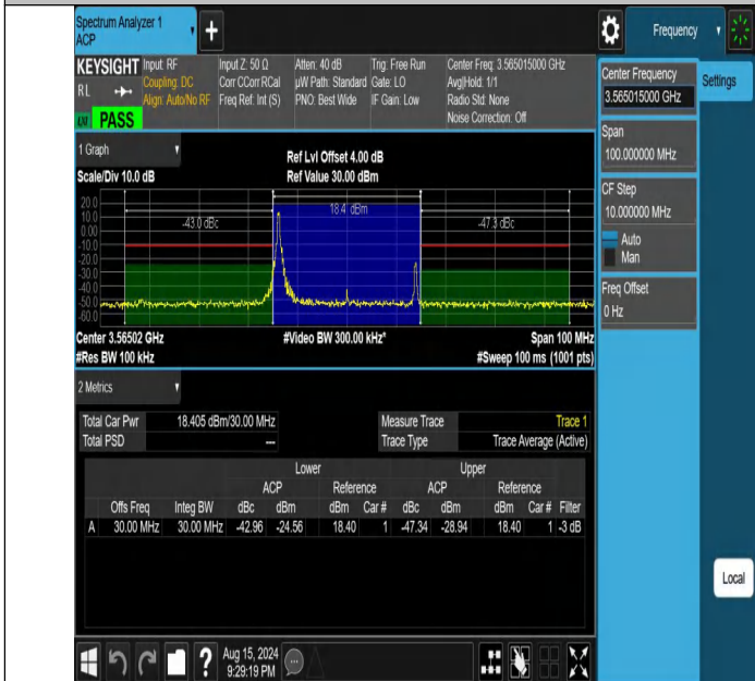
NTNV-DC_13A_n48A-PC3-30-5+30-M+L-N/A-N/A-CP-QPSK-Edge _1RB_Left-PASS
