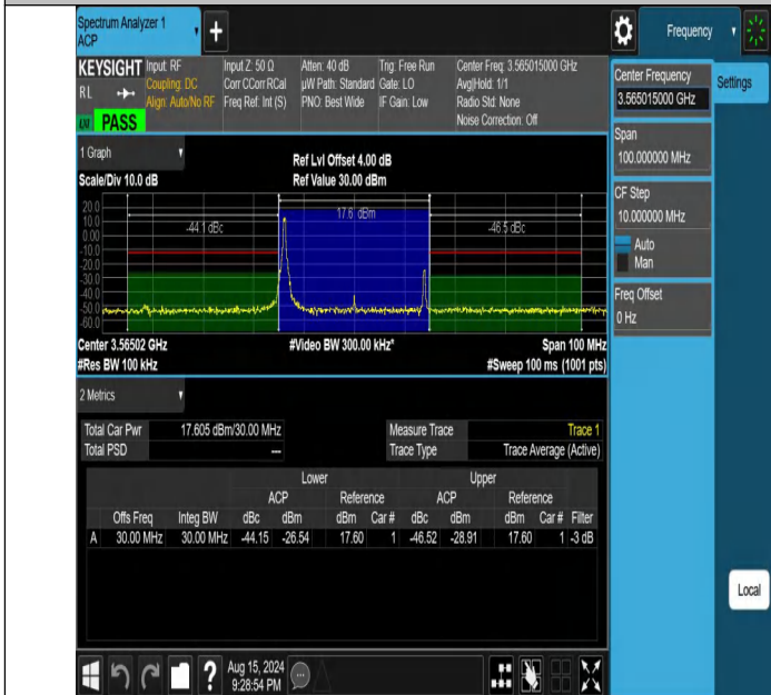
NTNV-DC_13A_n48A-PC3-30-5+30-M+L-N/A-N/A-DFT-256QAM-E dge_1RB_Left-PASS
