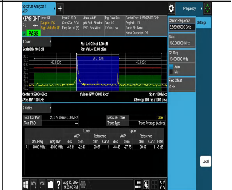
NTNV-DC_13A_n48A-PC3-30-5+40-M+L-N/A-N/A-DFT-PI2BPSK-Edge_1RB_Left-PASS
