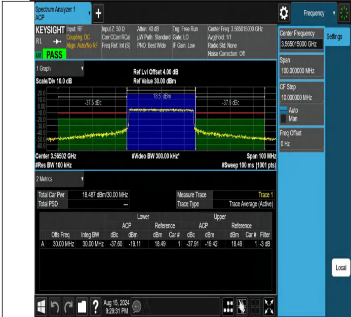
NTNV-DC_13A_n48A-PC3-30-5+30-M+L-N/A-N/A-CP-QPSK-Outer _Full-PASS
