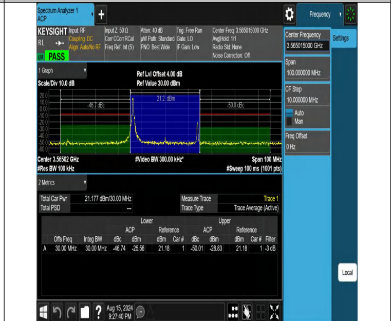
NTVN-DC_13A_n48A-PC3-30-5+30-M+L-N/A-N/A-DFT-QPSK-Edg e_1RB_Left-PASS
