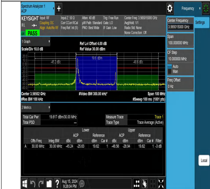
NTVN-DC_13A_n48A-PC3-30-5+30-M+L-N/A-N/A-DFT-16QAM-Ed ge_1RB_Left-PASS
