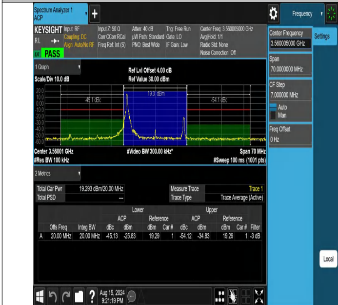
NTNV-DC_13A_n48A-PC3-30-5+20-M+L-N/A-N/A-CP-QPSK-Edge _1RB_Left-PASS
