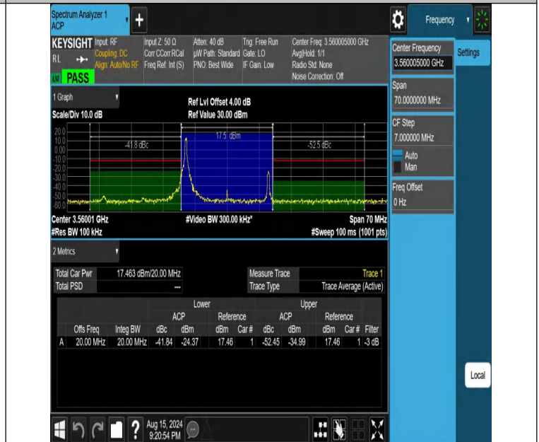
NTNV-DC_13A_n48A-PC3-30-5+20-M+L-N/A-N/A-DFT-256QAM-E dge_1RB_Left-PASS
