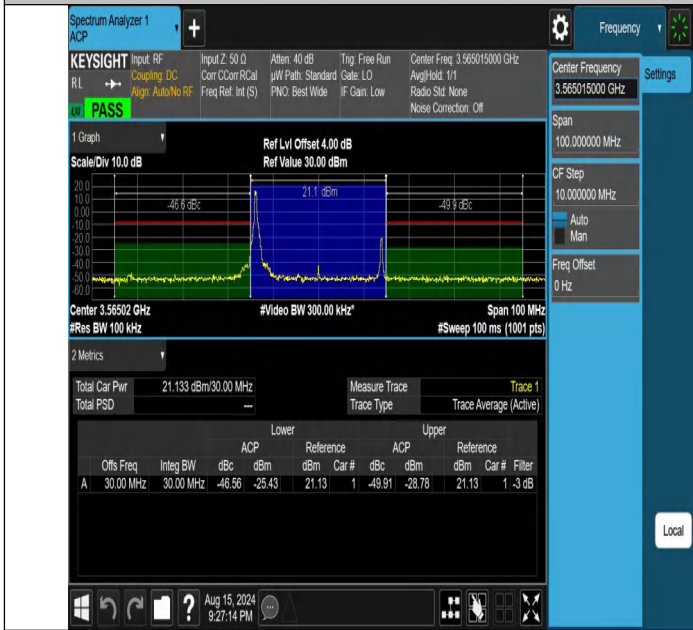
NTNV-DC_13A_n48A-PC3-30-5+30-M+L-N/A-N/A-DFT-PI2BPSK-E_dge_1RB_Left-PASS
