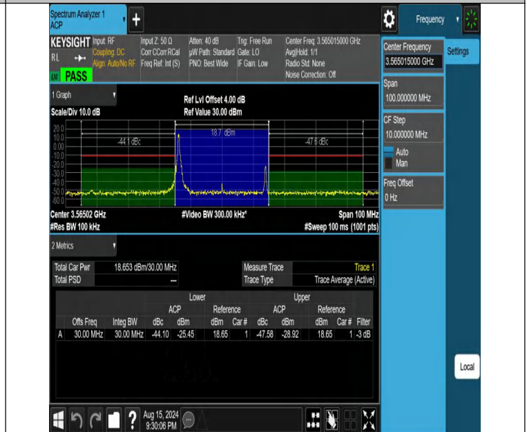
NTNV-DC_13A_n48A-PC3-30-5+30-M+L-N/A-N/A-CP-64QAM-Edge_1RB_Left-PASS
