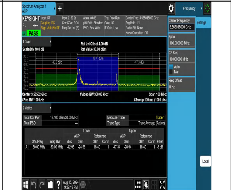
NTNV-DC_13A_n48A-PC3-30-5+30-M+L-N/A-N/A-CP-QPSK-Edge _1RB_Left-PASS
