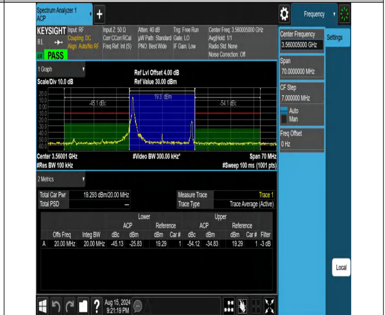
NTNV-DC_13A_n48A-PC3-30-5+20-M+L-N/A-N/A-CP-QPSK-Edge _1RB_Left-PASS
