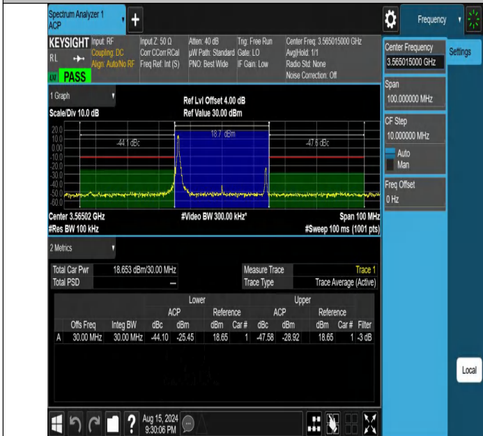
NTNV-DC_13A_n48A-PC3-30-5+30-M+L-N/A-N/A-CP-64QAM-Edge_1RB_Left-PASS
