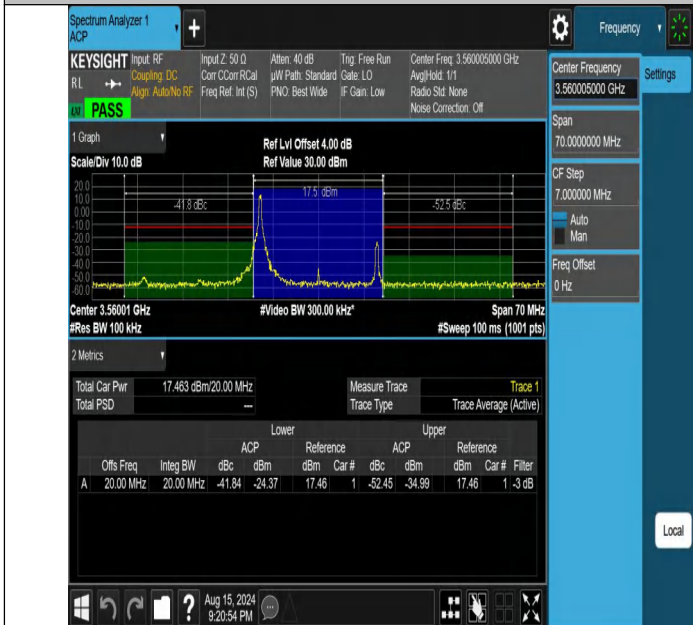
NTNV-DC_13A_n48A-PC3-30-5+20-M+L-N/A-N/A-DFT-256QAM-E dge_1RB_Left-PASS
