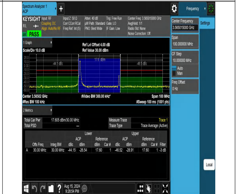
NTNV-DC_13A_n48A-PC3-30-5+30-M+L-N/A-N/A-DFT-256QAM-E dge_1RB_Left-PASS
