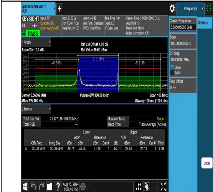
NTVN-DC_13A_n48A-PC3-30-5+30-M+L-N/A-N/A-DFT-QPSK-Edg e_1RB_Left-PASS
