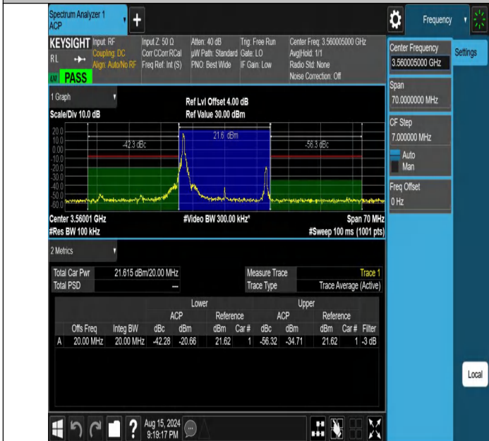
NTNV-DC_13A_n48A-PC3-30-5+20-M+L-N/A-N/A-DFT-PI2BPSK-Edge_1RB_Left-PASS
