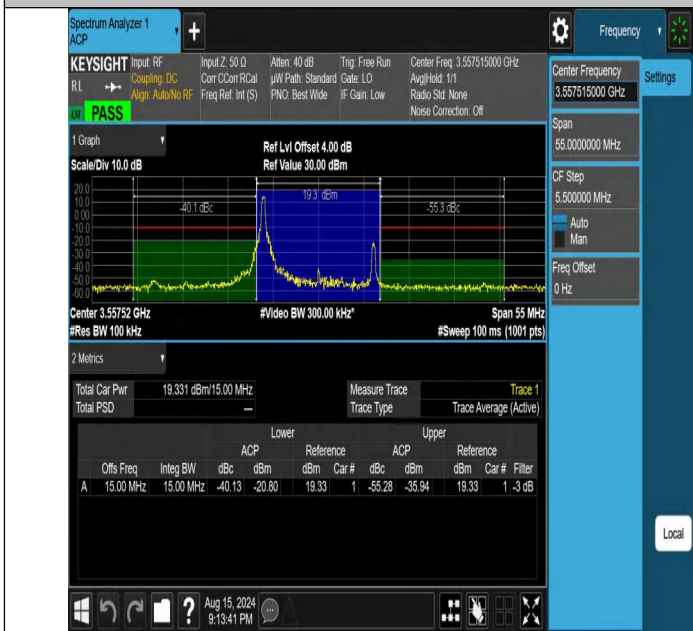
NTNV-DC_13A_n48A-PC3-30-5+15-M+L-N/A-N/A-CP-QPSK-Edge_1RB_Left-PASS
