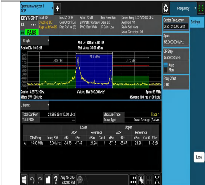
NTNV-DC_13A_n48A-PC3-30-5+15-M+L-N/A-N/A-DFT-QPSK-Edg e_1RB_Left-PASS
