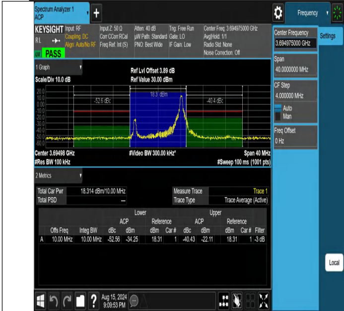
NTNV-DC_13A_n48A-PC3-30-5+10-M+H-N/A-N/A-CP-QPSK-Edge _1RB_Right-PASS
