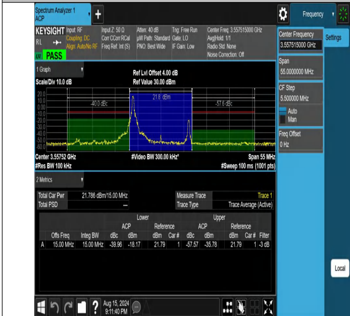
NTNV-DC_13A_n48A-PC3-30-5+15-M+L-N/A-N/A-DFT-PI2BPSK-E_dge_1RB_Left-PASS
