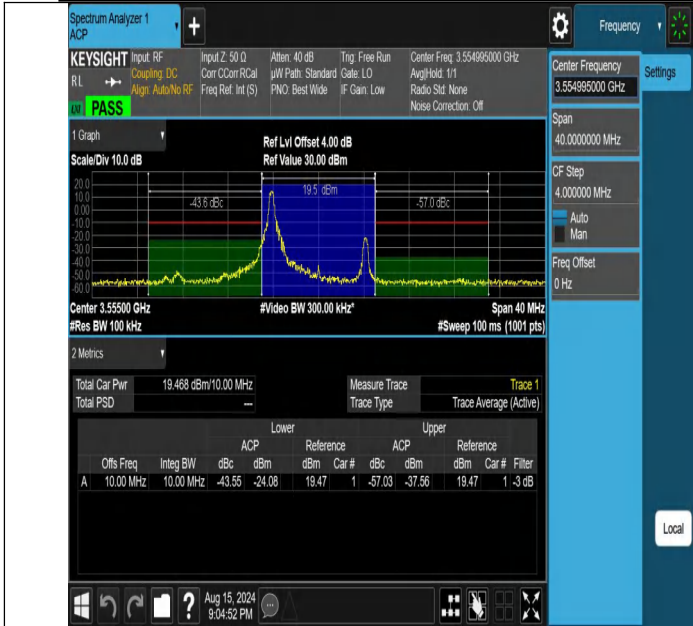
NTNV-DC_13A_n48A-PC3-30-5+10-M+L-N/A-N/A-DFT-16QAM-Edge_1RB_Left-PASS
