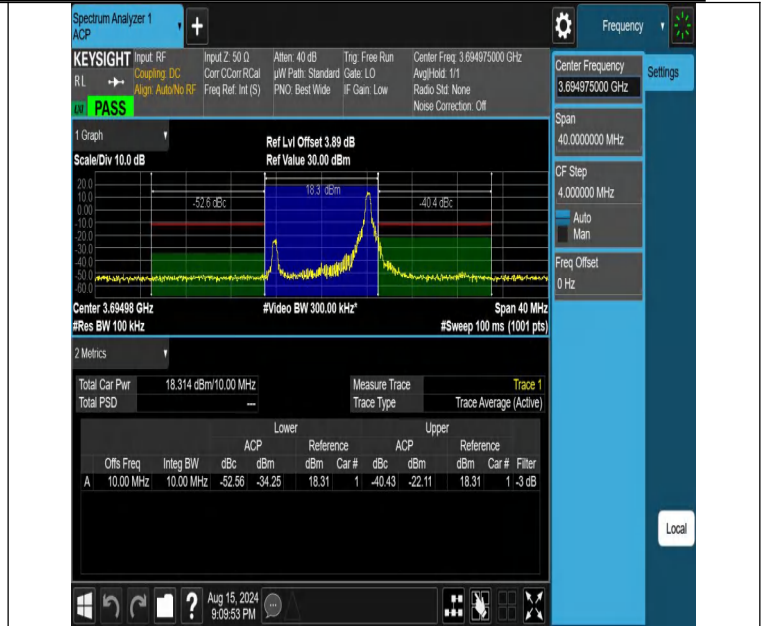
NTNV-DC_13A_n48A-PC3-30-5+10-M+H-N/A-N/A-CP-QPSK-Edge _1RB_Right-PASS
