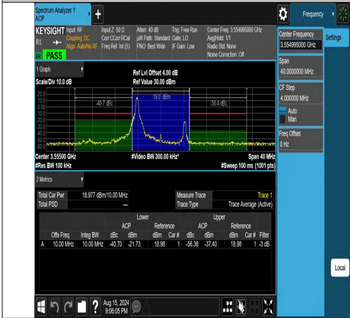
NTVN-DC_13A_n48A-PC3-30-5+10-M+L-N/A-N/A-CP-QPSK-Edge _1RB_Left-PASS
