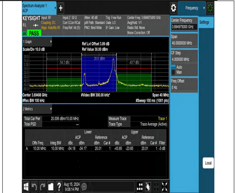
NTNV-DC_13A_n48A-PC3-30-5+10-M+H-N/A-N/A-DFT-QPSK-Edge_1RB_Right-PASS
