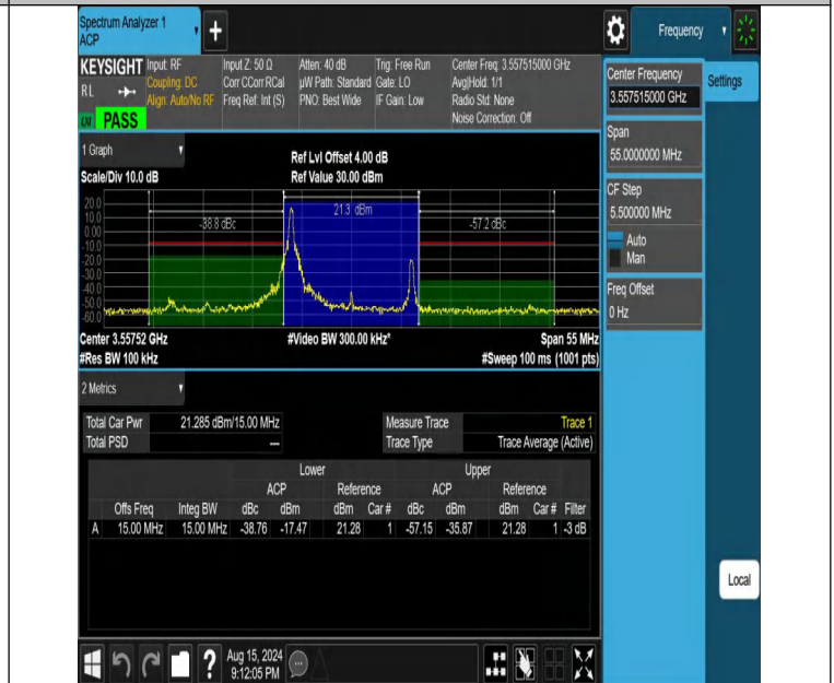
NTNV-DC_13A_n48A-PC3-30-5+15-M+L-N/A-N/A-DFT-QPSK-Edg e_1RB_Left-PASS
