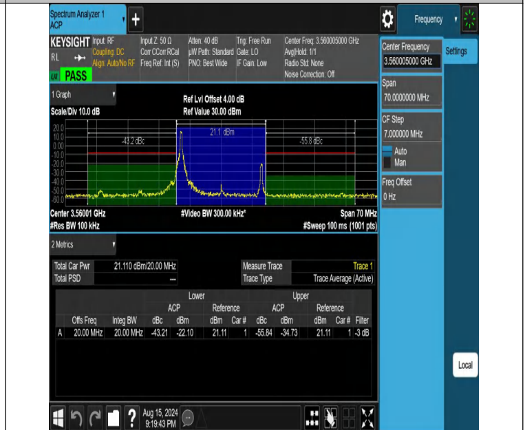
NTNV-DC_13A_n48A-PC3-30-5+20-M+L-N/A-N/A-DFT-QPSK-Edg e_1RB_Left-PASS
