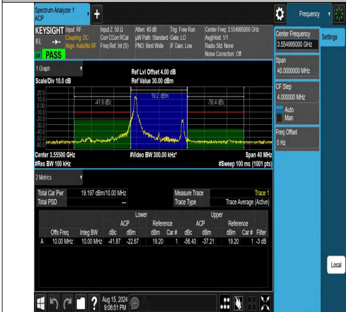
NTNV-DC_13A_n48A-PC3-30-5+10-M+L-N/A-N/A-CP-64QAM-Edge_1RB_Left-PASS
