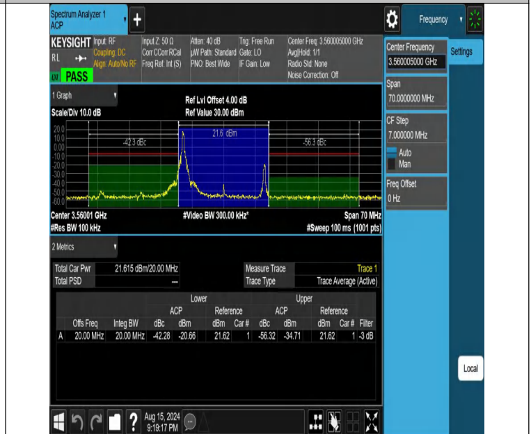
NTNV-DC_13A_n48A-PC3-30-5+20-M+L-N/A-N/A-DFT-PI2BPSK-Edge_1RB_Left-PASS
