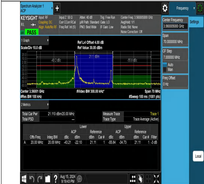
NTNV-DC_13A_n48A-PC3-30-5+20-M+L-N/A-N/A-DFT-QPSK-Edg e_1RB_Left-PASS
