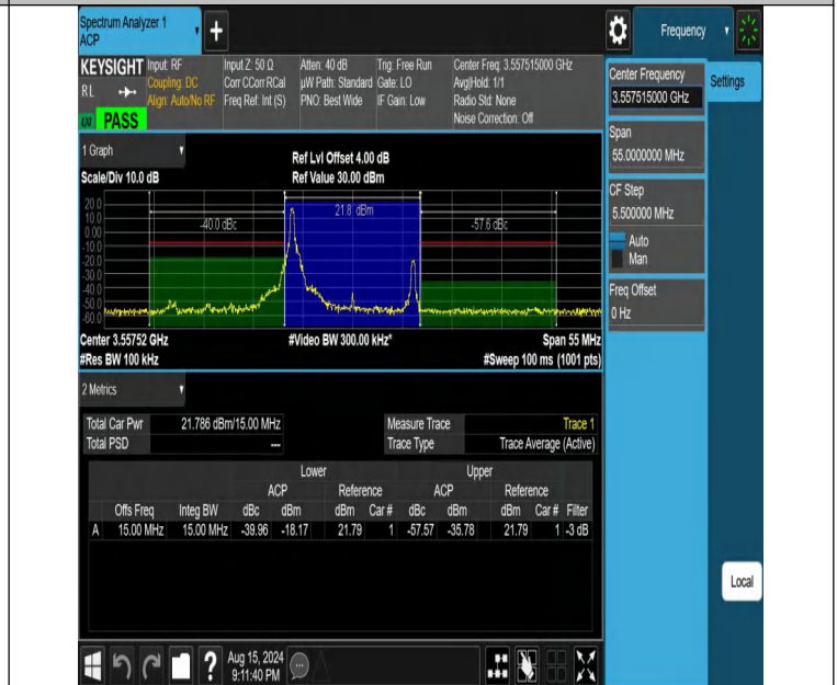
NTNV-DC_13A_n48A-PC3-30-5+15-M+L-N/A-N/A-DFT-PI2BPSK-E_dge_1RB_Left-PASS
