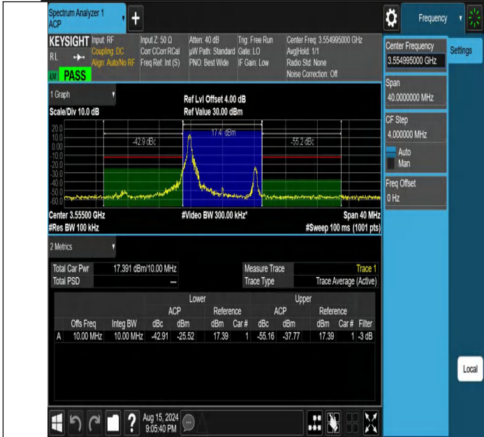
NTVN-DC_13A_n48A-PC3-30-5+10-M+L-N/A-N/A-DFT-256QAM-E dge_1RB_Left-PASS
