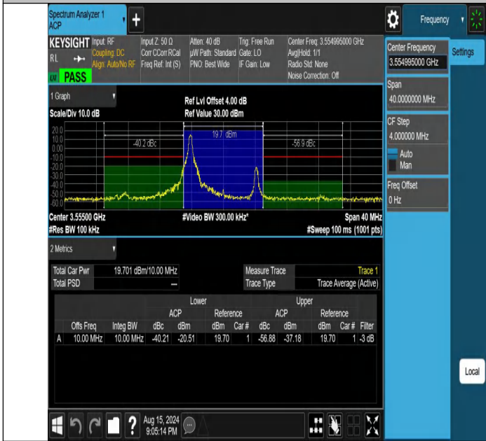
NTNV-DC_13A_n48A-PC3-30-5+10-M+L-N/A-N/A-DFT-64QAM-Edge_1RB_Left-PASS
