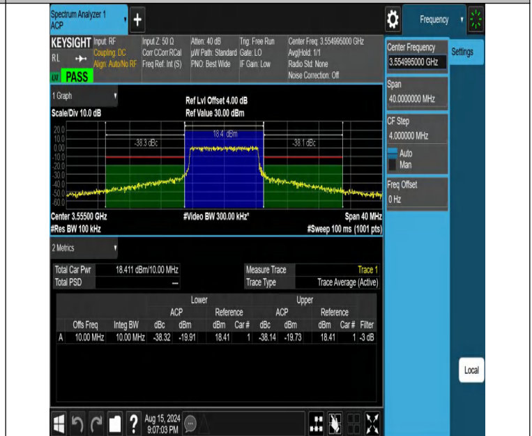
NTNV-DC_13A_n48A-PC3-30-5+10-M+L-N/A-N/A-CP-64QAM-Out_Full-PASS
