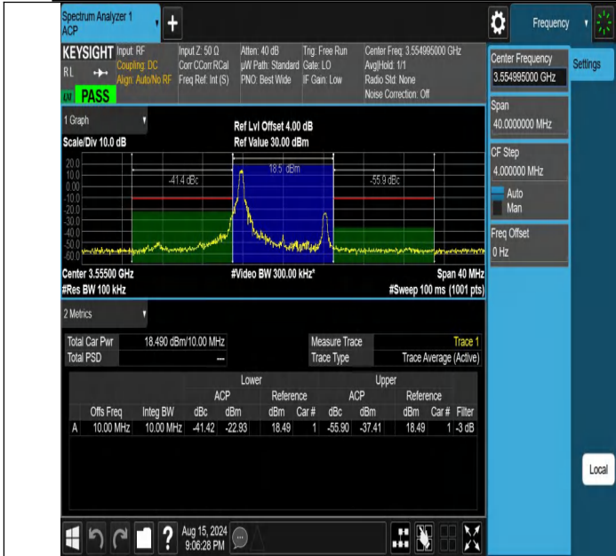
NTNV-DC_13A_n48A-PC3-30-5+10-M+L-N/A-N/A-CP-16QAM-Edge_1RB_Left-PASS
