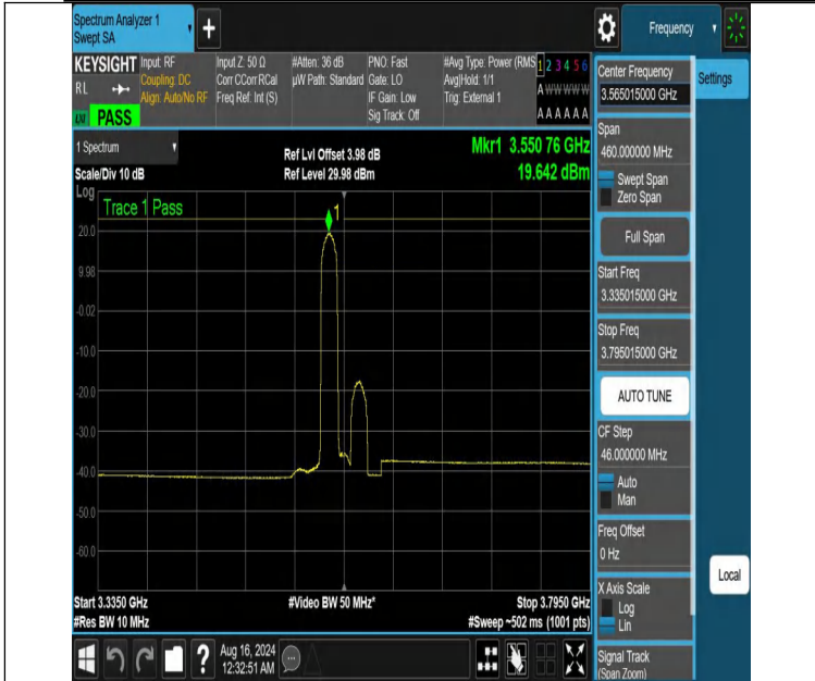
NTNV-DC_13A_n48A-PC3-30-5+30-M+L-N/A-N/A-CP-QPSK-Edge _1RB_Left-3335.015-3795.015-PASS
