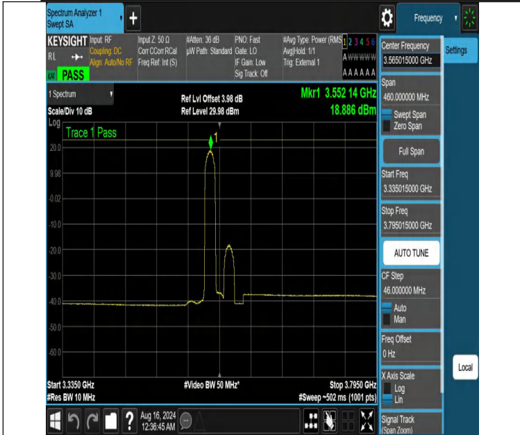
NTVN-DC_13A_n48A-PC3-30-5+30-M+L-N/A-N/A-CP-64QAM-Edge_1RB_Left-3335.015-3795.015-PASS
