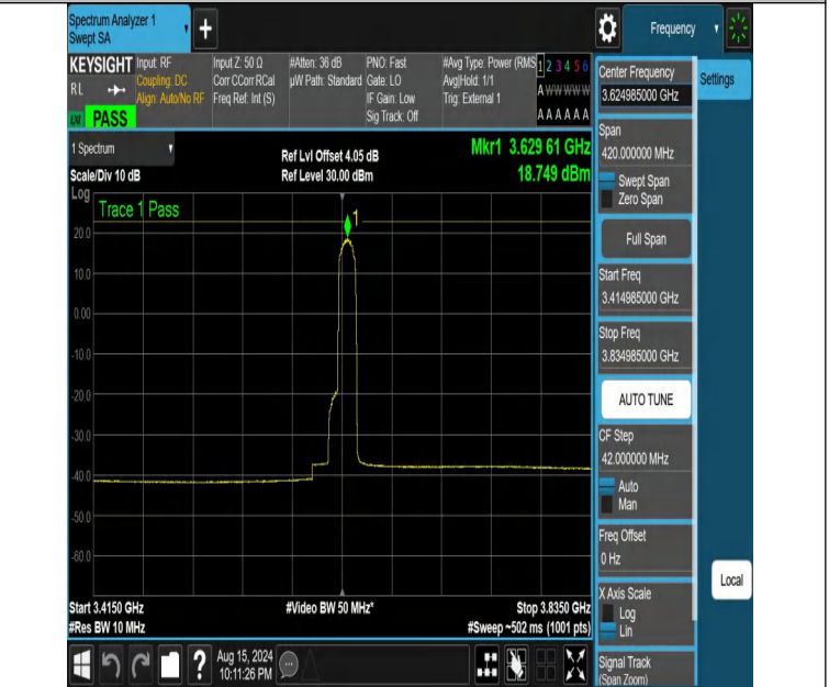
NTVN-DC_13A_n48A-PC3-30-5+10-M+M-N/A-N/A-CP-QPSK-Edge_1RB_Right-3414.985-3834.985-PASS
