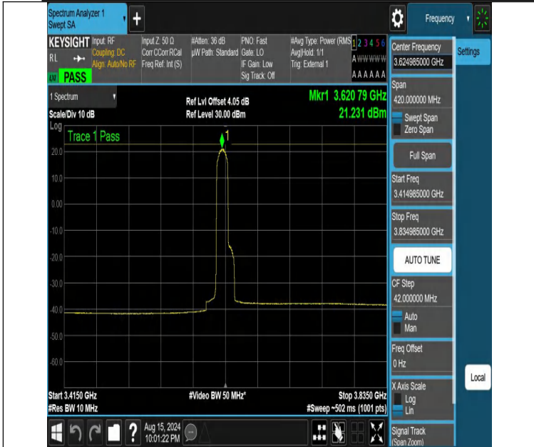
NTNV-DC_13A_n48A-PC3-30-5+10-M+M-N/A-N/A-DFT-PI2BPSK-Edge_1RB_Left-3414.985-3834.985-PASS
