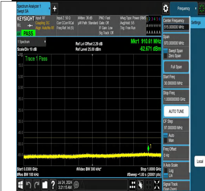
NTNV-N48-PC3-30-30-H-DFT-QPSK-Edge_1RB_Left-30-1000-A nt1-PASS
