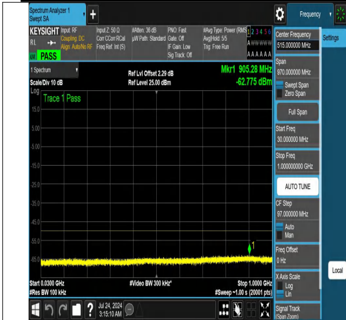
NTNV-N48-PC3-30-30-M-DFT-QPSK-Edge_1RB_Left-30-1000-A nt1-PASS
