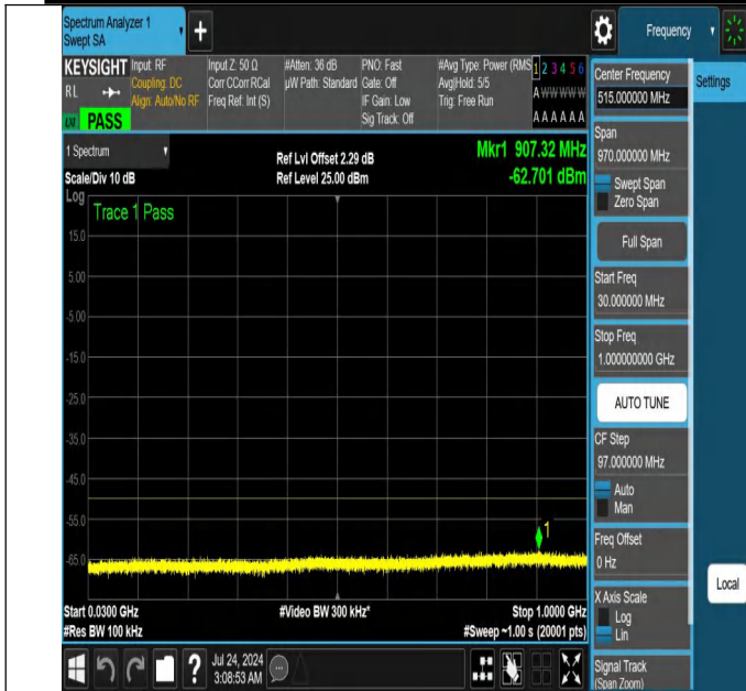
NTNV-N48-PC3-30-30-L-DFT-QPSK-Edge_1RB_Left-30-1000-A nt1-PASS
