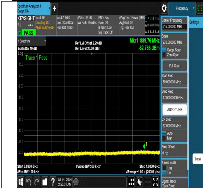
NTNV-N48-PC3-30-20-M-DFT-QPSK-Edge_1RB_Left-30-1000-A nt1-PASS
