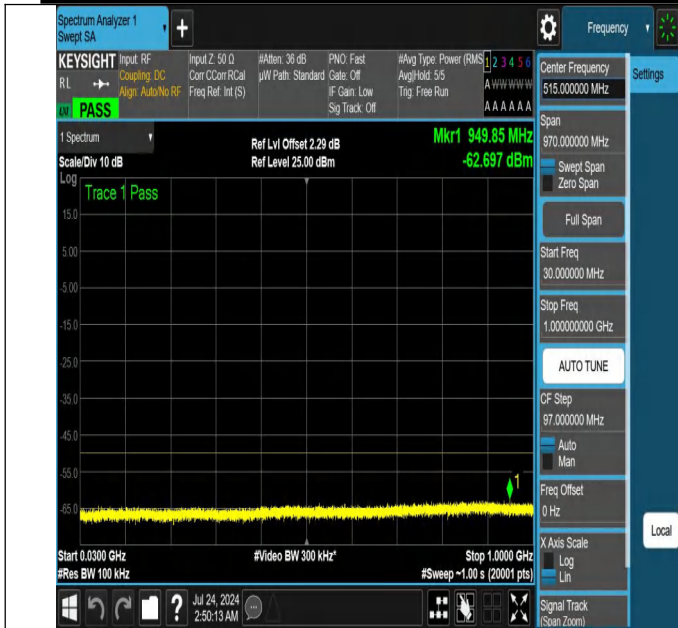
NTNV-N48-PC3-30-20-L-DFT-QPSK-Edge_1RB_Left-30-1000-A nt1-PASS
