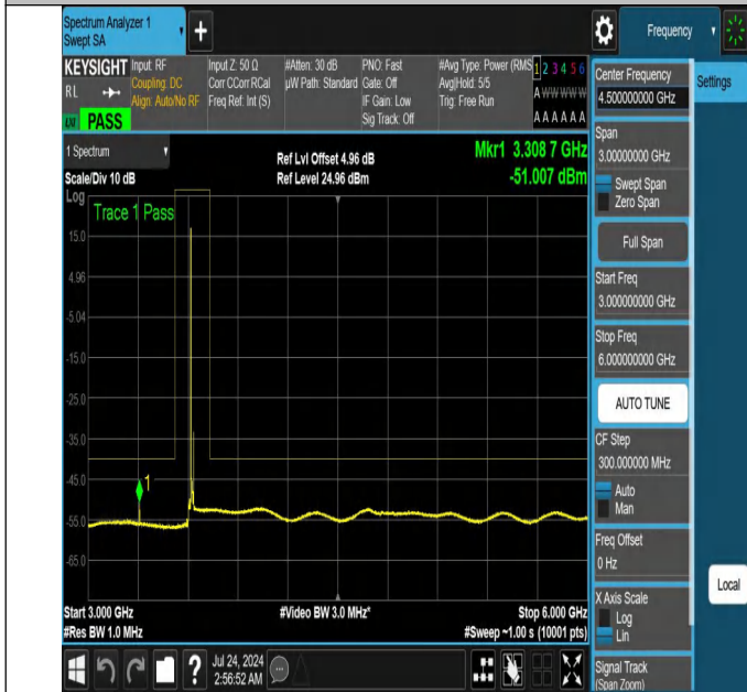
NTNV-N48-PC3-30-20-M-DFT-QPSK-Edge_1RB_Left-3000-6000-A -Ant1-PASS
