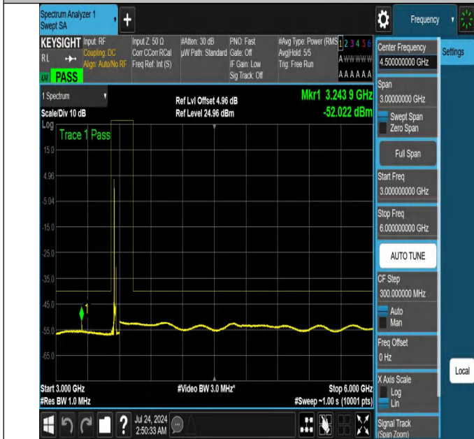
NTNV-N48-PC3-30-20-L-DFT-QPSK-Edge_1RB_Left-3000-6000-Ant1-PASS
