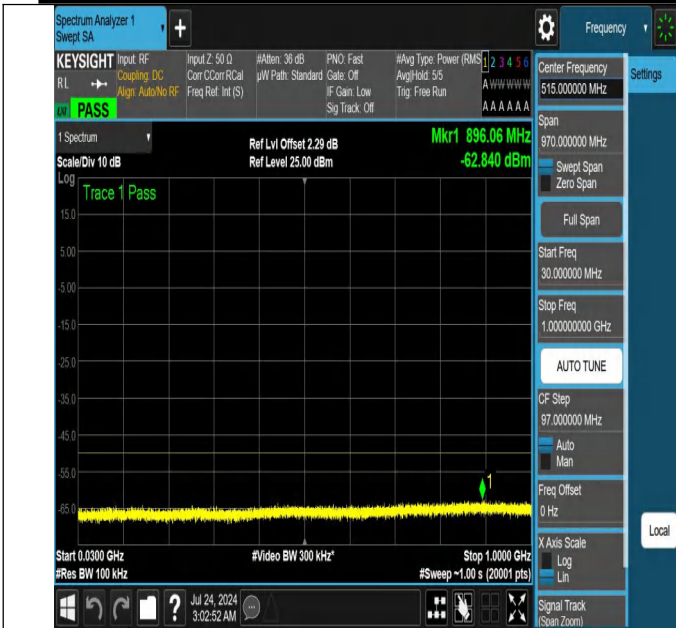
NTNV-N48-PC3-30-20-H-DFT-QPSK-Edge_1RB_Left-30-1000-A nt1-PASS
