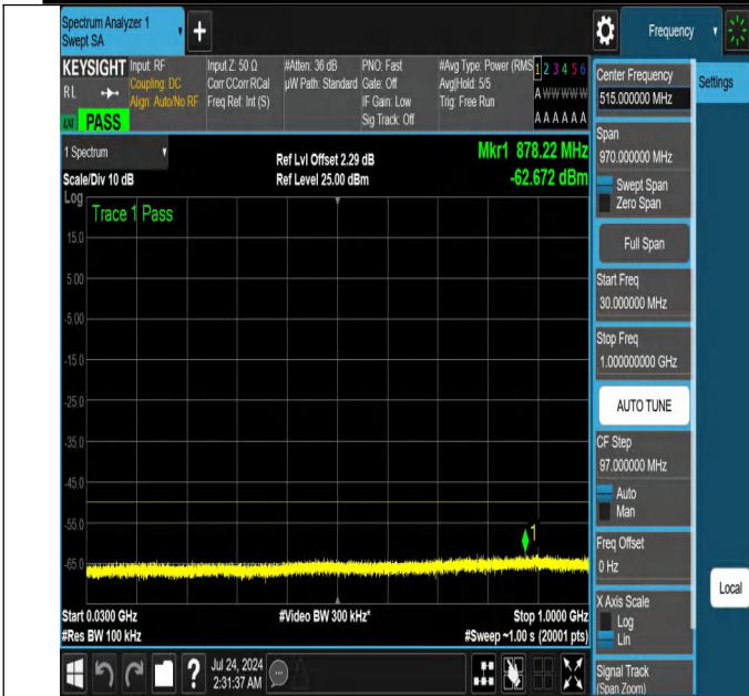
NTNV-N48-PC3-30-15-L-DFT-QPSK-Edge_1RB_Left-30-1000-A nt1-PASS
