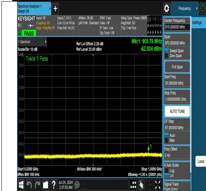
NTNV-N48-PC3-30-15-M-DFT-QPSK-Edge_1RB_Left-30-1000-A nt1-PASS
