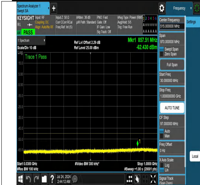
NTNV-N48-PC3-30-15-H-DFT-QPSK-Edge_1RB_Left-30-1000-A nt1-PASS
