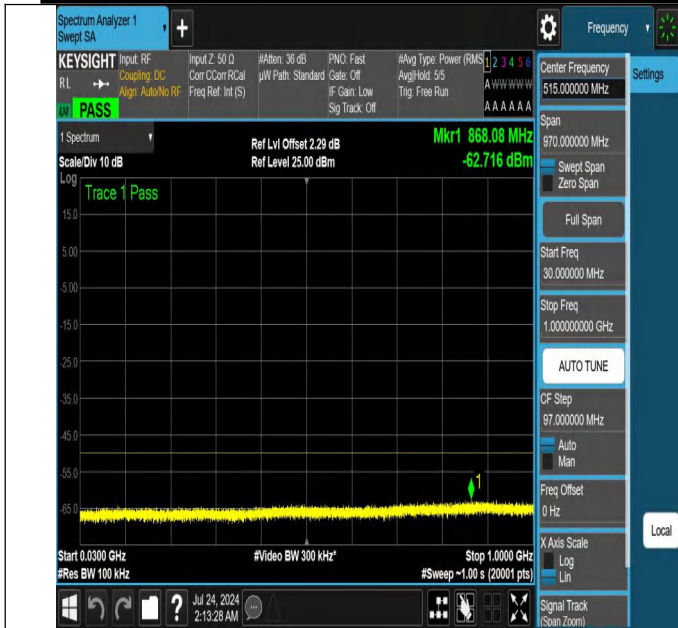
NTNV-N48-PC3-30-10-L-DFT-QPSK-Edge_1RB_Left-30-1000-A nt1-PASS
