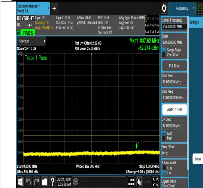
NTNV-N48-PC3-30-10-H-DFT-QPSK-Edge_1RB_Left-30-1000-A nt1-PASS
