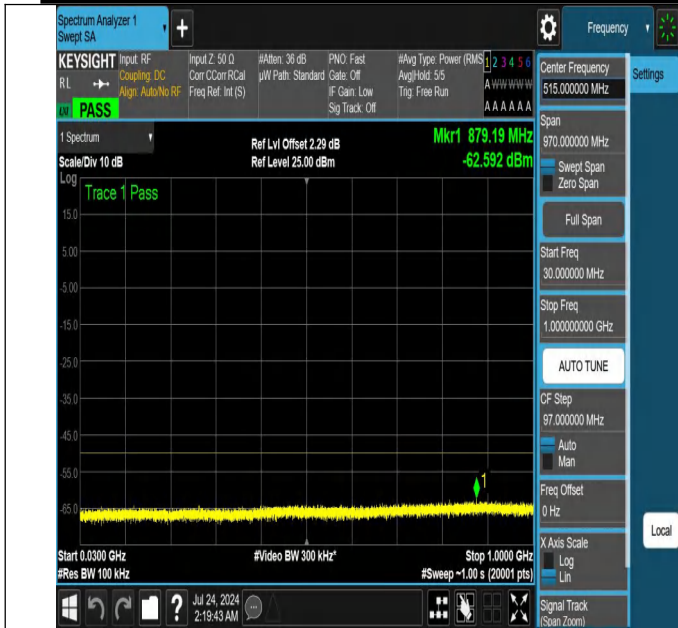
NTNV-N48-PC3-30-10-M-DFT-QPSK-Edge_1RB_Left-30-1000-A nt1-PASS
