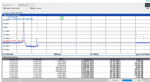
NTVN-n48-PC3-30-20-L-DFT-QPSK-Edge_1RB_Left-PASS
