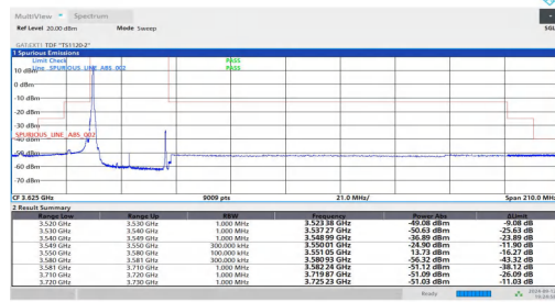
NTVN-n48-PC3-30-30-L-DFT-BPSK-Edge_1RB_Left-PASS
