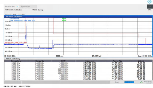
NTNV-n48-PC3-30-40-L-DFT-QPSK-Edge_1RB_Left-PASS
