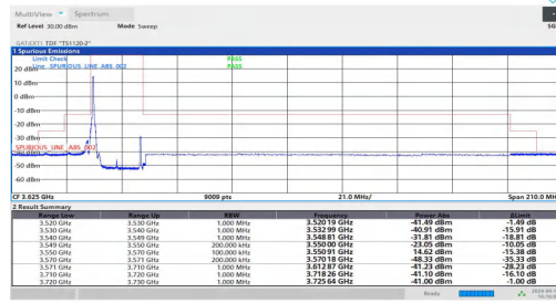
NTVN-n48-PC3-30-20-L-DFT-BPSK-Edge_1RB_Left-PASS
