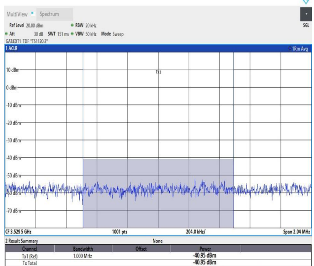
NTVN-n48-PC3-30-30-L-DFT-QPSK-Edge_1RB_Left-PASS
