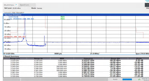
NTVN-n48-PC3-30-30-L-DFT-QPSK-Edge_1RB_Left-PASS
