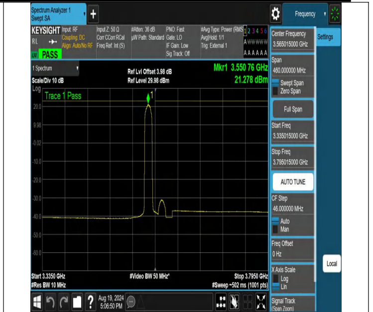
NTNV-N48-PC3-30-30-L-DFT-QPSK-Edge_1RB_Left-3335.015-3795.015-Ant1-PASS
