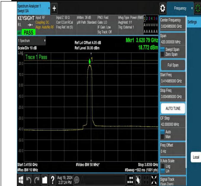
NTNV-N48-PC3-30-10-M-CP-QPSK-Edge_1RB_Left-3414.985-3834.985-Ant1-PASS
