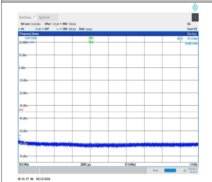
NTNV-n41-PC1.5-30-90-M-CP-QPSK-Edge_1RB_Left-30-1000-P ASS
