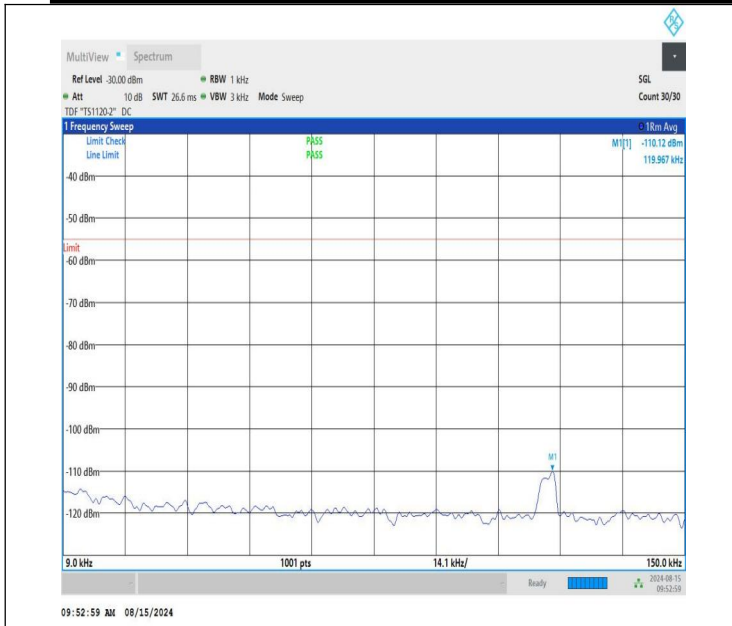
NTNV-n41-PC1.5-30-100-L-CP-QPSK-Edge_1RB_Left-0.009-0.15 -PASS
