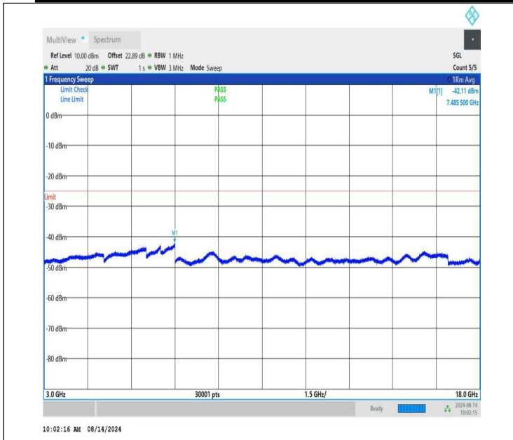
NTNV-n41-PC1.5-30-30-M-CP-QPSK-Edge_1RB_Left-3000-1800 0-PASS
