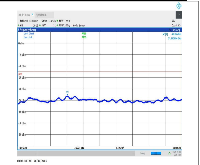
NTVN-n41-PC1.5-30-50-L-CP-QPSK-Edge_1RB_Left-18000-3000 0-PASS
