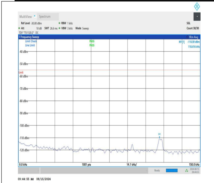
NTNV-n41-PC1.5-30-30-L-CP-QPSK-Edge_1RB_Left-0.009-0.15-PASS
