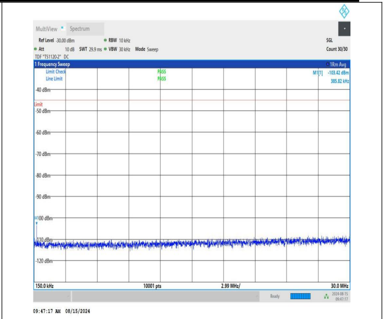
NTNV-n41-PC1.5-30-50-L-CP-QPSK-Edge_1RB_Left-0.15-30-PASS
