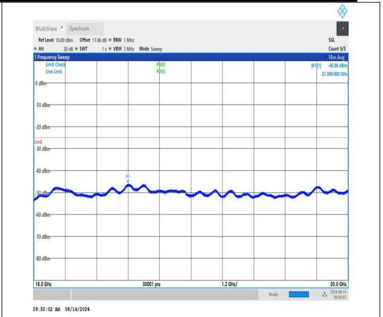
NTNV-n41-PC1.5-30-30-M-CP-QPSK-Edge_1RB_Left-18000-3000 0-PASS
