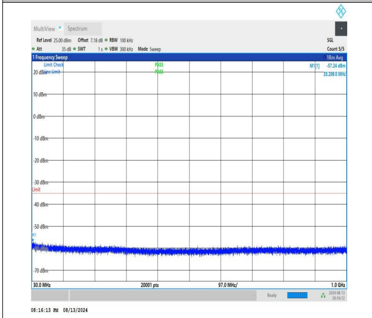
NTNV-n41-PC1.5-30-60-L-CP-QPSK-Edge_1RB_Left-30-1000-PASS
