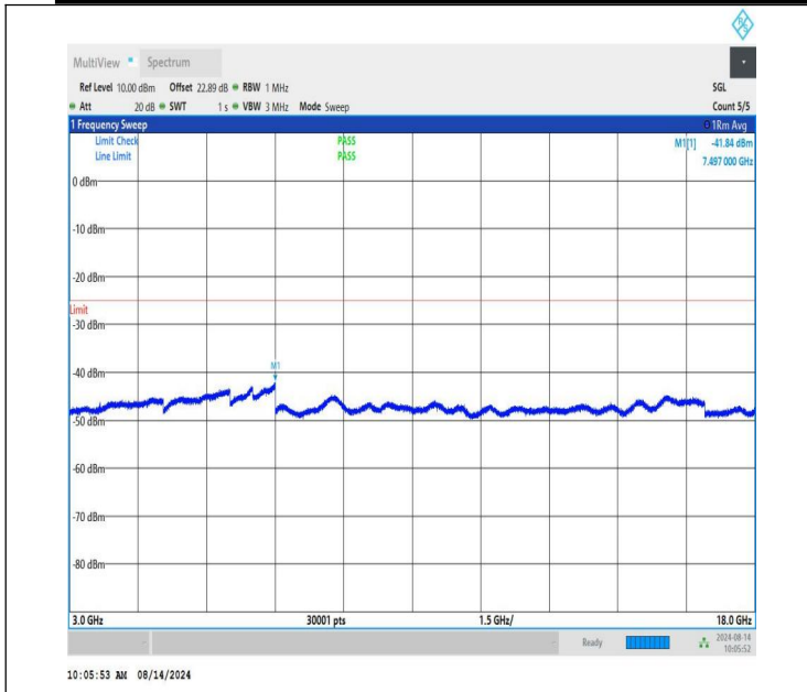
NTVN-n41-PC1.5-30-50-L-CP-QPSK-Edge_1RB_Left-3000-18000 -PASS
