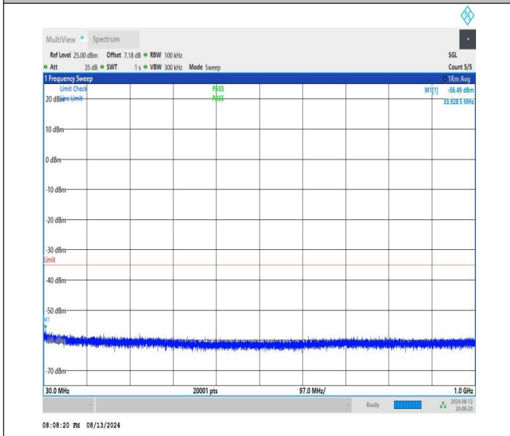
NTNV-n41-PC1.5-30-40-M-CP-QPSK-Edge_1RB_Left-30-1000-P ASS
