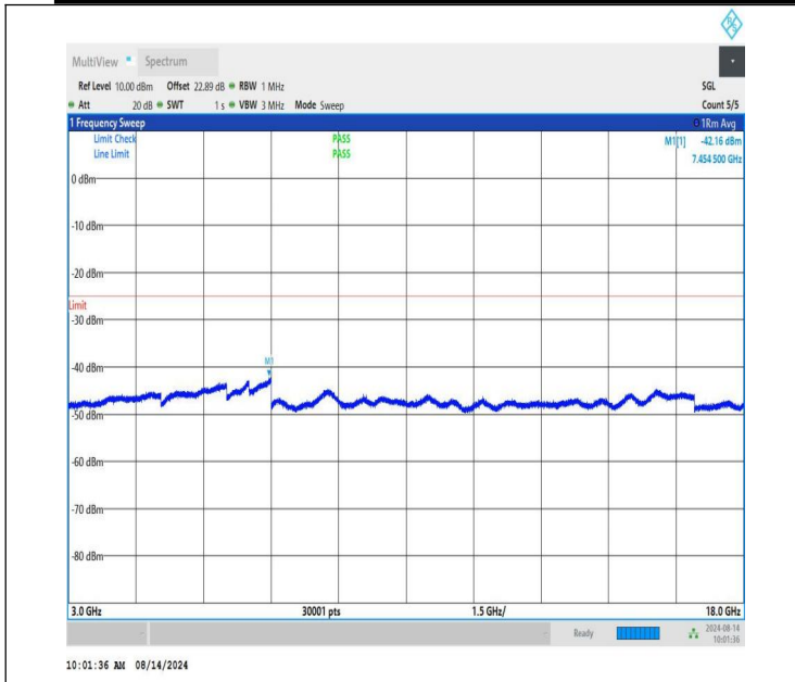
NTVN-n41-PC1.5-30-30-L-CP-QPSK-Edge_1RB_Left-3000-18000 -PASS
