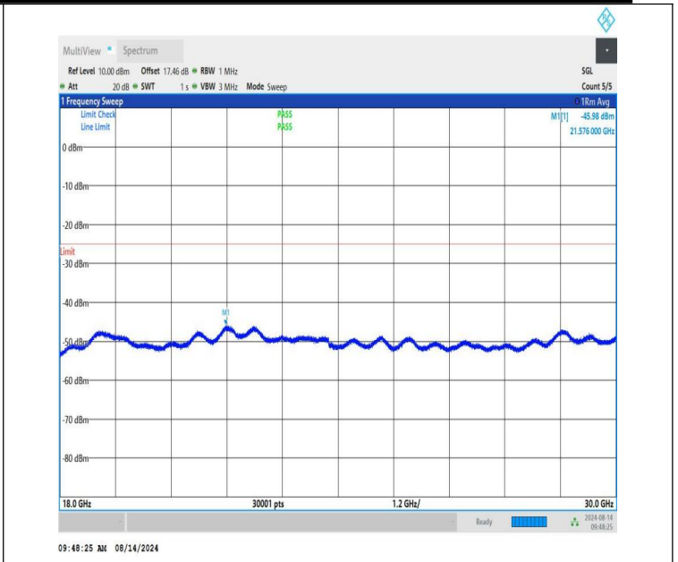
NTVN-n41-PC1.5-30-30-L-CP-QPSK-Edge_1RB_Left-18000-3000 0-PASS
