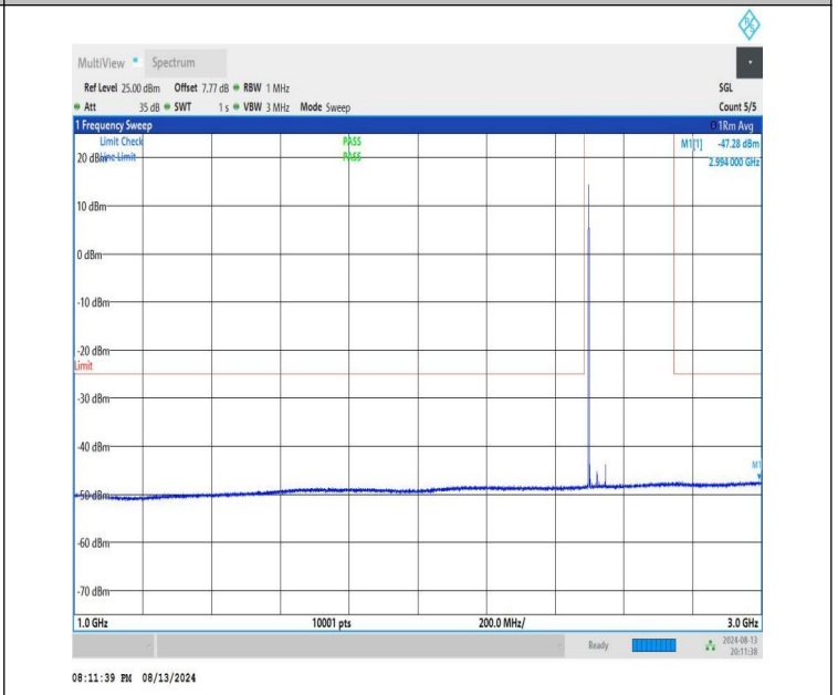
NTNV-n41-PC1.5-30-50-L-CP-QPSK-Edge_1RB_Left-1000-3000-PASS
