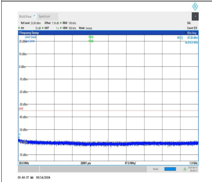
NTNV-n41-PC1.5-30-30-M-CP-QPSK-Edge_1RB_Left-30-1000-P ASS
