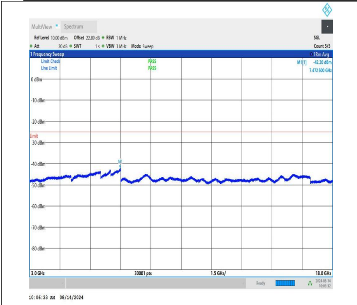
NTNV-n41-PC1.5-30-50-M-CP-QPSK-Edge_1RB_Left-3000-1800 0-PASS
