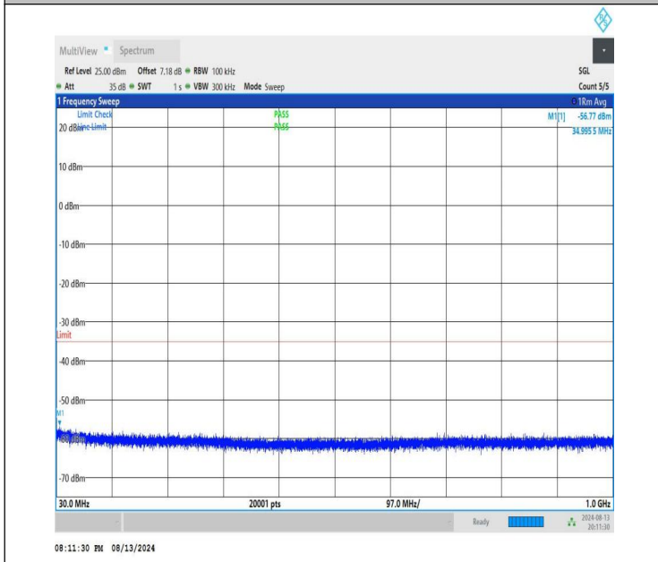
NTNV-n41-PC1.5-30-50-L-CP-QPSK-Edge_1RB_Left-30-1000-PASS
