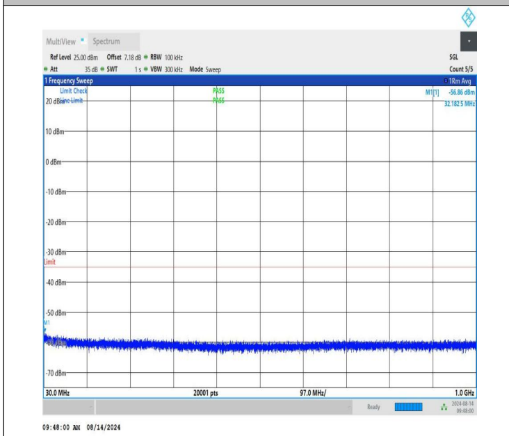
NTNV-n41-PC1.5-30-30-L-CP-QPSK-Edge_1RB_Left-30-1000-PASS
