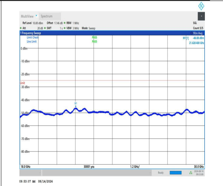
NTVN-n41-PC1.5-30-40-L-CP-QPSK-Edge_1RB_Left-18000-3000 0-PASS
