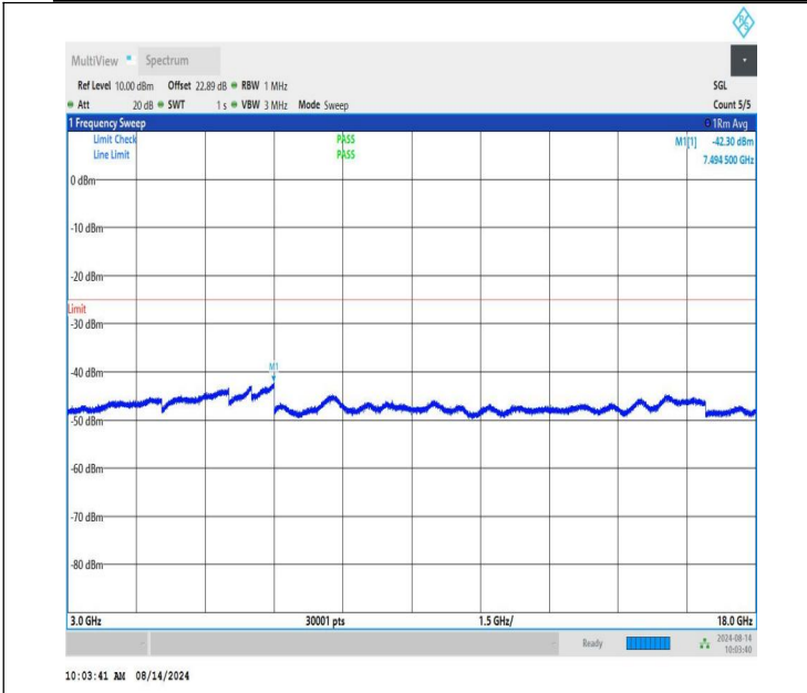
NTVN-n41-PC1.5-30-40-L-CP-QPSK-Edge_1RB_Left-3000-18000 -PASS
