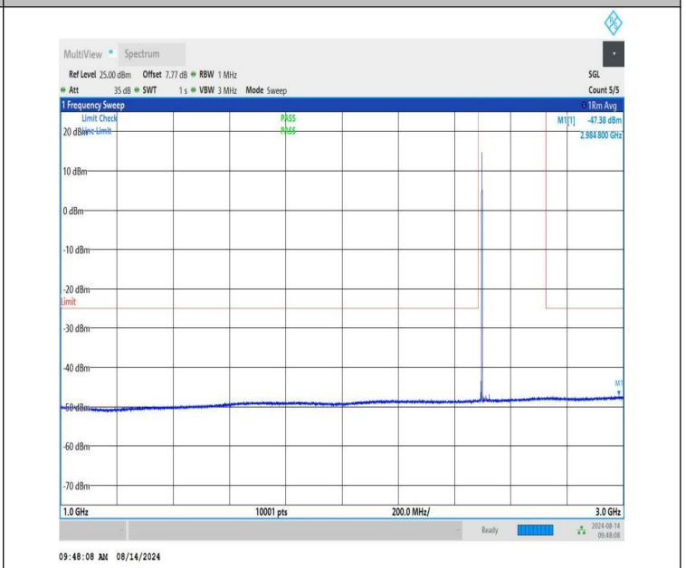
NTNV-n41-PC1.5-30-30-L-CP-QPSK-Edge_1RB_Left-1000-3000-PASS
