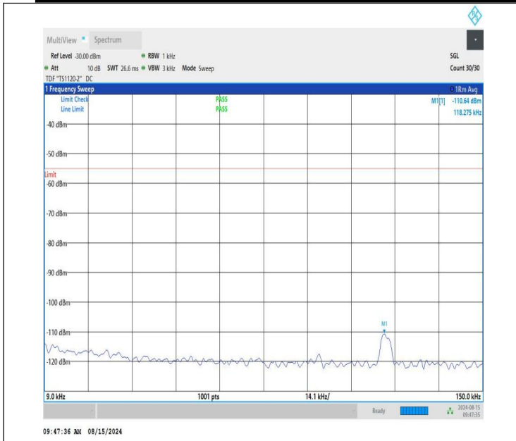
NTNV-n41-PC1.5-30-50-M-CP-QPSK-Edge_1RB_Left-0.009-0.15 -PASS
