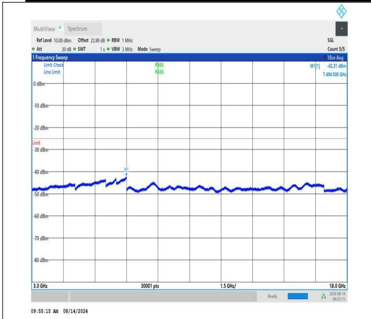
NTVN-n41-PC1.5-30-10-L-CP-QPSK-Edge_1RB_Left-3000-18000 -PASS
