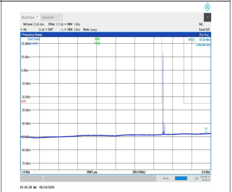
NTNV-n41-PC1.5-30-20-L-CP-QPSK-Edge_1RB_Left-1000-3000-PASS
