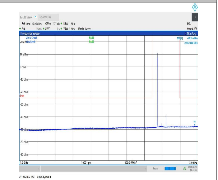
NTNV-n41-PC1.5-30-100-M-CP-QPSK-Edge_1RB_Left-1000-3000 -PASS
