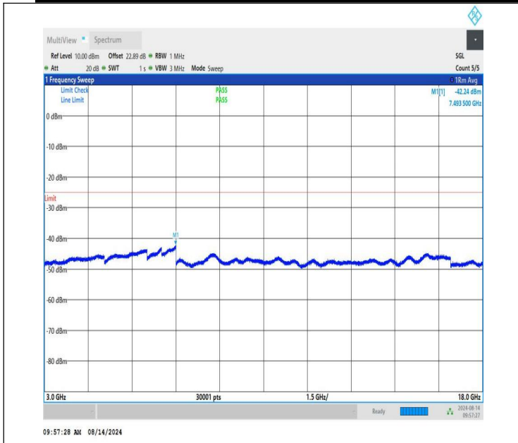
NTVN-n41-PC1.5-30-15-L-CP-QPSK-Edge_1RB_Left-3000-18000 -PASS
