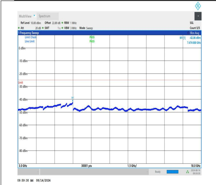
NTVN-n41-PC1.5-30-20-L-CP-QPSK-Edge_1RB_Left-3000-18000 -PASS
