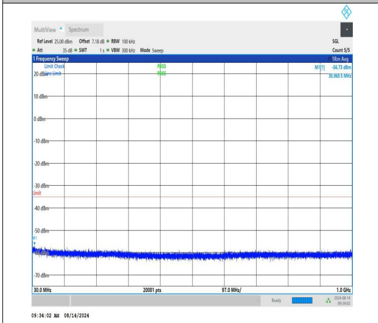
NTNV-n41-PC1.5-30-10-L-CP-QPSK-Edge_1RB_Left-30-1000-PASS
