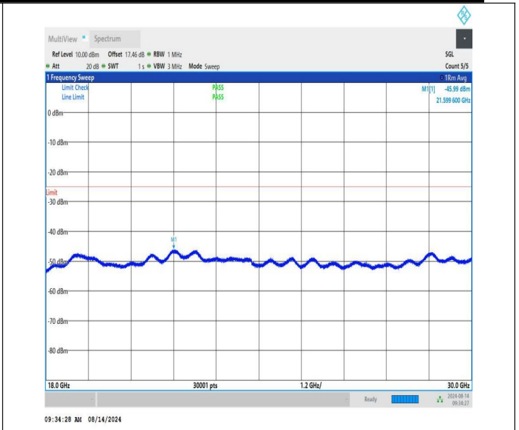
NTVN-n41-PC1.5-30-10-L-CP-QPSK-Edge_1RB_Left-18000-3000 0-PASS
