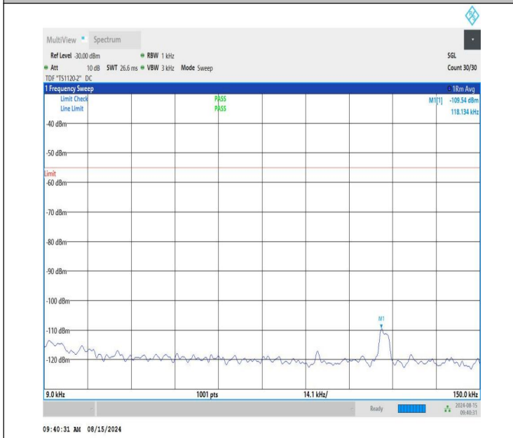
NTVN-n41-PC1.5-30-100-L-CP-QPSK-Edge_1RB_Right-0.009-0. 15-PASS
