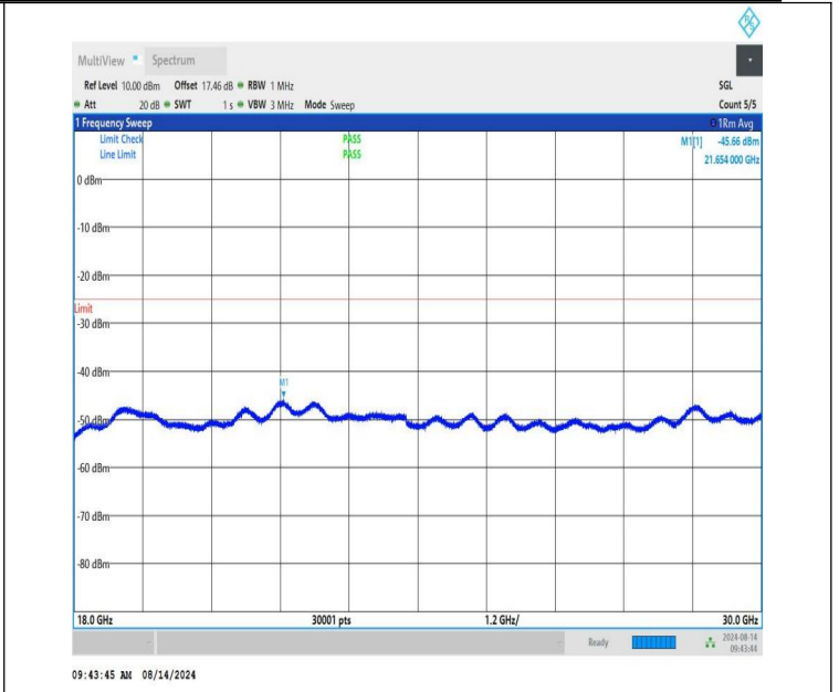
NTVN-n41-PC1.5-30-20-L-CP-QPSK-Edge_1RB_Left-18000-3000 0-PASS
