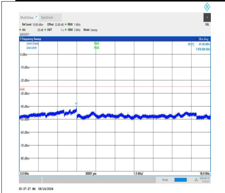
NTVN-n41-PC1.5-30-100-L-CP-QPSK-Edge_1RB_Left-3000-1800 0-PASS
