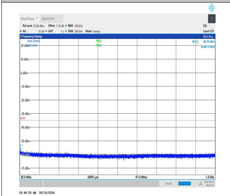
NTNV-n41-PC1.5-30-20-M-CP-QPSK-Edge_1RB_Left-30-1000-P ASS
