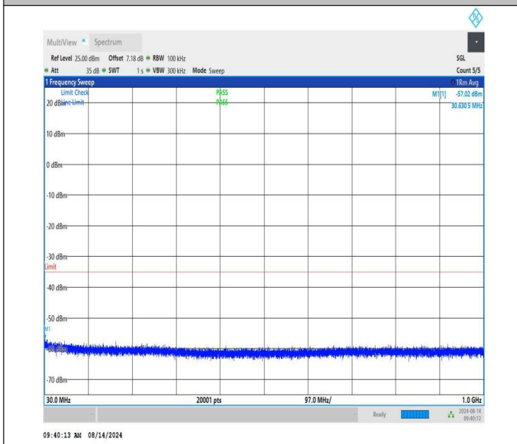
NTNV-n41-PC1.5-30-15-M-CP-QPSK-Edge_1RB_Left-30-1000-P ASS
