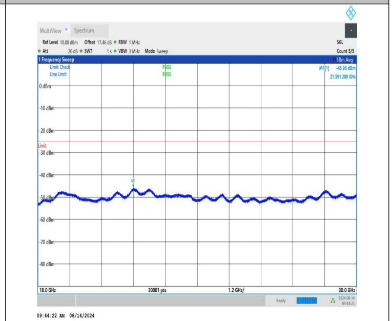
NTNV-n41-PC1.5-30-20-L-CP-QPSK-Edge_1RB_Right-18000-300 00-PASS
