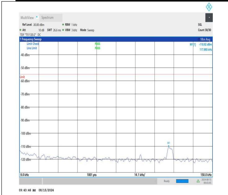
NTNV-n41-PC1.5-30-20-L-CP-QPSK-Edge_1RB_Left-0.009-0.15-PASS
