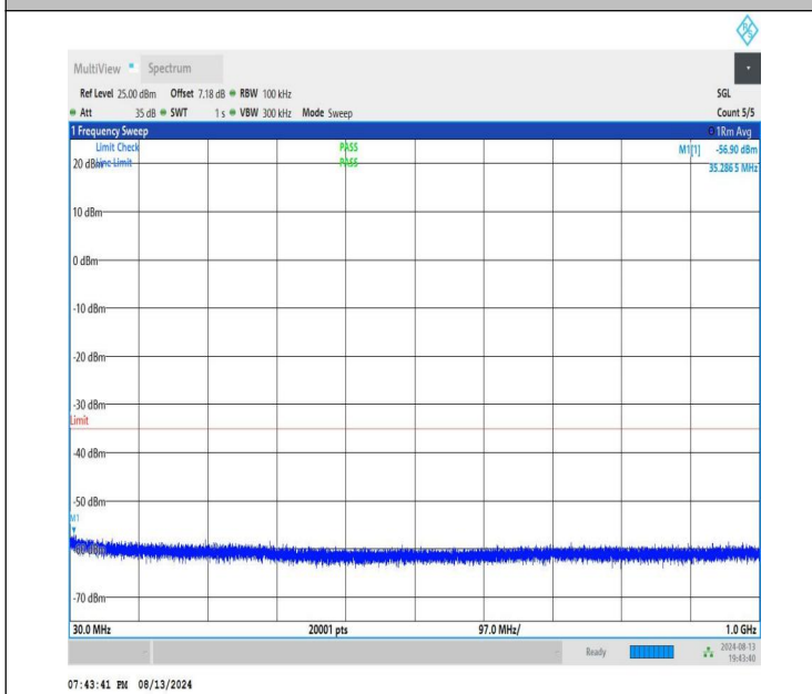
NTNV-n41-PC1.5-30-100-L-CP-QPSK-Edge_1RB_Left-30-1000-P ASS
