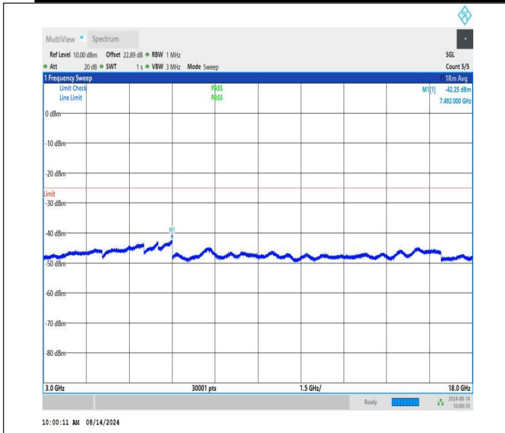
NTNV-n41-PC1.5-30-20-M-CP-QPSK-Edge_1RB_Left-3000-1800 0-PASS
