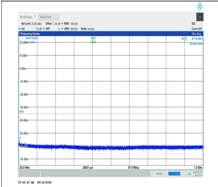
NTNV-n41-PC1.5-30-20-L-CP-QPSK-Edge_1RB_Left-30-1000-PASS
