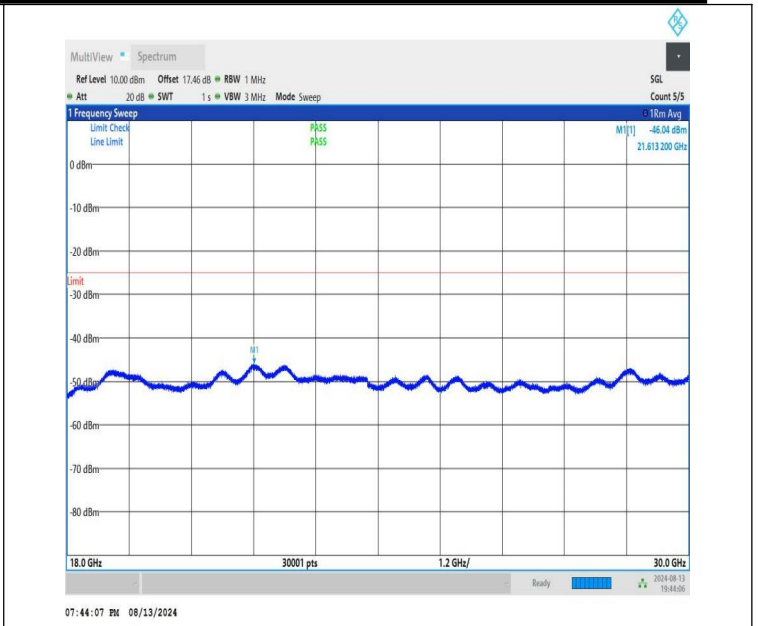
NTVN-n41-PC1.5-30-100-L-CP-QPSK-Edge_1RB_Left-18000-300 00-PASS
