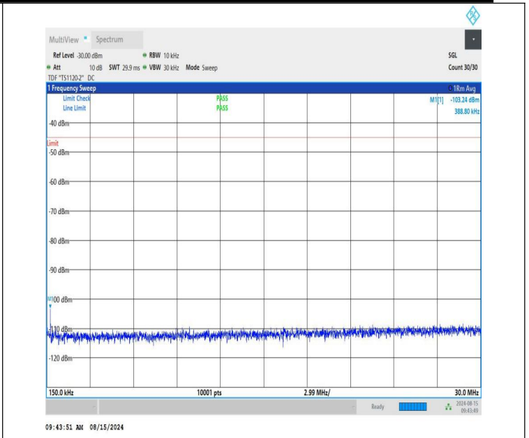
NTNV-n41-PC1.5-30-20-L-CP-QPSK-Edge_1RB_Left-0.15-30-PASS
