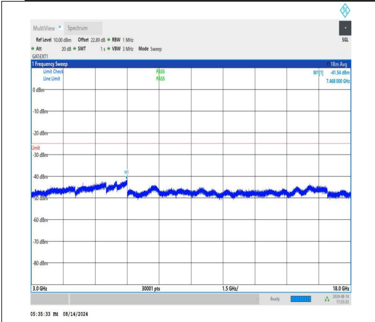
NTNV-n41-PC1.5-30-90-M-CP-QPSK-Edge_1RB_Left-3000-1800 0-PASS
