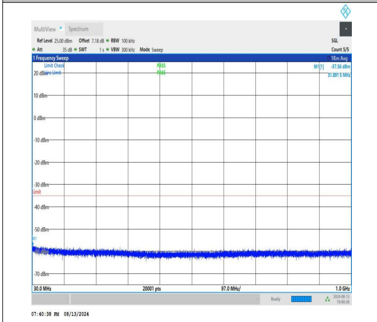
NTNV-n41-PC1.5-30-90-M-CP-QPSK-Edge_1RB_Left-30-1000-P ASS
