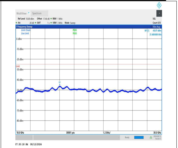
NTVN-n41-PC1.5-30-70-L-CP-QPSK-Edge_1RB_Left-18000-3000 0-PASS
