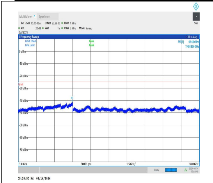
NTVN-n41-PC1.5-30-70-L-CP-QPSK-Edge_1RB_Left-3000-18000 -PASS
