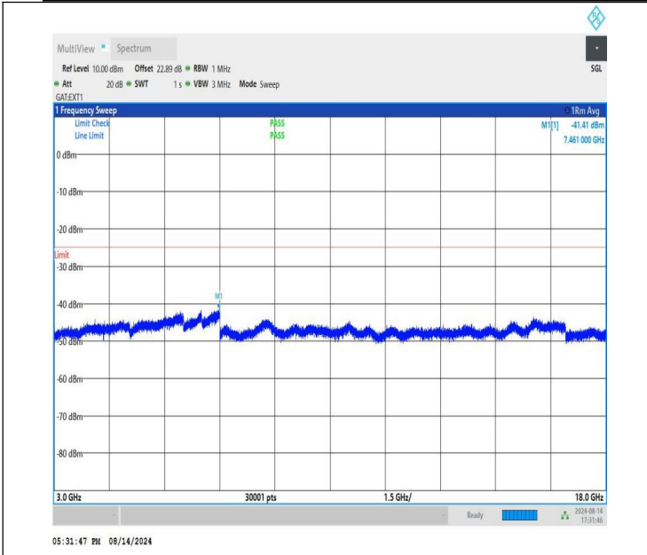
NTVN-n41-PC1.5-30-80-L-CP-QPSK-Edge_1RB_Left-3000-18000 -PASS
