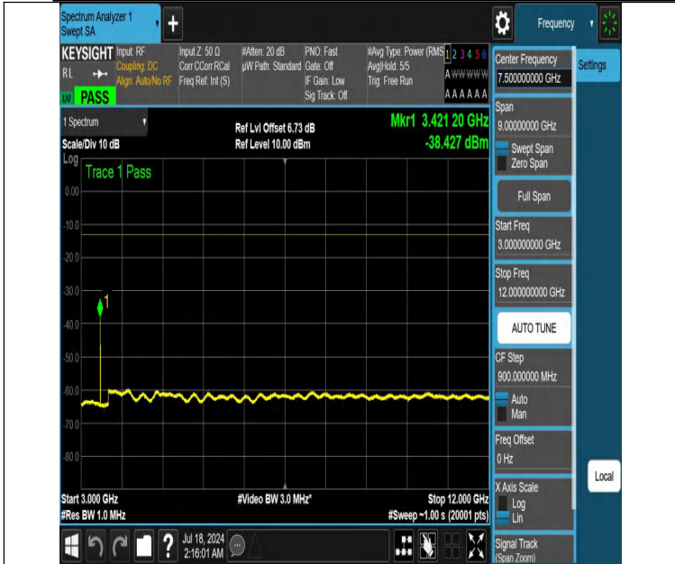
NTNV-DC_12A_n66A-PC3-15-5+40-M+L-N/A-N/A-DFT-QPSK-Edge e_1RB_Left-3000-12000-PASS
