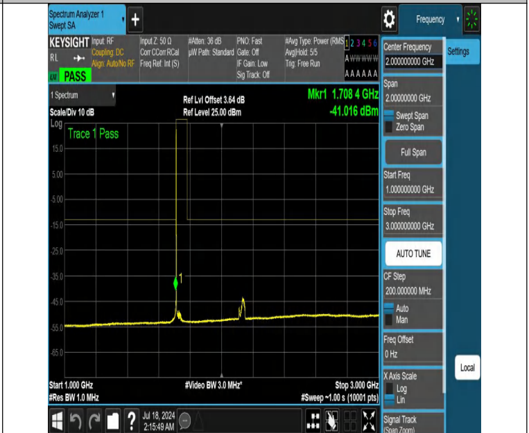
NTNV-DC_12A_n66A-PC3-15-5+40-M+L-N/A-N/A-DFT-QPSK-Edge _1RB_Left-1000-3000-PASS
