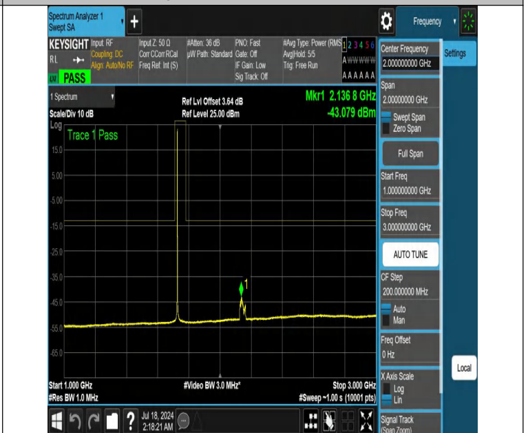
NTNV-DC_12A_n66A-PC3-15-5+40-M+M-N/A-N/A-DFT-PI2BPSK-E dge_1RB_Left-1000-3000-PASS
