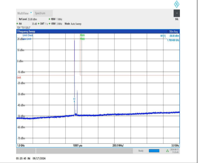
NTNV-DC_12A-n66A-PC3-15-5+35-M+L-QPSK-IDLE-DFT-QPSK-E dge_1RB_Left-1000-3000-PASS
