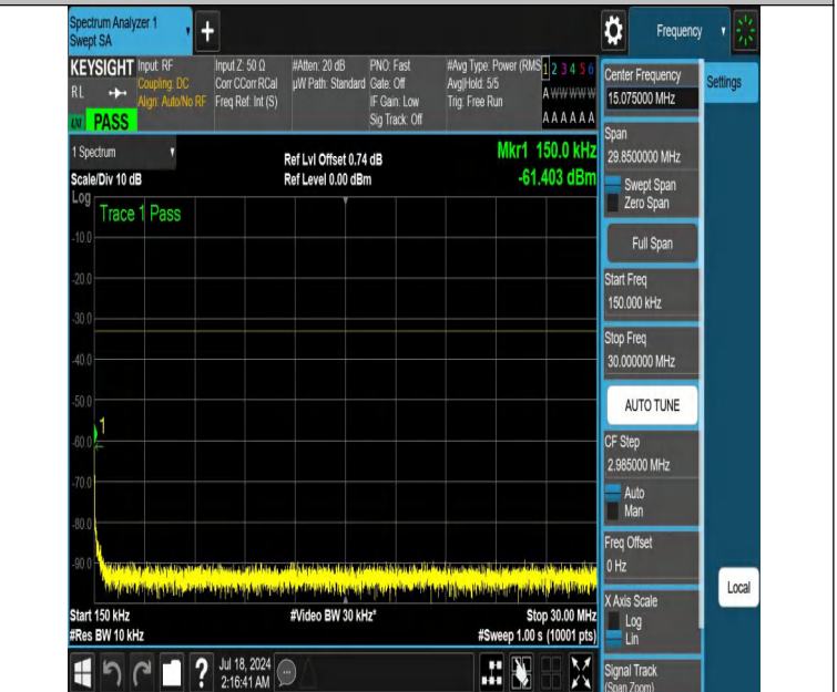
NTNV-DC_12A_n66A-PC3-15-5+40-M+L-N/A-N/A-DFT-QPSK-Edge _1RB_Right-0.15-30-PASS
