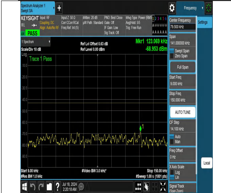
NTNV-DC_12A_n66A-PC3-15-5+40-M+M-N/A-N/A-DFT-QPSK-Edge_1RB_Left-0.009-0.15-PASS
