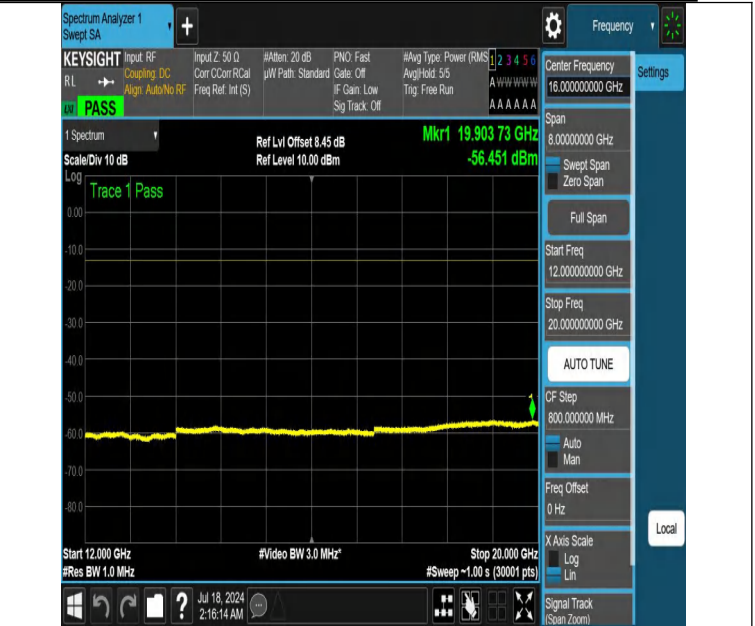
NTNV-DC_12A_n66A-PC3-15-5+40-M+L-N/A-N/A-DFT-QPSK-Edge _1RB_Left-12000-20000-PASS
