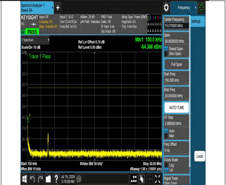
NTNV-DC_12A_n66A-PC3-15-5+40-M+L-N/A-N/A-DFT-QPSK-Edge _1RB_Left-0.15-30-PASS
