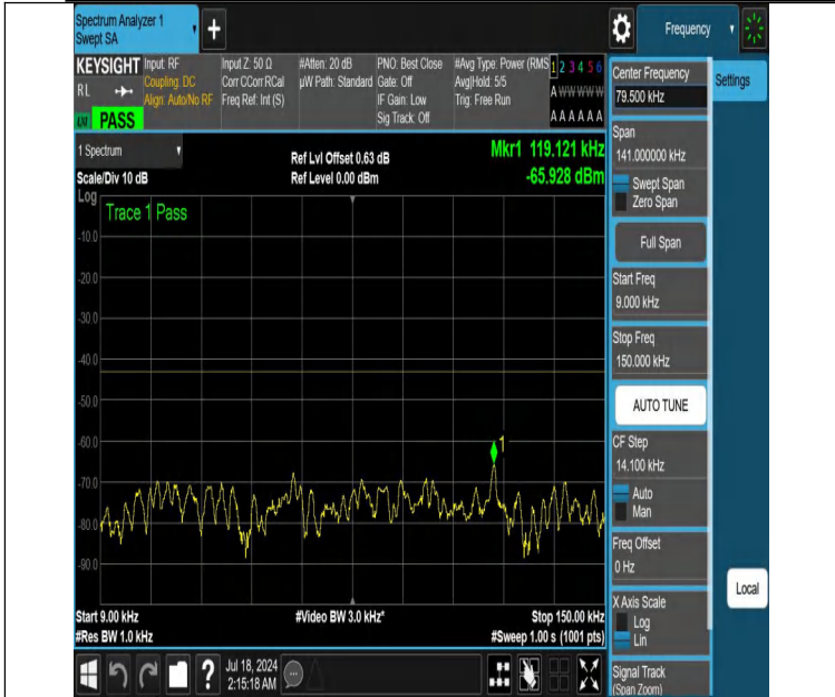
NTNV-DC_12A_n66A-PC3-15-5+40-M+L-N/A-N/A-DFT-QPSK-Edge e_1RB_Left-0.009-0.15-PASS
