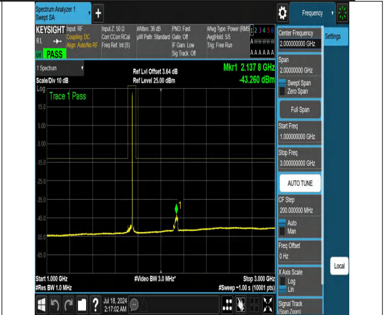
NTNV-DC_12A_n66A-PC3-15-5+40-M+L-N/A-N/A-DFT-QPSK-Edge _1RB_Right-1000-3000-PASS
