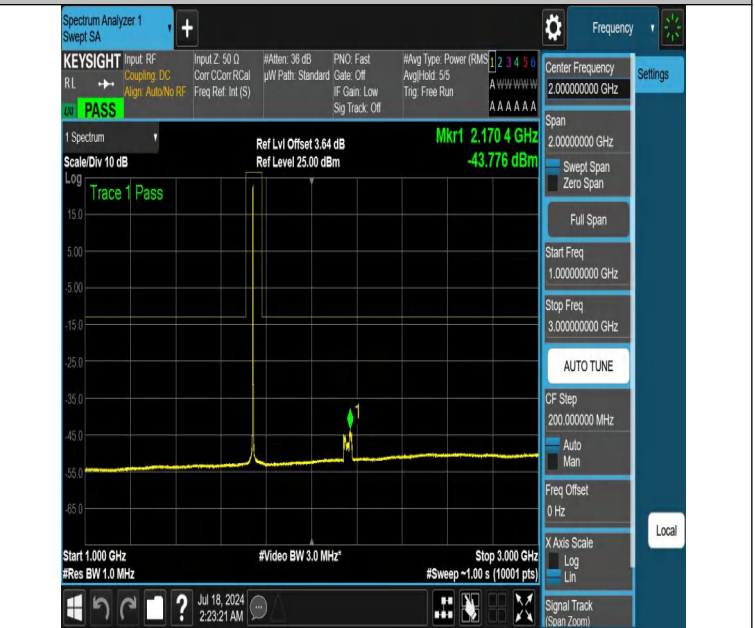
NTNV-DC_12A_n66A-PC3-15-5+40-M+H-N/A-N/A-DFT-PI2BPSK-E dge_1RB_Left-1000-3000-PASS
