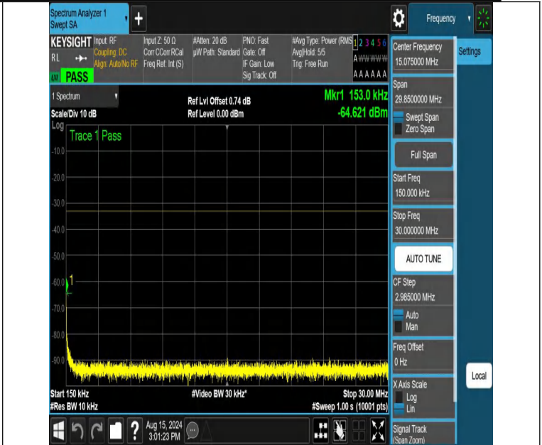
NTNV-DC_12A_n66A-PC3-15-5+30-M+H-N/A-N/A-DFT-PI2BPSK-E dge_1RB_Left-0.15-30-PASS
