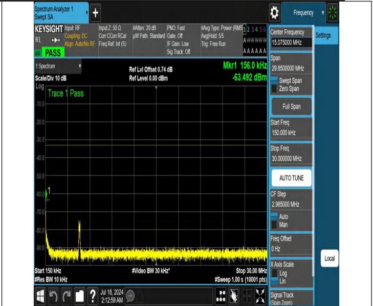
NTNV-DC_12A_n66A-PC3-15-5+40-M+L-N/A-N/A-DFT-PI2BPSK-E dge_1RB_Left-0.15-30-PASS
