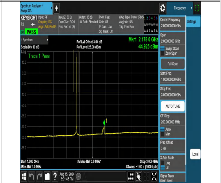
NTNV-DC_12A_n66A-PC3-15-5+30-M+H-N/A-N/A-DFT-PI2BPSK-E dge_1RB_Left-1000-3000-PASS
