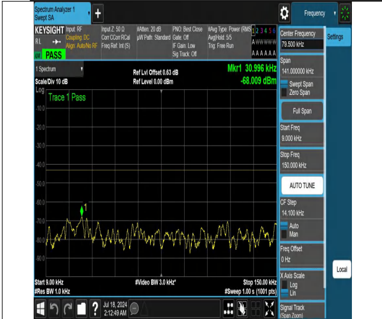
NTNV-DC_12A_n66A-PC3-15-5+40-M+L-N/A-N/A-DFT-PI2BPSK-Edge_1RB_Left-0.009-0.15-PASS
