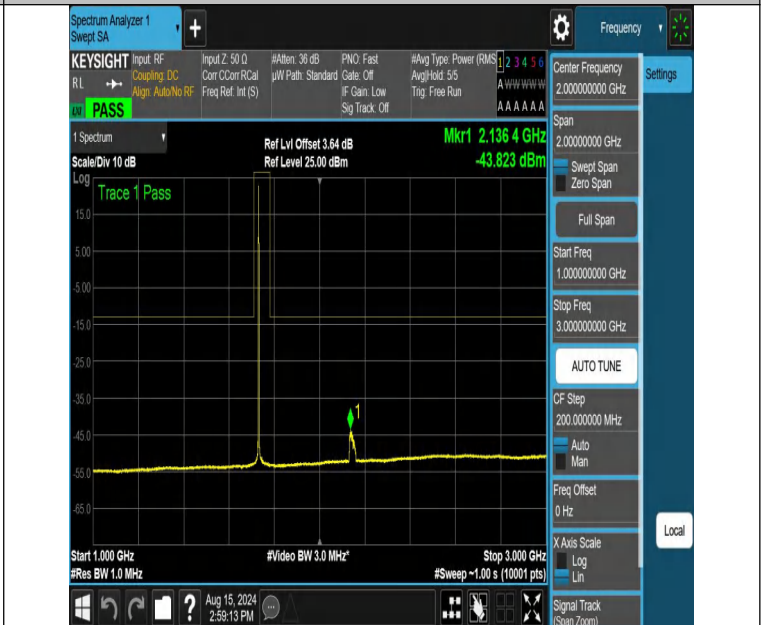
NTNV-DC_12A_n66A-PC3-15-5+30-M+M-N/A-N/A-DFT-QPSK-Edge_1RB_Left-1000-3000-PASS
