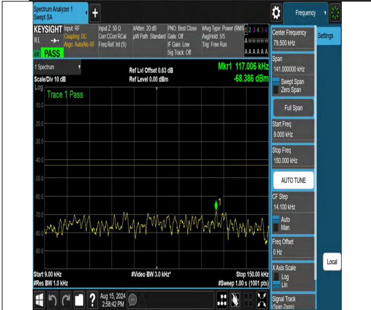
NTNV-DC_12A_n66A-PC3-15-5+30-M+M-N/A-N/A-DFT-QPSK-Edge_1RB_Left-0.009-0.15-PASS
