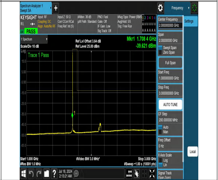
NTNV-DC_12A_n66A-PC3-15-5+40-M+L-N/A-N/A-DFT-PI2BPSK-E dge_1RB_Left-1000-3000-PASS
