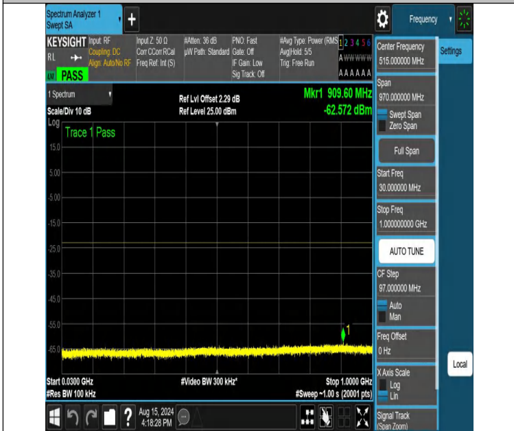
NTNV-DC_12A_n66A-PC3-15-5+25-M+L-N/A-N/A-DFT-QPSK-Edge e_1RB_Left-30-1000-PASS
