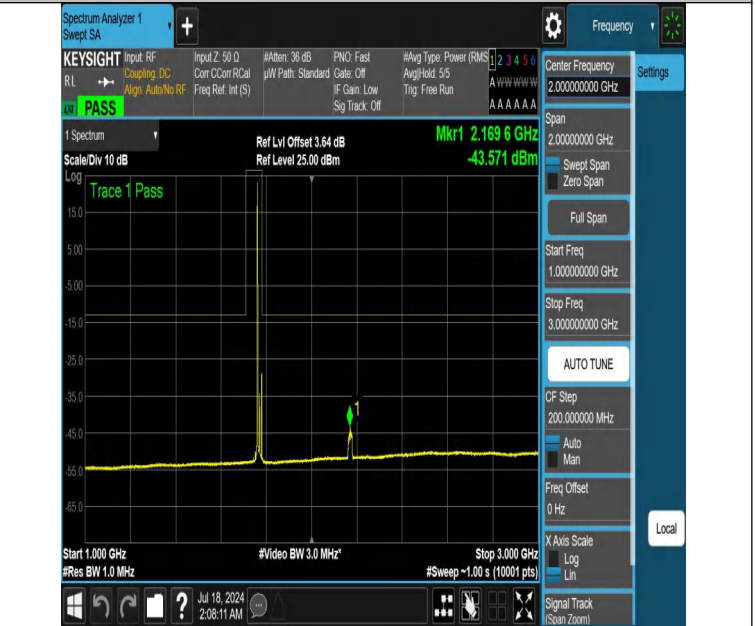
NTNV-DC_12A_n66A-PC3-15-5+20-M+H-N/A-N/A-DFT-PI2BPSK-E dge_1RB_Left-1000-3000-PASS
