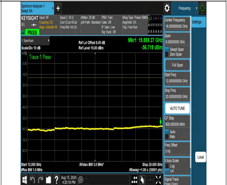
NTNV-DC_12A_n66A-PC3-15-5+25-M+L-N/A-N/A-DFT-QPSK-Edge _1RB_Right-12000-20000-PASS
