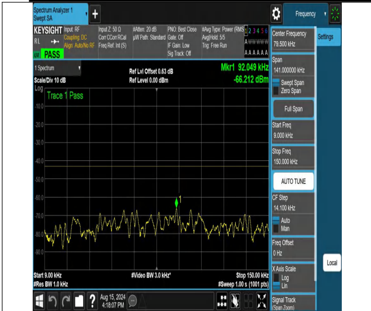
NTNV-DC_12A_n66A-PC3-15-5+25-M+L-N/A-N/A-DFT-QPSK-Edge e_1RB_Left-0.009-0.15-PASS
