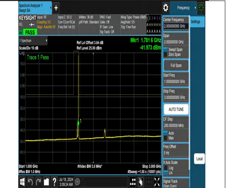
NTNV-DC_12A_n66A-PC3-15-5+20-M+H-N/A-N/A-DFT-PI2BPSK-E dge_1RB_Right-1000-3000-PASS
