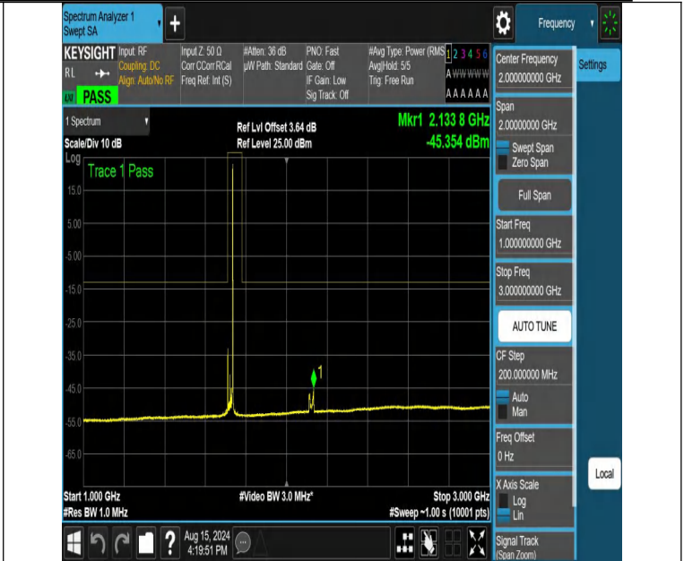
NTNV-DC_12A_n66A-PC3-15-5+25-M+L-N/A-N/A-DFT-QPSK-Edge _1RB_Right-1000-3000-PASS
