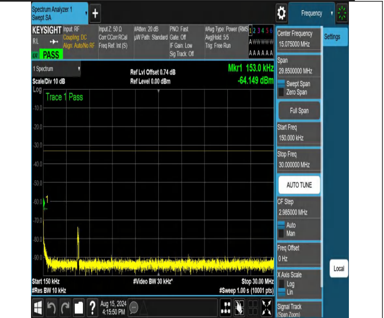
NTNV-DC_12A_n66A-PC3-15-5+25-M+L-N/A-N/A-DFT-PI2BPSK-E dge_1RB_Left-0.15-30-PASS
