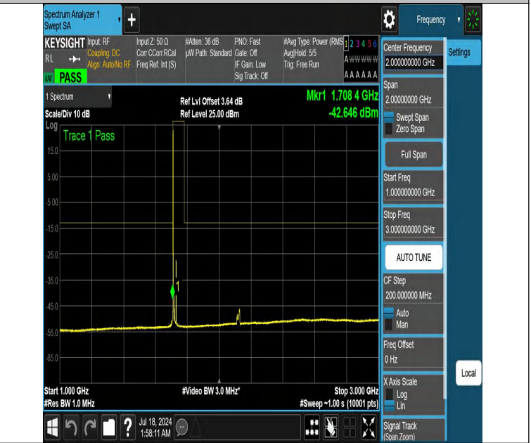
NTNV-DC_12A_n66A-PC3-15-5+20-M+L-N/A-N/A-DFT-PI2BPSK-E dge_1RB_Left-1000-3000-PASS
