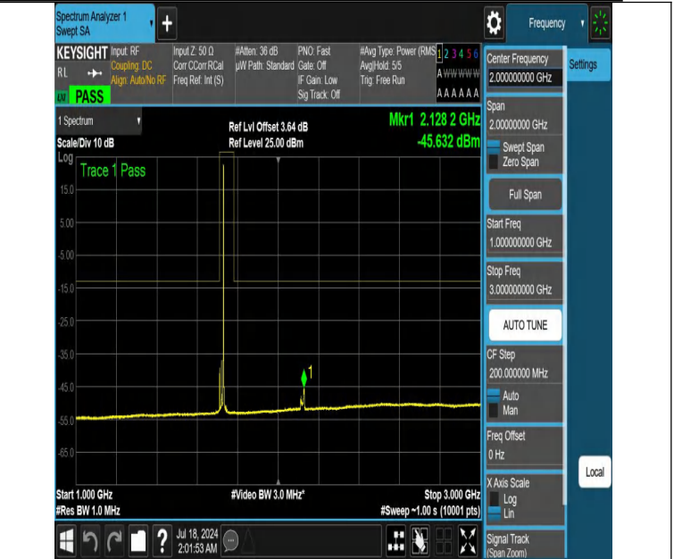
NTNV-DC_12A_n66A-PC3-15-5+20-M+L-N/A-N/A-DFT-QPSK-Edge _1RB_Right-1000-3000-PASS
