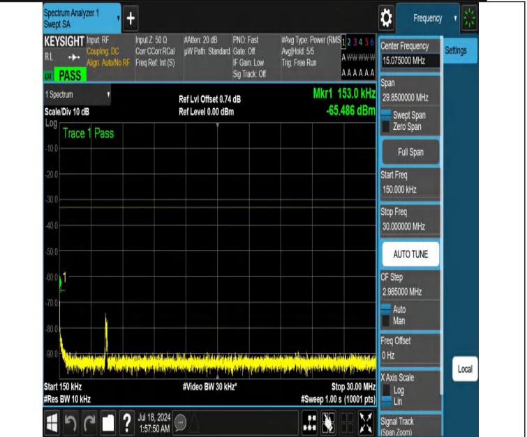
NTNV-DC_12A_n66A-PC3-15-5+20-M+L-N/A-N/A-DFT-PI2BPSK-E dge_1RB_Left-0.15-30-PASS
