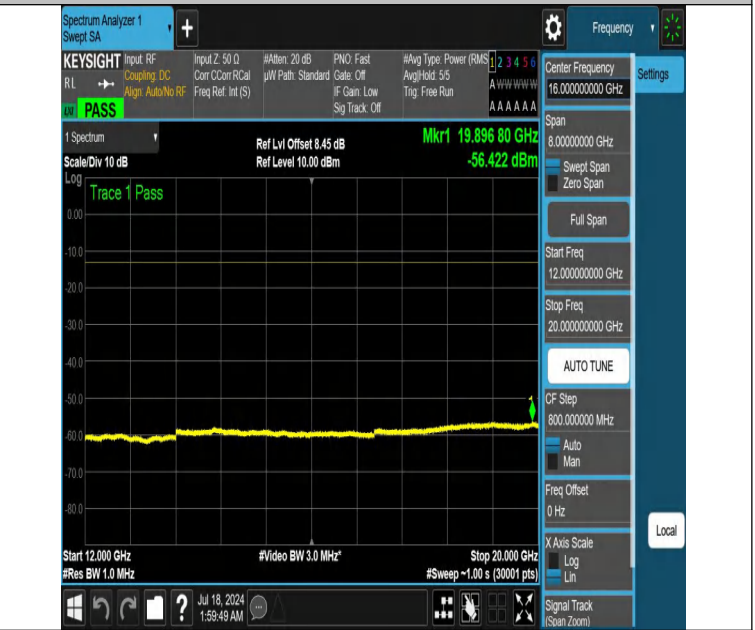
NTNV-DC_12A_n66A-PC3-15-5+20-M+L-N/A-N/A-DFT-PI2BPSK-E dge_1RB_Right-12000-20000-PASS
