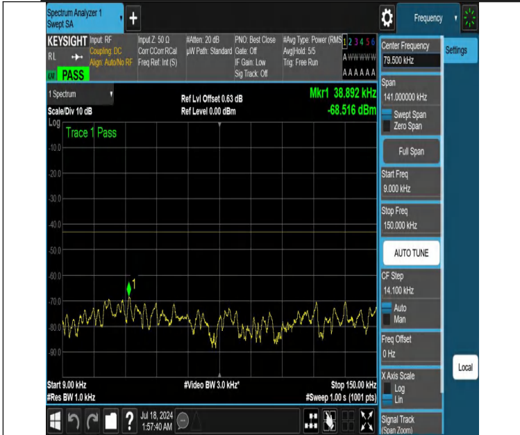
NTNV-DC_12A_n66A-PC3-15-5+20-M+L-N/A-N/A-DFT-PI2BPSK-Edge_1RB_Left-0.009-0.15-PASS
