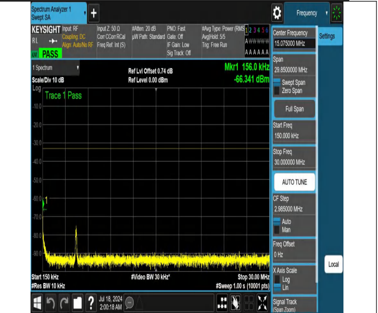
NTNV-DC_12A_n66A-PC3-15-5+20-M+L-N/A-N/A-DFT-QPSK-Edge _1RB_Left-0.15-30-PASS
