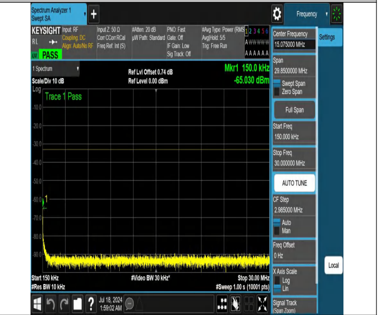
NTNV-DC_12A_n66A-PC3-15-5+20-M+L-N/A-N/A-DFT-PI2BPSK-E dge_1RB_Right-0.15-30-PASS
