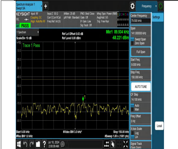
NTNV-DC_12A_n66A-PC3-15-5+20-M+L-N/A-N/A-DFT-QPSK-Edge e_1RB_Left-0.009-0.15-PASS
