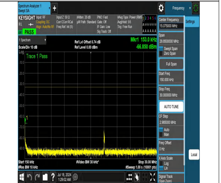
NTNV-DC_12A_n66A-PC3-15-5+10-M+L-N/A-N/A-DFT-PI2BPSK-E dge_1RB_Right-0.15-30-PASS
