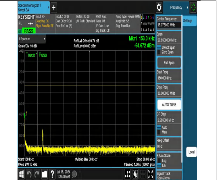
NTNV-DC_12A_n66A-PC3-15-5+10-M+L-N/A-N/A-DFT-PI2BPSK-E dge_1RB_Left-0.15-30-PASS
