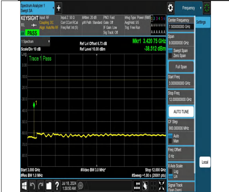
NTNV-DC_12A_n66A-PC3-15-5+10-M+L-N/A-N/A-DFT-QPSK-Edge e_1RB_Left-3000-12000-PASS
