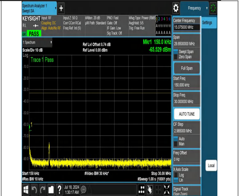
NTNV-DC_12A_n66A-PC3-15-5+10-M+L-N/A-N/A-DFT-QPSK-Edge _1RB_Left-0.15-30-PASS
