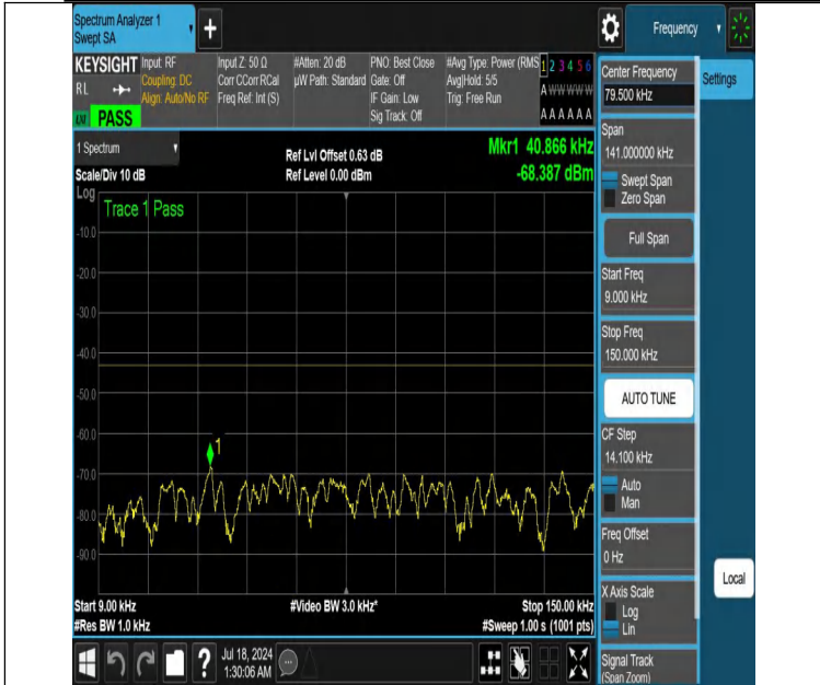
NTNV-DC_12A_n66A-PC3-15-5+10-M+L-N/A-N/A-DFT-QPSK-Edge e_1RB_Left-0.009-0.15-PASS
