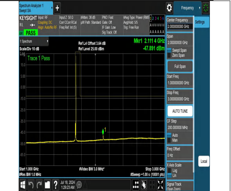
NTNV-DC_12A_n66A-PC3-15-5+10-M+L-N/A-N/A-DFT-PI2BPSK-E dge_1RB_Right-1000-3000-PASS
