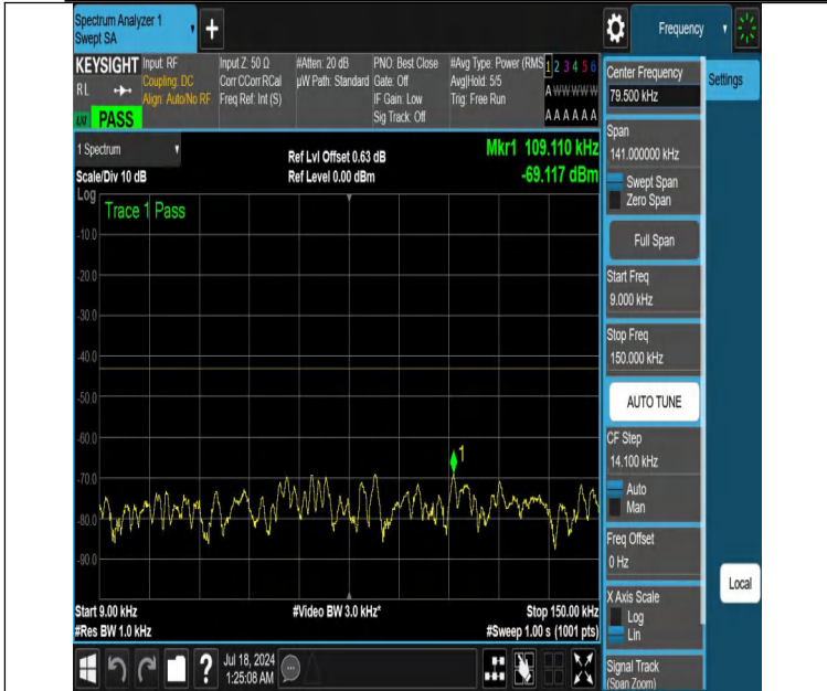
NTNV-DC_12A_n66A-PC3-15-5+5-M+H-N/A-N/A-DFT-QPSK-Edge _1RB_Left-0.009-0.15-PASS
