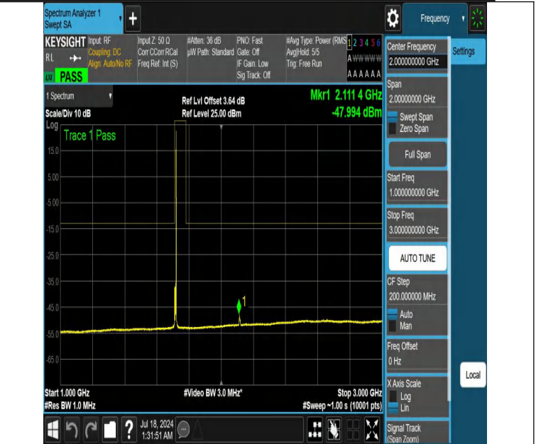
NTNV-DC_12A_n66A-PC3-15-5+10-M+L-N/A-N/A-DFT-QPSK-Edge _1RB_Right-1000-3000-PASS
