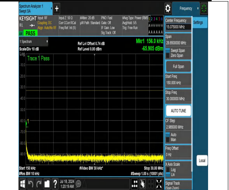
NTNV-DC_12A_n66A-PC3-15-5+5-M+M-N/A-N/A-DFT-QPSK-Edge _1RB_Left-0.15-30-PASS
