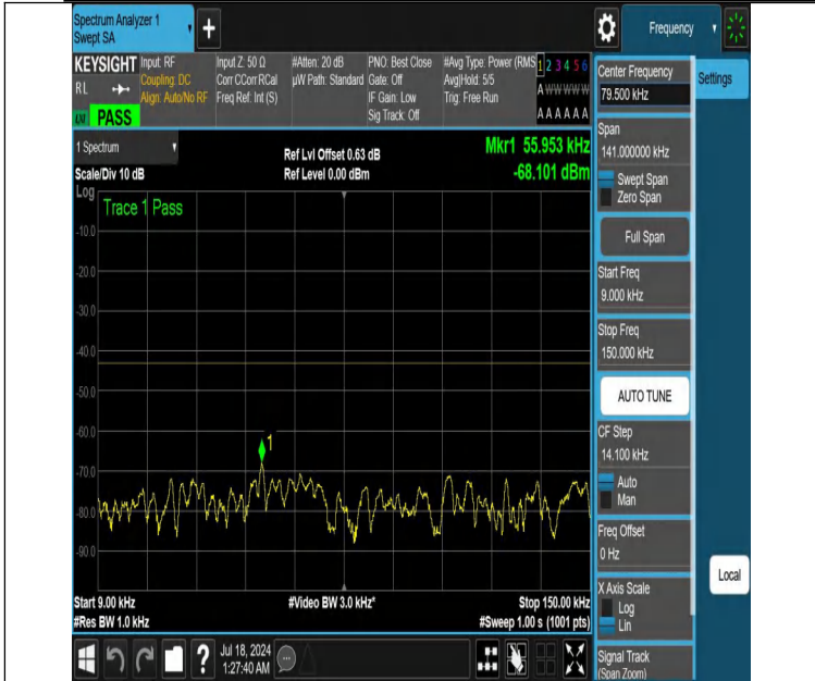
NTNV-DC_12A_n66A-PC3-15-5+10-M+L-N/A-N/A-DFT-PI2BPSK-Edge_1RB_Left-0.009-0.15-PASS
