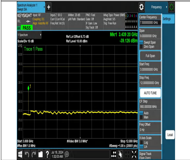
NTNV-DC_12A_n66A-PC3-15-5+10-M+L-N/A-N/A-DFT-QPSK-Edge e_1RB_Right-3000-12000-PASS
