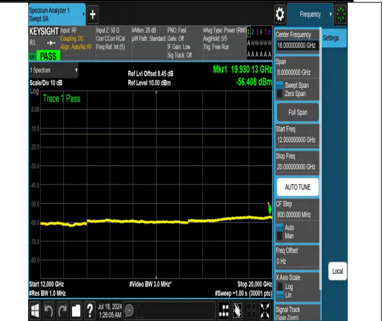
NTNV-DC_12A_n66A-PC3-15-5+5-M+H-N/A-N/A-DFT-QPSK-Edge _1RB_Left-12000-20000-PASS
