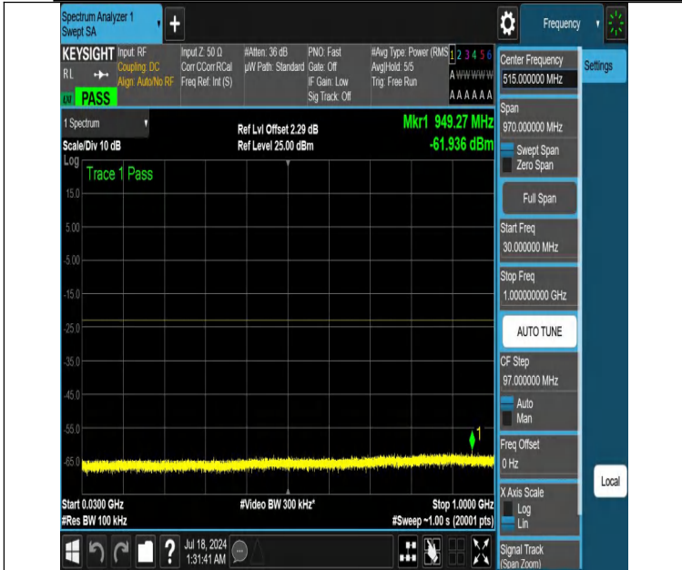
NTNV-DC_12A_n66A-PC3-15-5+10-M+L-N/A-N/A-DFT-QPSK-Edge e_1RB_Right-30-1000-PASS
