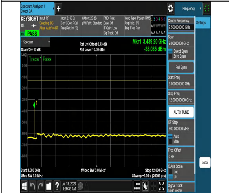
NTNV-DC_12A_n66A-PC3-15-5+10-M+L-N/A-N/A-DFT-PI2BPSK-Edge_1RB_Right-3000-12000-PASS
