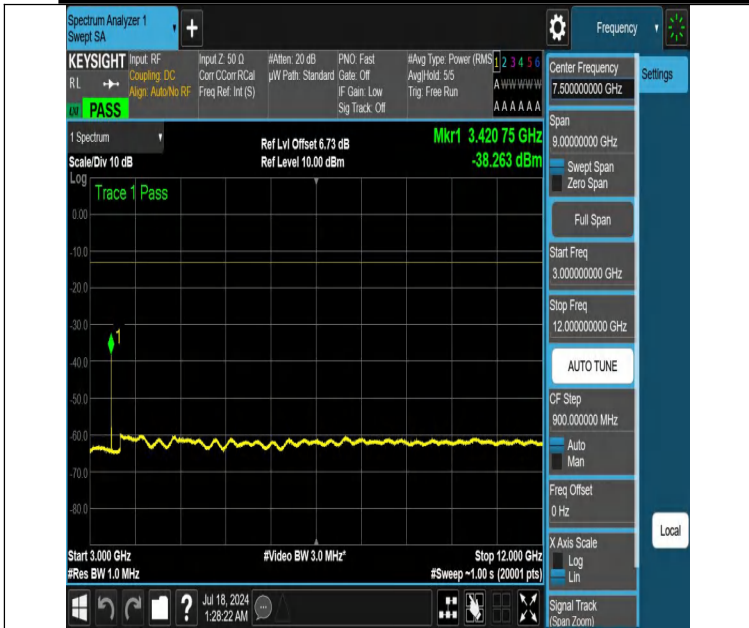
NTNV-DC_12A_n66A-PC3-15-5+10-M+L-N/A-N/A-DFT-PI2BPSK-Edge_1RB_Left-3000-12000-PASS
