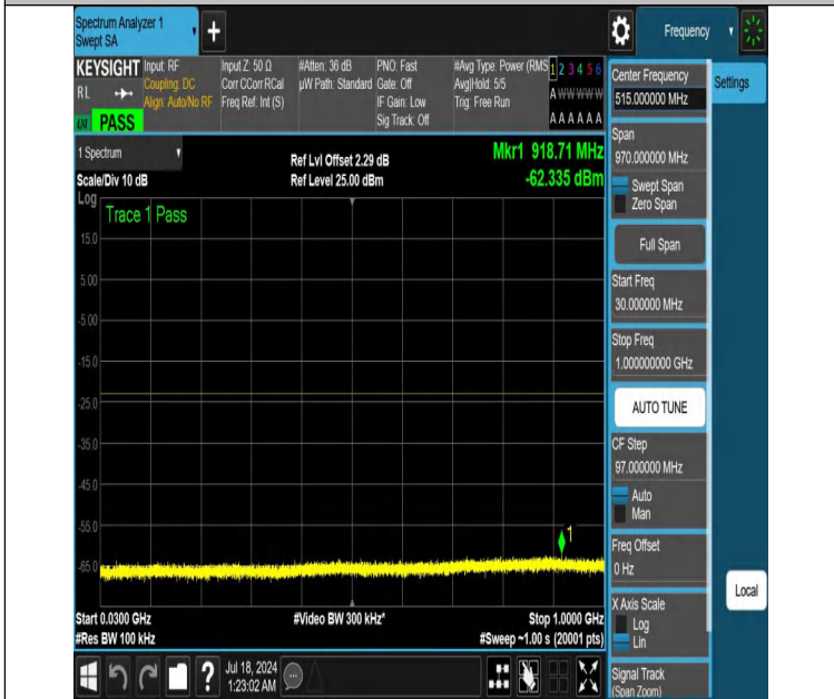
NTNV-DC_12A_n66A-PC3-15-5+5-M+H-N/A-N/A-DFT-PI2BPSK-E dge_1RB_Left-30-1000-PASS
