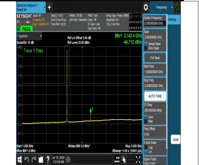
NTNV-DC_12A_n66A-PC3-15-5+5-M+M-N/A-N/A-DFT-QPSK-Edge _1RB_Right-1000-3000-PASS
