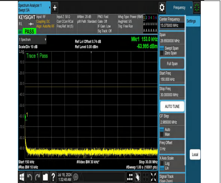
NTNV-DC_12A_n66A-PC3-15-5+10-M+M-N/A-N/A-DFT-PI2BPSK-E dge_1RB_Left-0.15-30-PASS
