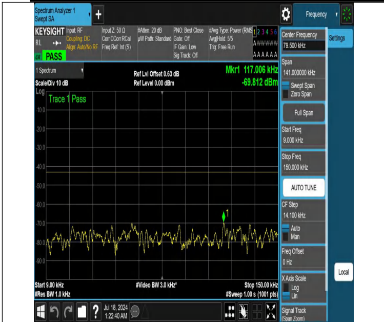
NTNV-DC_12A_n66A-PC3-15-5+5-M+H-N/A-N/A-DFT-PI2BPSK-E dge_1RB_Left-0.009-0.15-PASS
