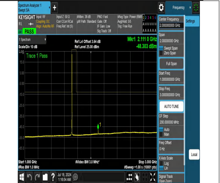
NTNV-DC_12A_n66A-PC3-15-5+5-M+L-N/A-N/A-DFT-QPSK-Edge_1RB_Right-1000-3000-PASS
