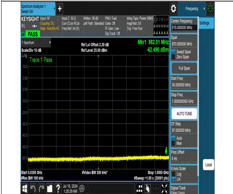
NTNV-DC_12A_n66A-PC3-15-5+5-M+H-N/A-N/A-DFT-QPSK-Edge _1RB_Left-30-1000-PASS
