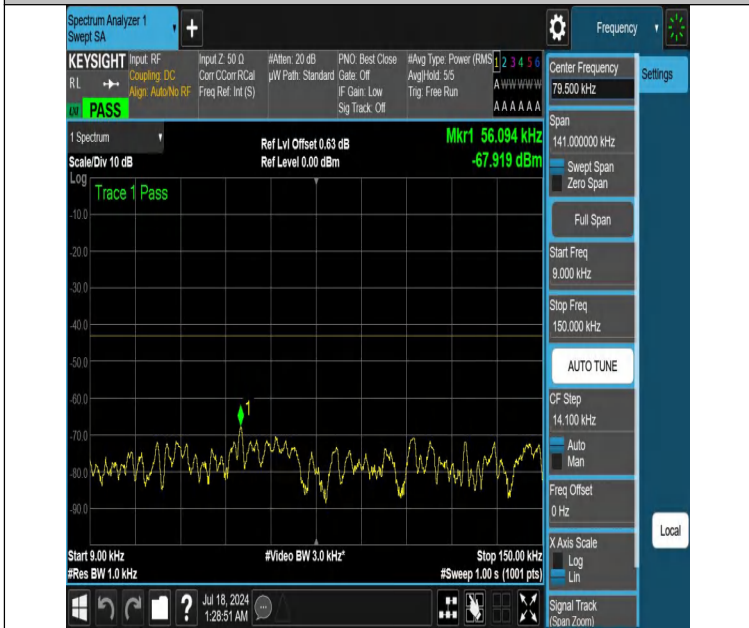
NTNV-DC_12A_n66A-PC3-15-5+10-M+L-N/A-N/A-DFT-PI2BPSK-Edge_1RB_Right-0.009-0.15-PASS
