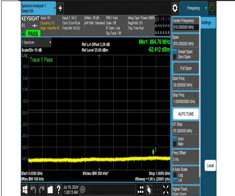
NTNV-DC_12A_n66A-PC3-15-5+10-M+L-N/A-N/A-DFT-PI2BPSK-Edge_1RB_Right-30-1000-PASS
