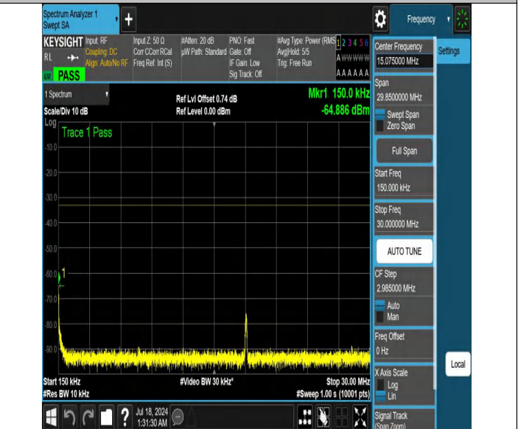
NTNV-DC_12A_n66A-PC3-15-5+10-M+L-N/A-N/A-DFT-QPSK-Edge _1RB_Right-0.15-30-PASS
