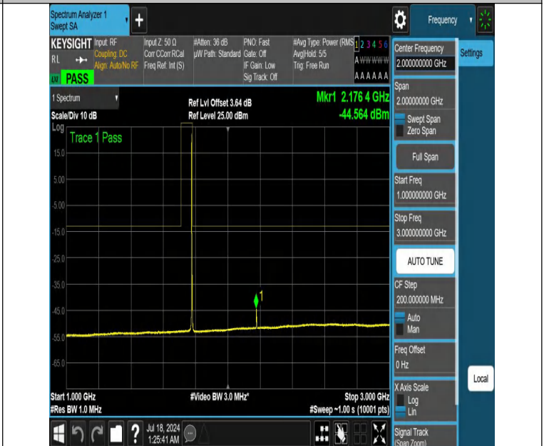
NTNV-DC_12A_n66A-PC3-15-5+5-M+H-N/A-N/A-DFT-QPSK-Edge _1RB_Left-1000-3000-PASS
