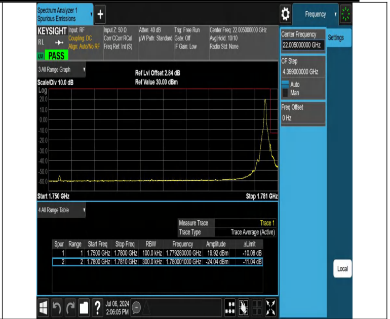
NTNV-DC_12A_n66A-PC3-15-5+30-M+H-N/A-N/A-DFT-PI2BPSK-E dge_1RB_Right-PASS
