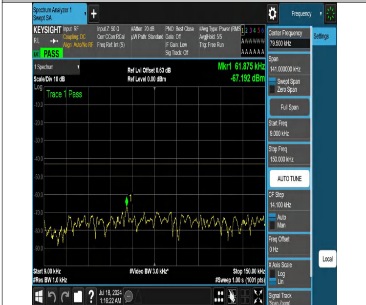
NTNV-DC_12A_n66A-PC3-15-5+5-M+L-N/A-N/A-DFT-QPSK-Edge_1RB_Right-0.009-0.15-PASS
