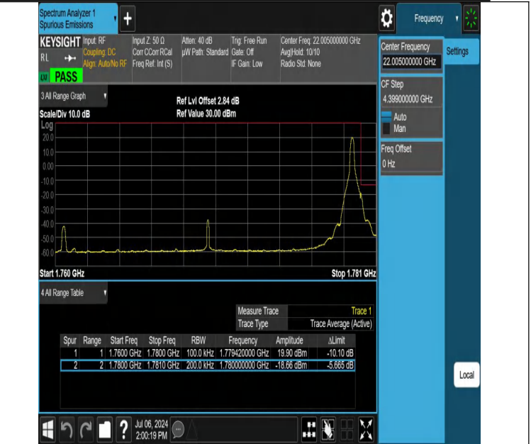
NTNV-DC_12A_n66A-PC3-15-5+20-M+H-N/A-N/A-DFT-PI2BPSK-E dge_1RB_Right-PASS
