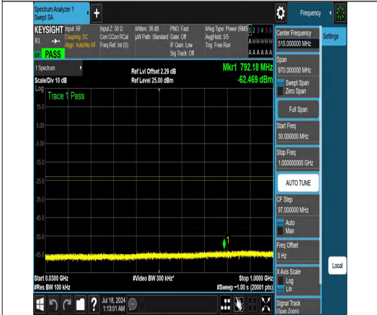
NTNV-DC_12A_n66A-PC3-15-5+5-M+L-N/A-N/A-DFT-PI2BPSK-E dge_1RB_Left-30-1000-PASS
