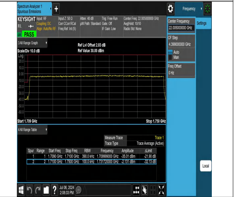
NTVN-DC_12A_n66A-PC3-15-5+40-M+L-N/A-N/A-DFT-QPSK-Outer_Full-PASS
