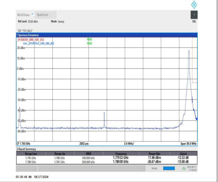
NTVN-DC_12A-n66A-PC3-15-5+35-M+H-QPSK-IDLE-DFT-QPSK-E dge_1RB_Right-PASS
