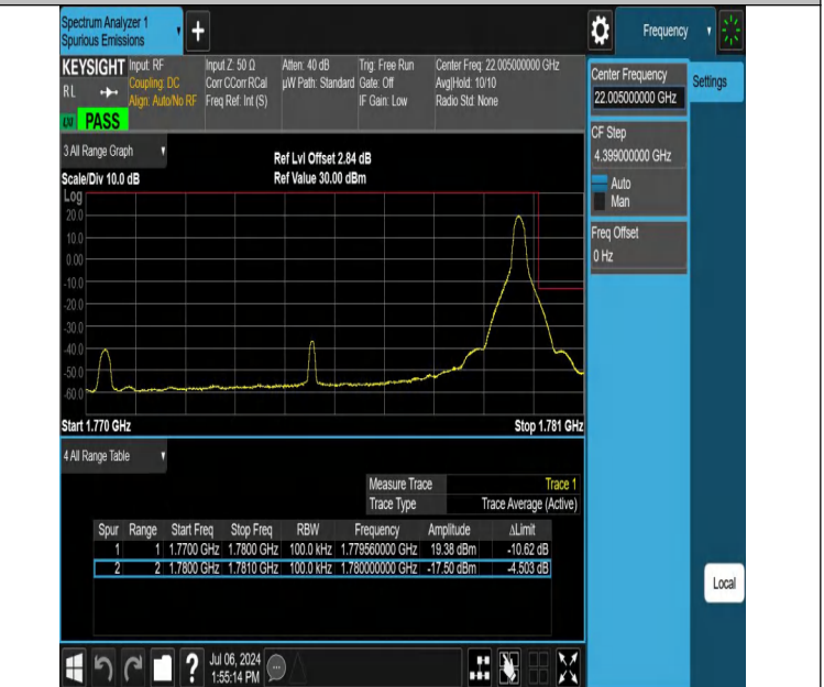
NTNV-DC_12A_n66A-PC3-15-5+10-M+H-N/A-N/A-DFT-QPSK-Edge_1RB_Right-PASS
