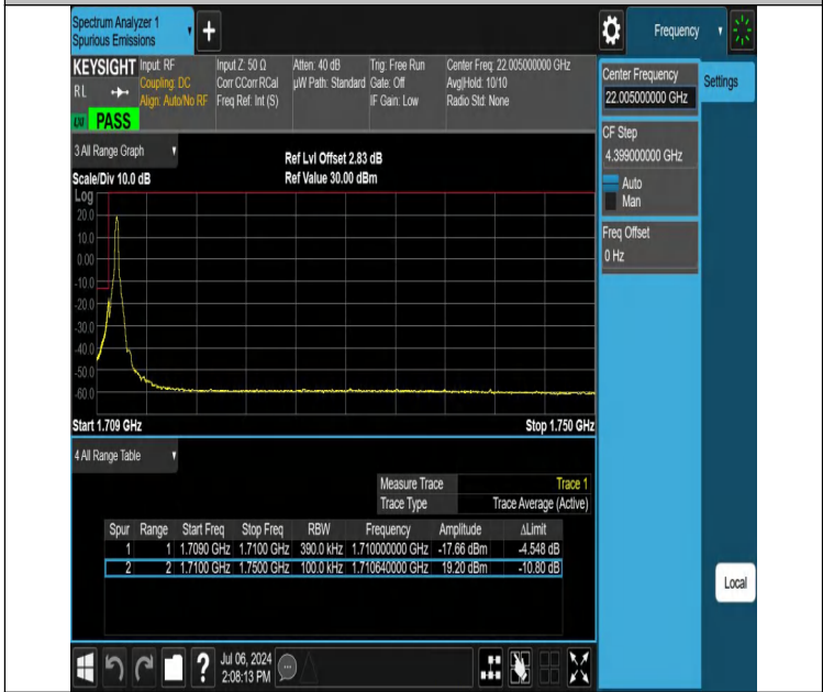
NTVN-DC_12A_n66A-PC3-15-5+40-M+L-N/A-N/A-DFT-QPSK-Edge_1RB_Left-PASS
