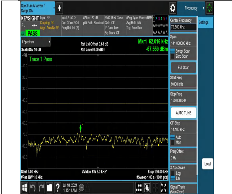
NTNV-DC_12A_n66A-PC3-15-5+5-M+L-N/A-N/A-DFT-QPSK-Edge_1RB_Left-0.009-0.15-PASS
