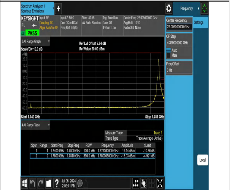
NTVN-DC_12A_n66A-PC3-15-5+40-M+H-N/A-N/A-DFT-QPSK-Edge_1RB_Right-PASS
