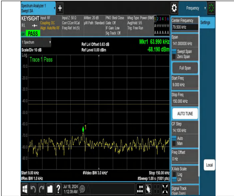
NTNV-DC_12A_n66A-PC3-15-5+5-M+L-N/A-N/A-DFT-PI2BPSK-E dge_1RB_Left-0.009-0.15-PASS
