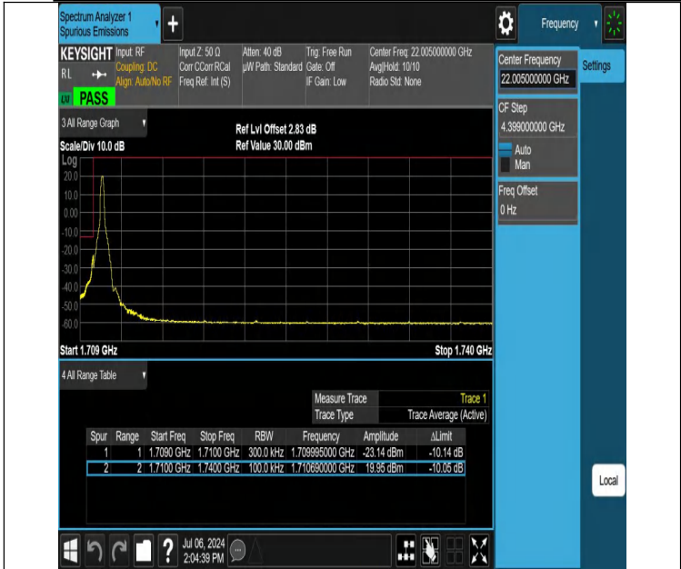
NTVN-DC_12A_n66A-PC3-15-5+30-M+L-N/A-N/A-DFT-PI2BPSK-Edge_1RB_Left-PASS
