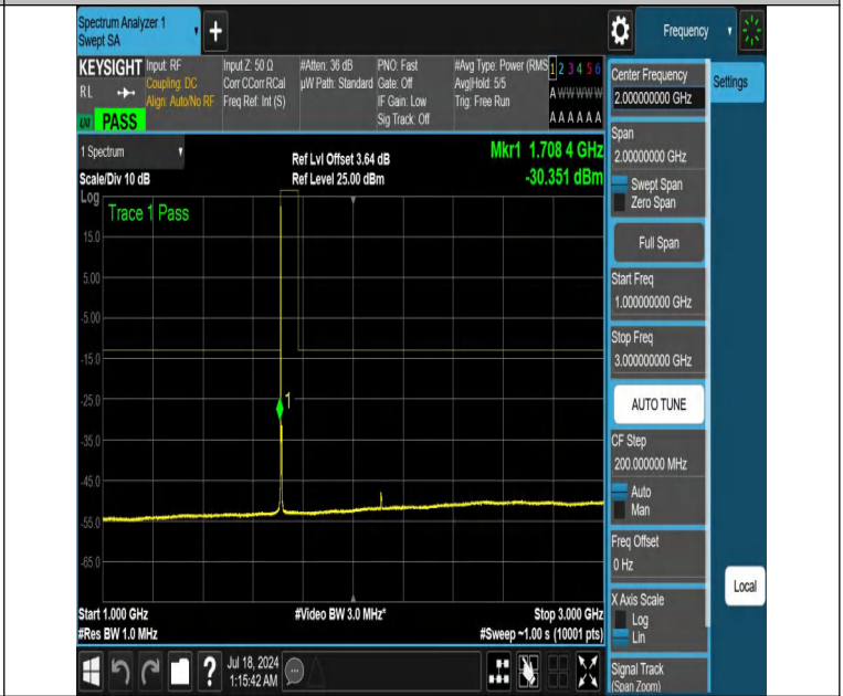
NTNV-DC_12A_n66A-PC3-15-5+5-M+L-N/A-N/A-DFT-QPSK-Edge_1RB_Left-1000-3000-PASS
