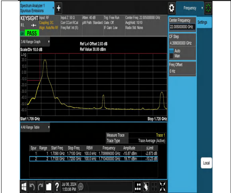
NTVN-DC_12A_n66A-PC3-15-5+10-M+L-N/A-N/A-DFT-PI2BPSK-Edge_1RB_Left-PASS
