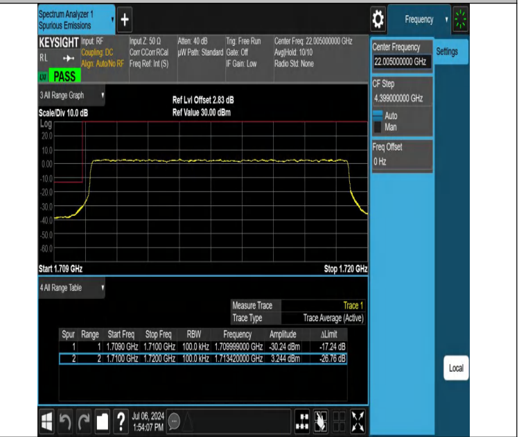
NTVN-DC_12A_n66A-PC3-15-5+10-M+L-N/A-N/A-DFT-QPSK-Outer_Full-PASS
