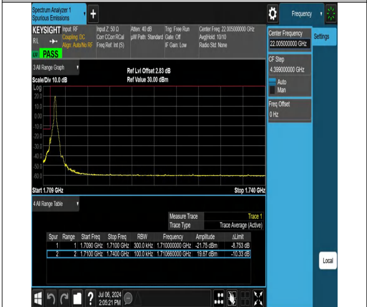
NTVN-DC_12A_n66A-PC3-15-5+30-M+L-N/A-N/A-DFT-QPSK-Edge_1RB_Left-PASS
