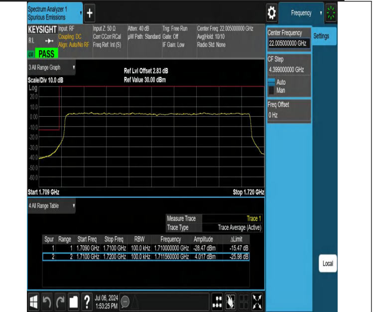
NTVN-DC_12A_n66A-PC3-15-5+10-M+L-N/A-N/A-DFT-PI2BPSK-Outer_Full-PASS
