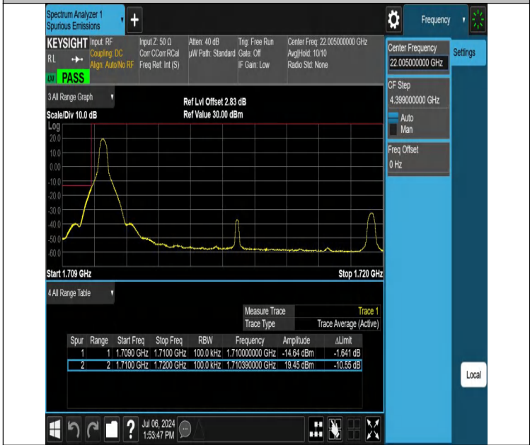
NTVN-DC_12A_n66A-PC3-15-5+10-M+L-N/A-N/A-DFT-QPSK-Edge_1RB_Left-PASS
