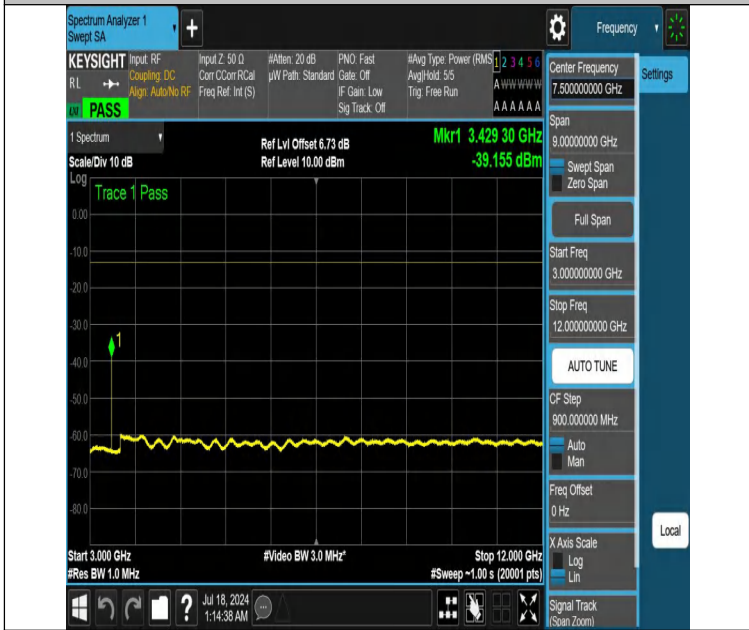
NTNV-DC_12A_n66A-PC3-15-5+5-M+L-N/A-N/A-DFT-PI2BPSK-E dge_1RB_Right-3000-12000-PASS
