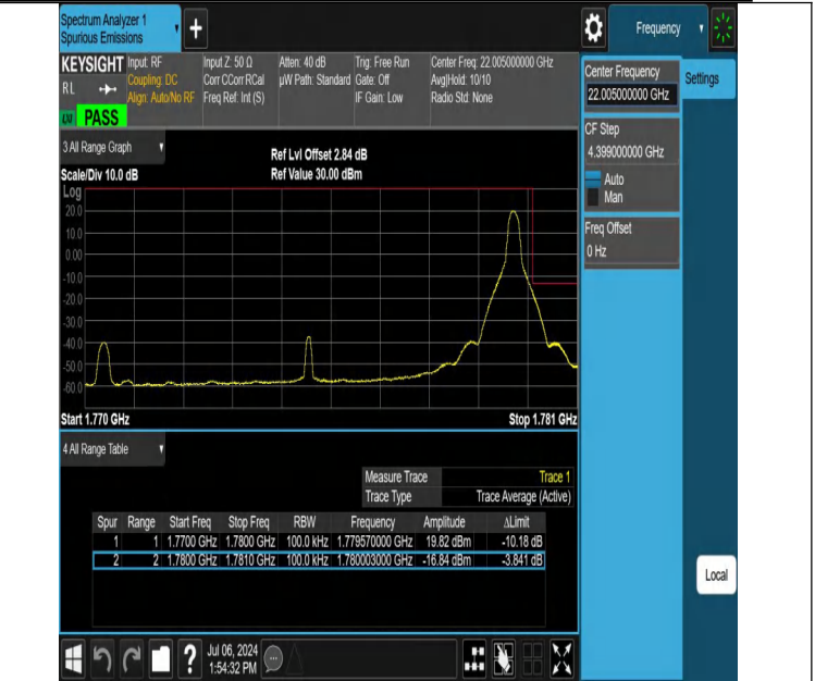
NTNV-DC_12A_n66A-PC3-15-5+10-M+H-N/A-N/A-DFT-PI2BPSK-E dge_1RB_Right-PASS
