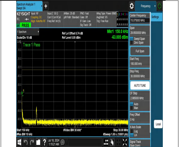
NTNV-DC_12A_n66A-PC3-15-5+5-M+L-N/A-N/A-DFT-QPSK-Edge_1RB_Left-0.15-30-PASS
