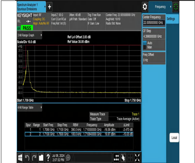
NTVN-DC_12A_n66A-PC3-15-5+40-M+L-N/A-N/A-DFT-PI2BPSK-Edge_1RB_Left-PASS
