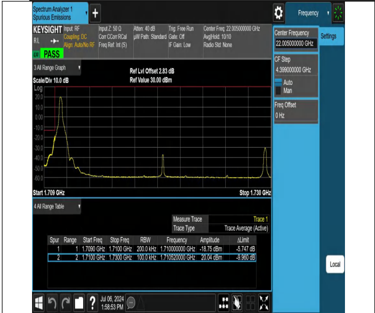
NTVN-DC_12A_n66A-PC3-15-5+20-M+L-N/A-N/A-DFT-PI2BPSK-Edge_1RB_Left-PASS
