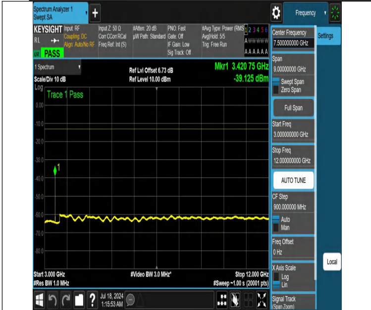
NTNV-DC_12A_n66A-PC3-15-5+5-M+L-N/A-N/A-DFT-QPSK-Edge_1RB_Left-3000-12000-PASS
