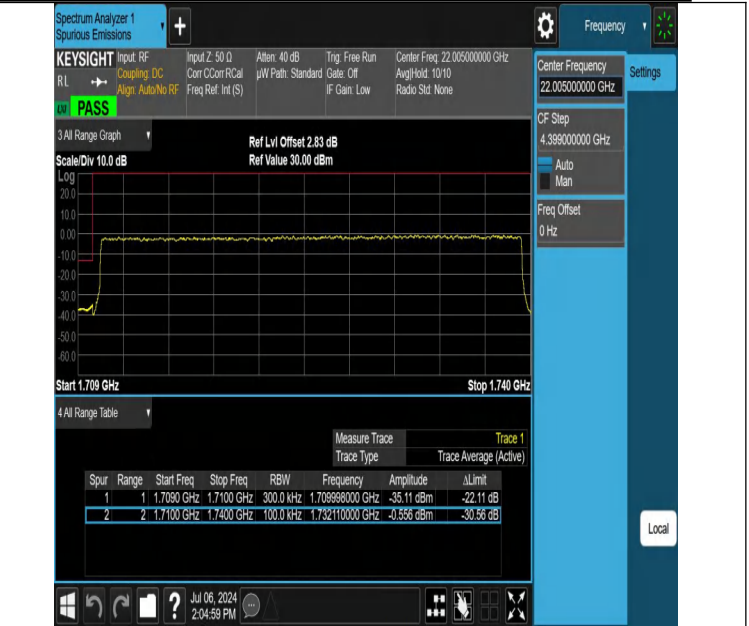
NTVN-DC_12A_n66A-PC3-15-5+30-M+L-N/A-N/A-DFT-PI2BPSK-Outer_Full-PASS
