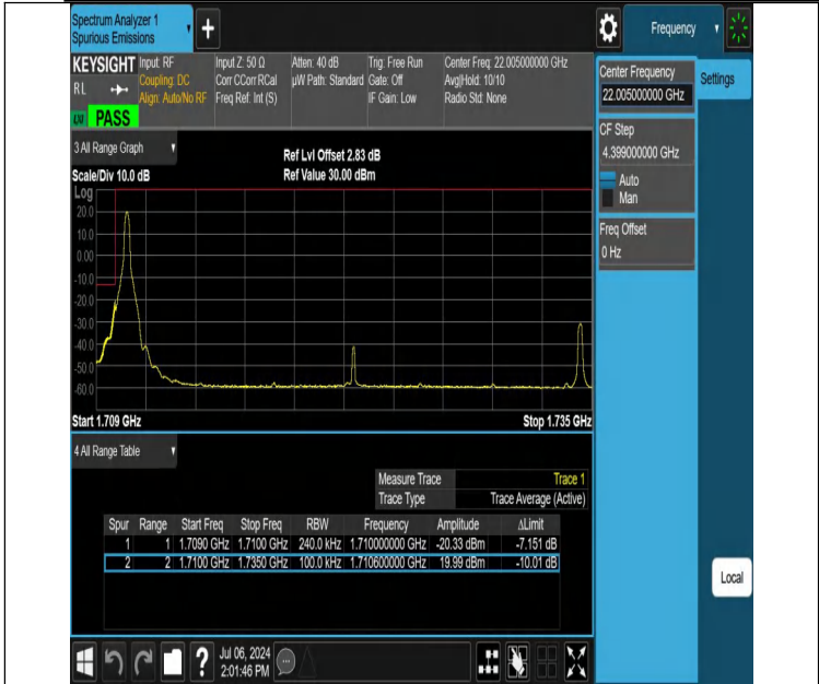
NTVN-DC_12A_n66A-PC3-15-5+25-M+L-N/A-N/A-DFT-PI2BPSK-Edge_1RB_Left-PASS
