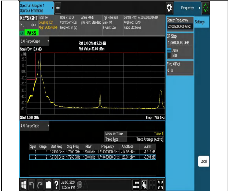
NTVN-DC_12A_n66A-PC3-15-5+15-M+L-N/A-N/A-DFT-PI2BPSK-Edge_1RB_Left-PASS
