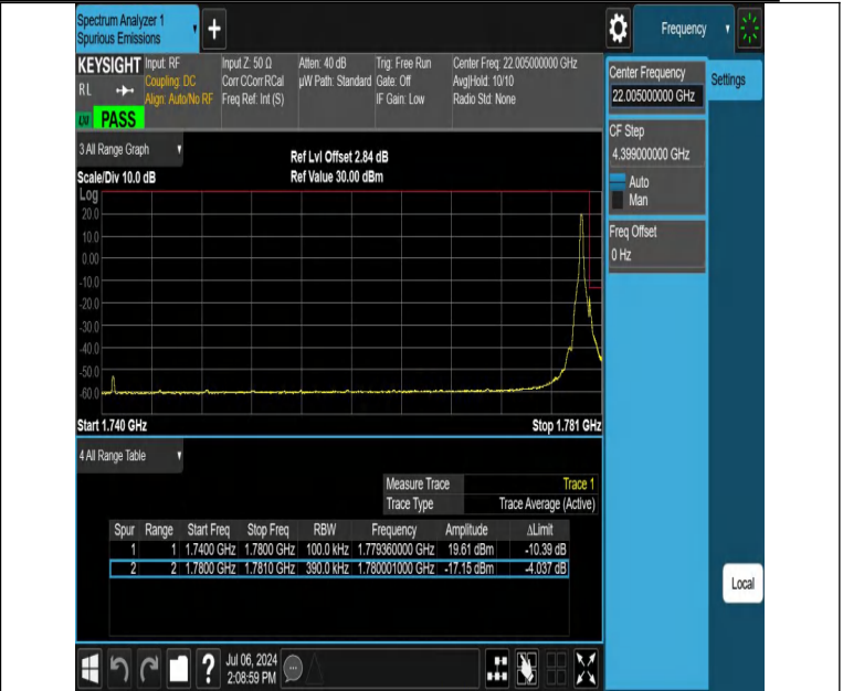
NTVN-DC_12A_n66A-PC3-15-5+40-M+H-N/A-N/A-DFT-PI2BPSK-E dge_1RB_Right-PASS
