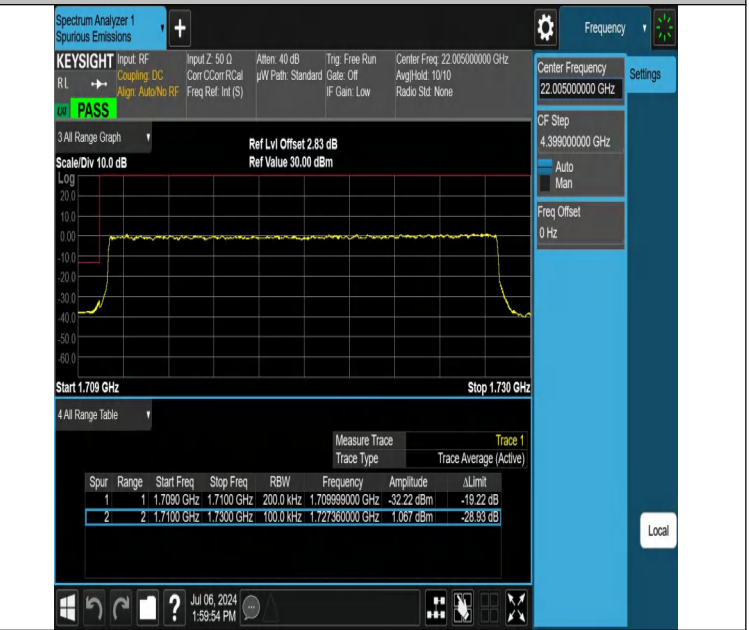
NTVN-DC_12A_n66A-PC3-15-5+20-M+L-N/A-N/A-DFT-QPSK-Outer_Full-PASS
