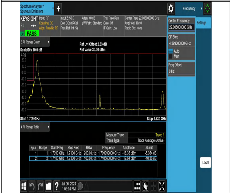
NTVN-DC_12A_n66A-PC3-15-5+20-M+L-N/A-N/A-DFT-QPSK-Edge_1RB_Left-PASS
