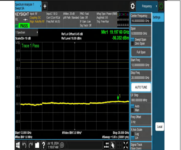
NTNV-DC_12A_n66A-PC3-15-5+5-M+L-N/A-N/A-DFT-QPSK-Edge_1RB_Left-12000-20000-PASS
