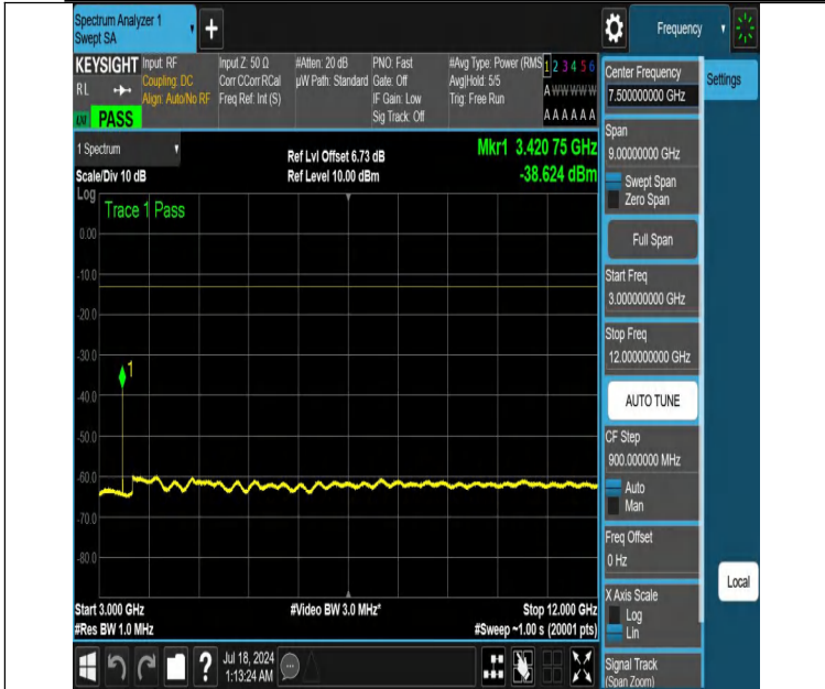
NTNV-DC_12A_n66A-PC3-15-5+5-M+L-N/A-N/A-DFT-PI2BPSK-E dge_1RB_Left-3000-12000-PASS
