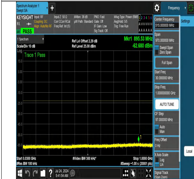
NTNV-N66-PC3-15-40-L-DFT-QPSK-Edge_1RB_Left-30-1000-Ant1-PASS
