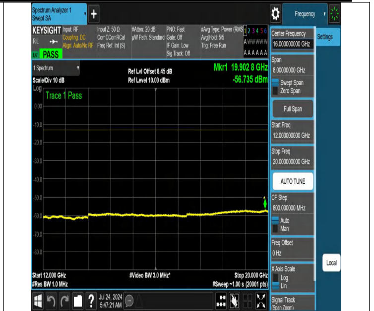
NTNV-N66-PC3-15-40-M-DFT-QPSK-Edge_1RB_Left-12000-200 00-Ant1-PASS
