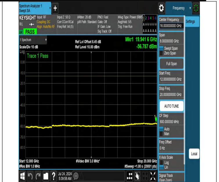
NTNV-N66-PC3-15-40-L-DFT-PI2BPSK-Edge_1RB_Left-12000-20000-Ant1-PASS
