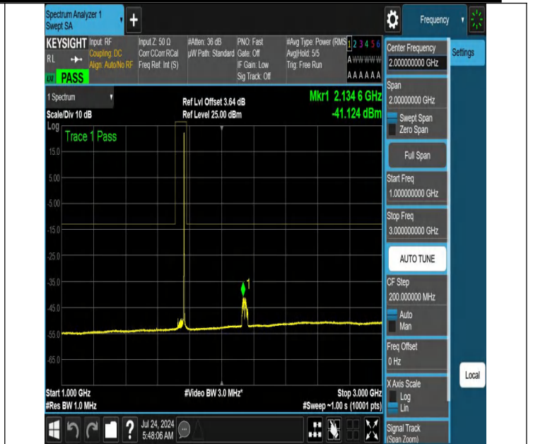
NTNV-N66-PC3-15-40-M-DFT-QPSK-Edge_1RB_Right-1000-300-0-Ant1-PASS
