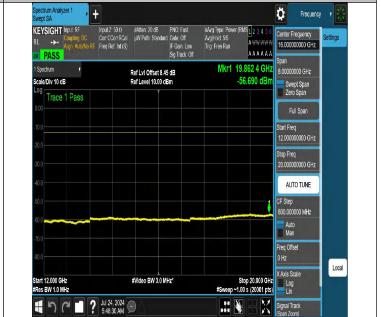
NTNV-N66-PC3-15-40-M-DFT-QPSK-Edge_1RB_Right-12000-20000-Ant1-PASS
