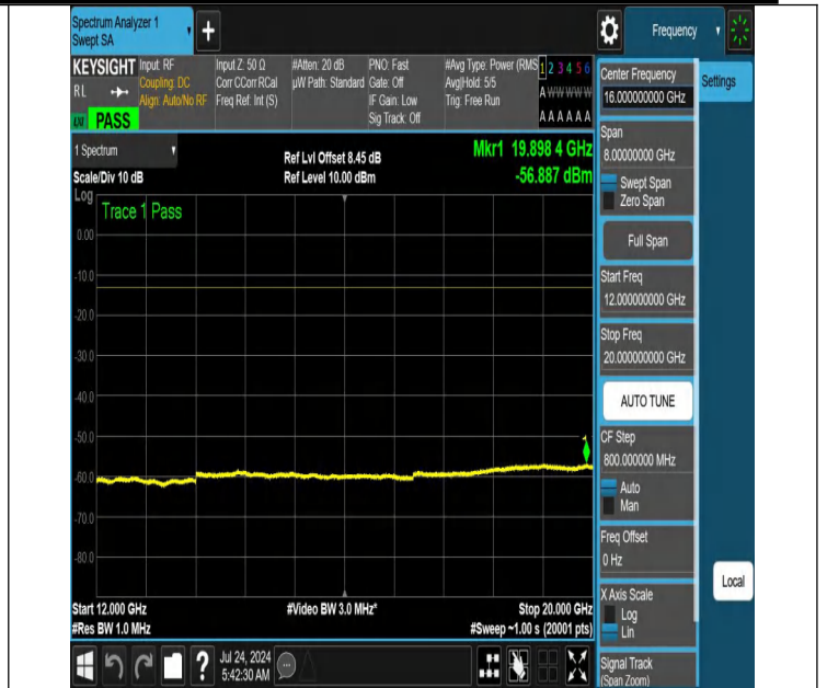
NTNV-N66-PC3-15-40-L-DFT-QPSK-Edge_1RB_Left-12000-2000 0-Ant1-PASS
