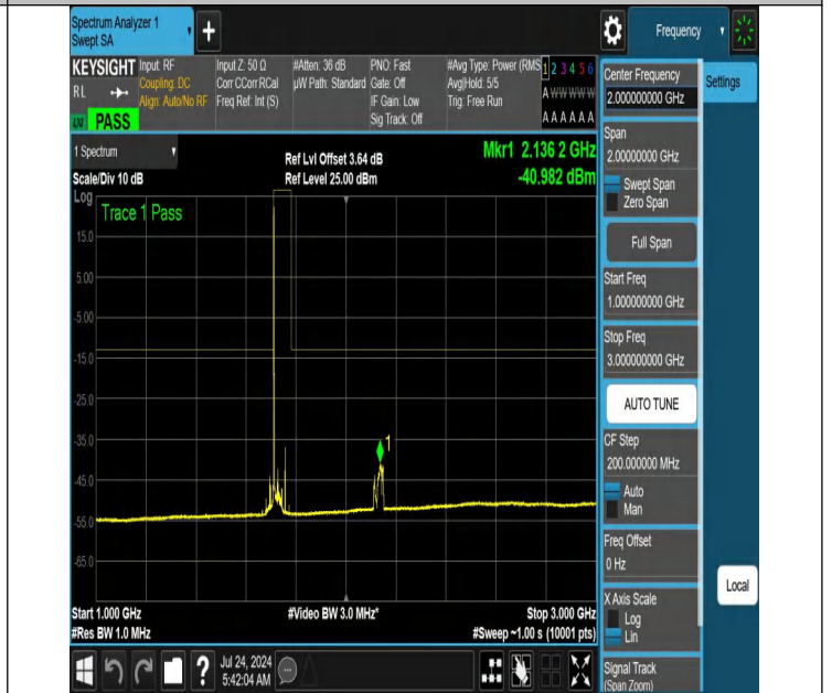
NTNV-N66-PC3-15-40-L-DFT-QPSK-Edge_1RB_Left-1000-3000-Ant1-PASS
