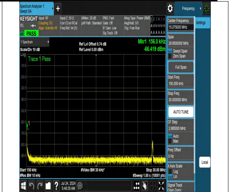
NTNV-N66-PC3-15-40-M-DFT-QPSK-Edge_1RB_Left-0.15-30-Ant 1-PASS
