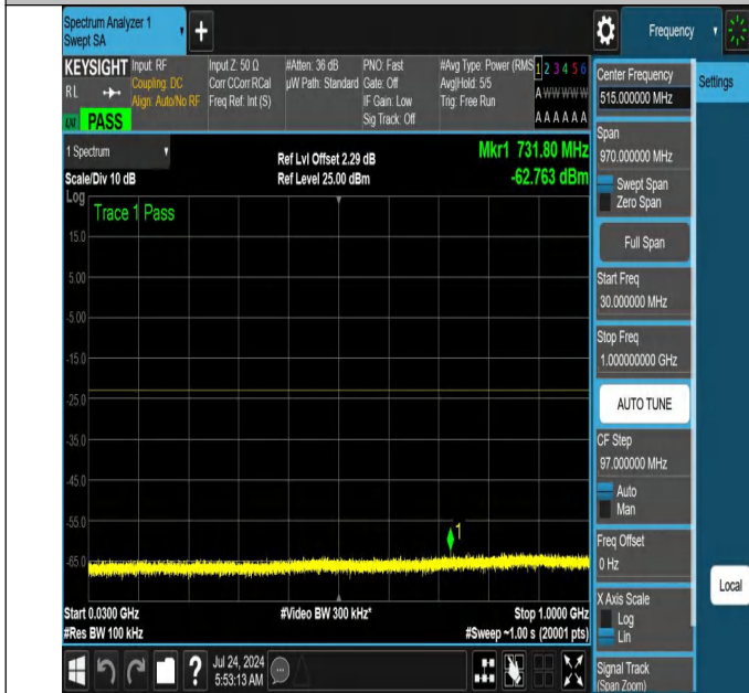
NTNV-N66-PC3-15-40-H-DFT-QPSK-Edge_1RB_Left-30-1000-A nt1-PASS
