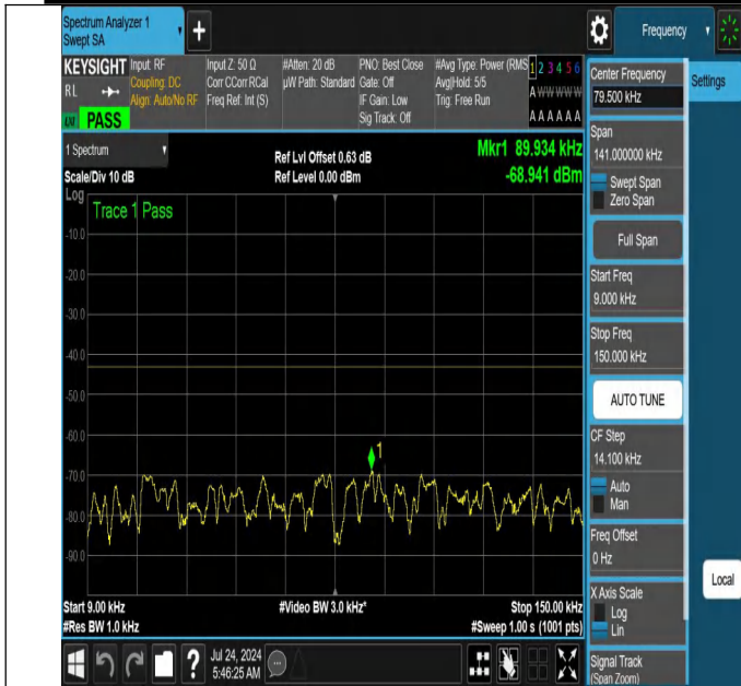
NTNV-N66-PC3-15-40-M-DFT-QPSK-Edge_1RB_Left-0.009-0.15 -Ant1-PASS
