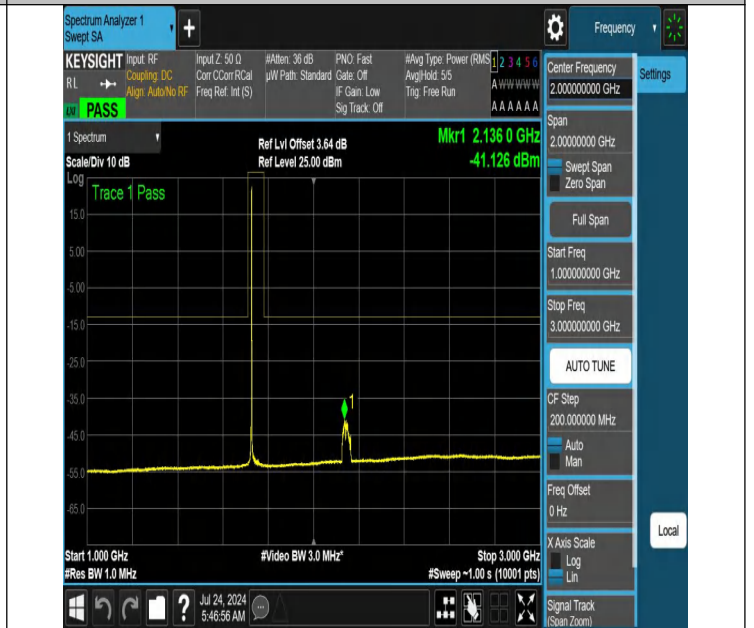
NTNV-N66-PC3-15-40-M-DFT-QPSK-Edge_1RB_Left-1000-3000-Ant1-PASS
