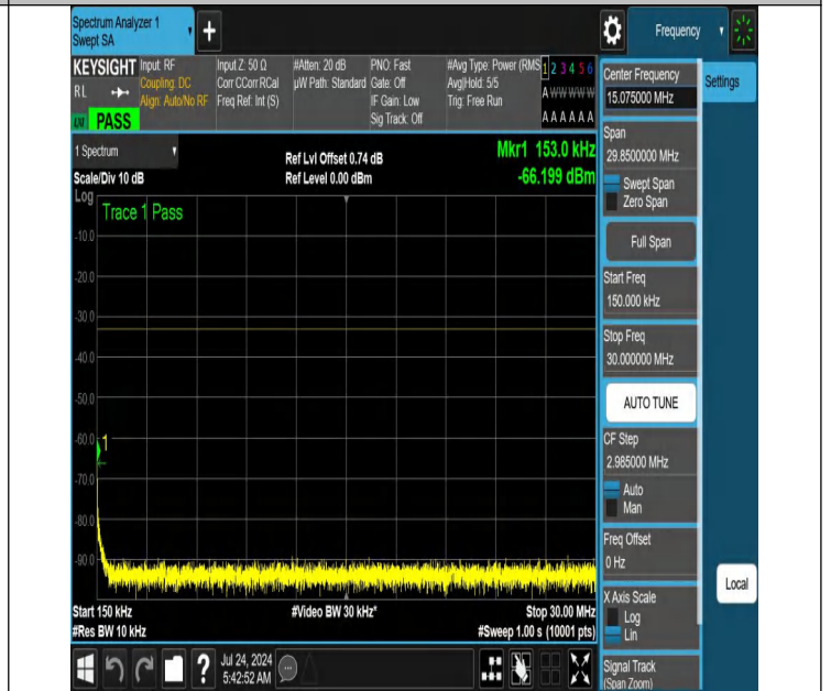
NTNV-N66-PC3-15-40-L-DFT-QPSK-Edge_1RB_Right-0.15-30-A nt1-PASS
