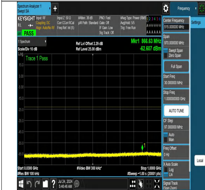
NTNV-N66-PC3-15-40-M-DFT-QPSK-Edge_1RB_Left-30-1000-Ant1-PASS
