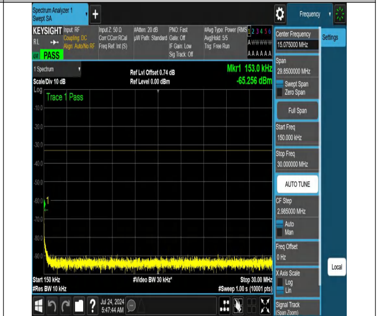
NTNV-N66-PC3-15-40-M-DFT-QPSK-Edge_1RB_Right-0.15-30-A nt1-PASS
