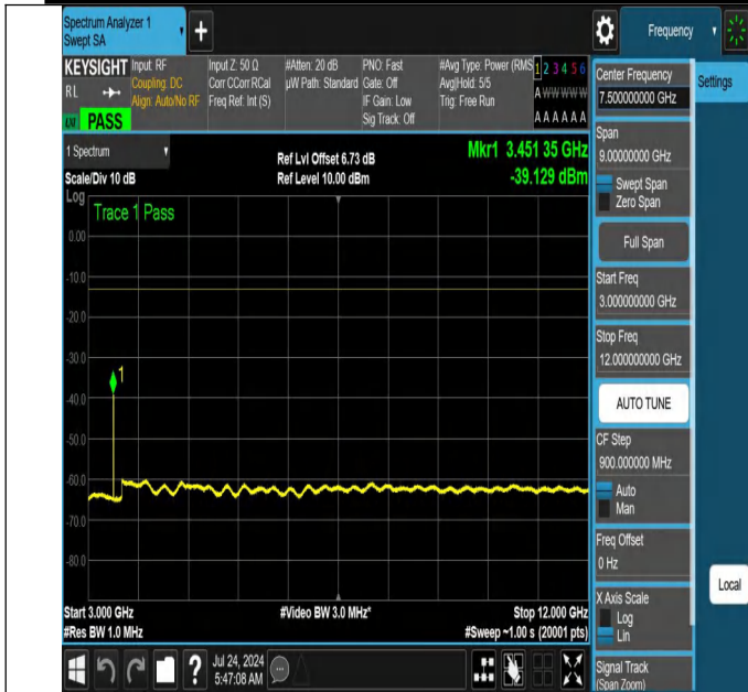
NTNV-N66-PC3-15-40-M-DFT-QPSK-Edge_1RB_Left-3000-1200 0-Ant1-PASS
