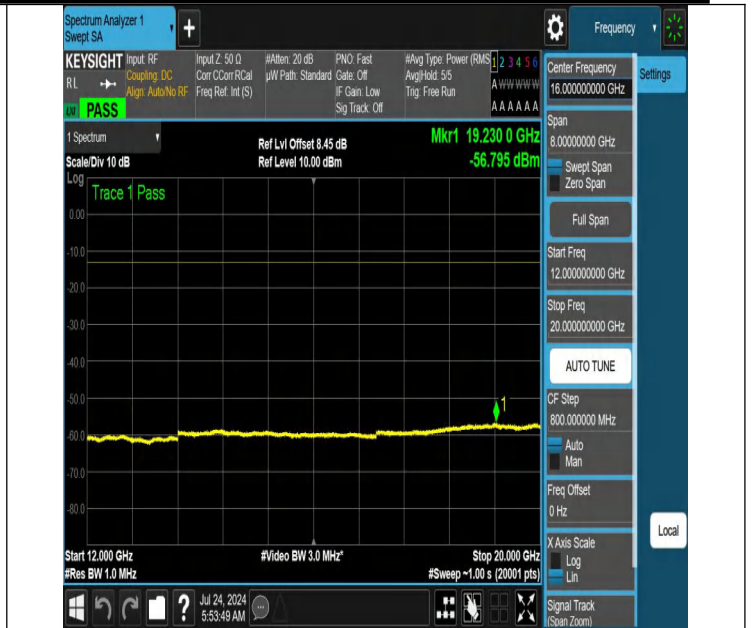
NTNV-N66-PC3-15-40-H-DFT-QPSK-Edge_1RB_Left-12000-2000 0-Ant1-PASS
