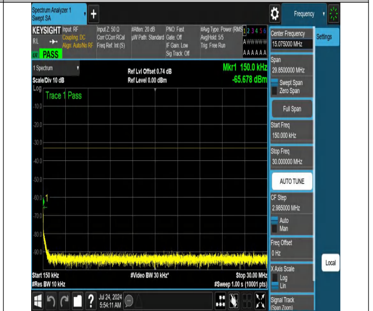
NTNV-N66-PC3-15-40-H-DFT-QPSK-Edge_1RB_Right-0.15-30-A nt1-PASS
