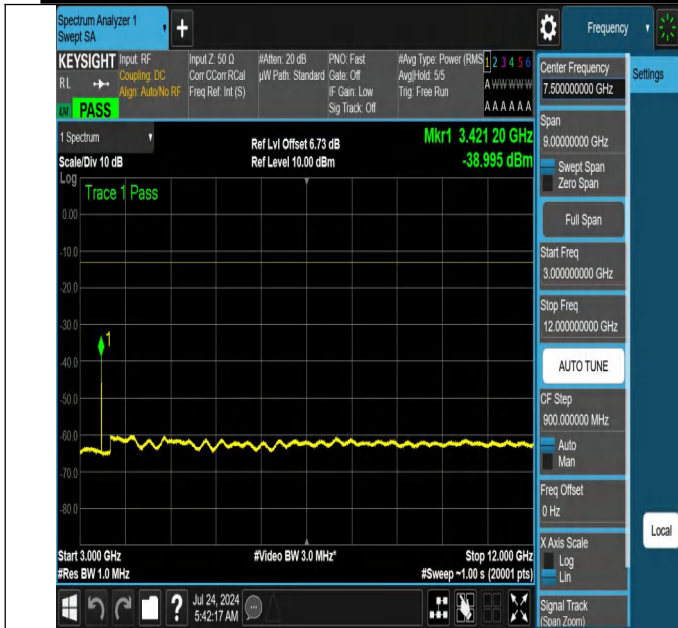
NTNV-N66-PC3-15-40-L-DFT-QPSK-Edge_1RB_Left-3000-1200 0-Ant1-PASS
