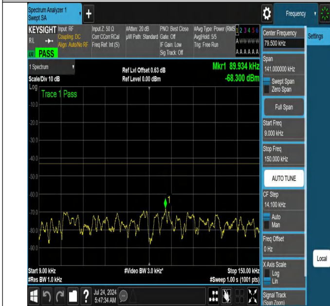
NTNV-N66-PC3-15-40-M-DFT-QPSK-Edge_1RB_Right-0.009-0. 15-Ant1-PASS
