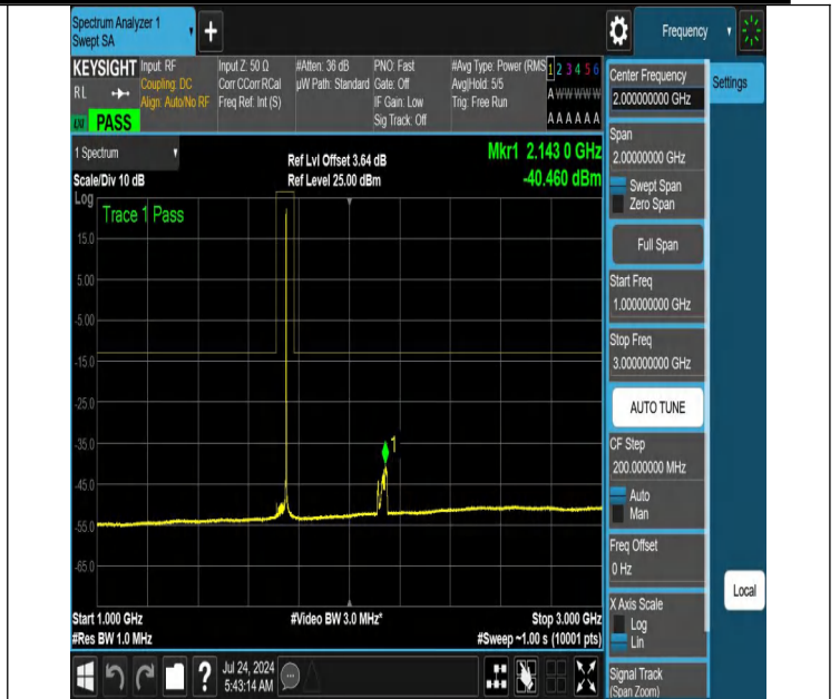
NTNV-N66-PC3-15-40-L-DFT-QPSK-Edge_1RB_Right-1000-3000-Ant1-PASS
