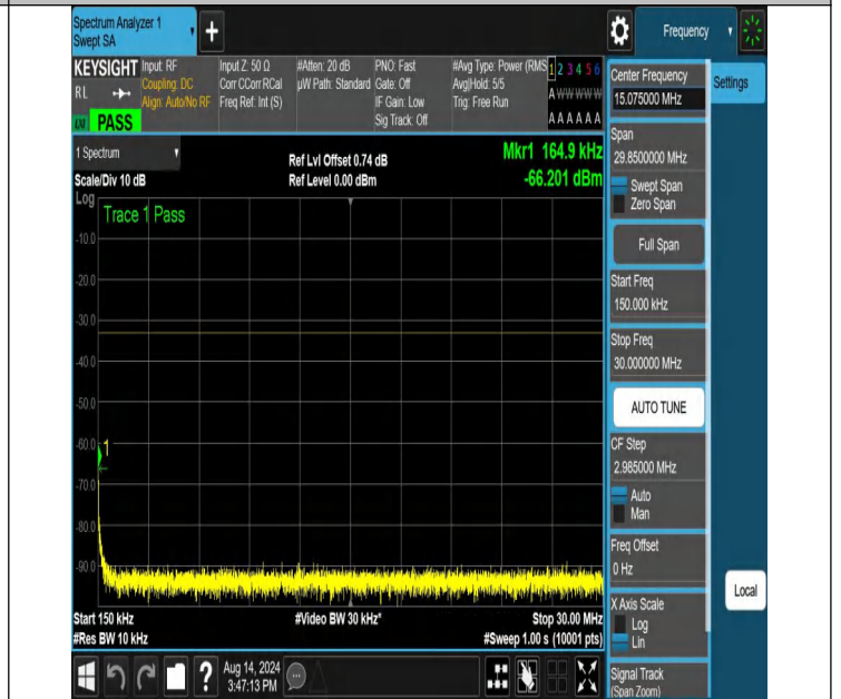
NTNV-N66-PC3-15-30-M-DFT-QPSK-Edge_1RB_Right-0.15-30-A nt1-PASS
