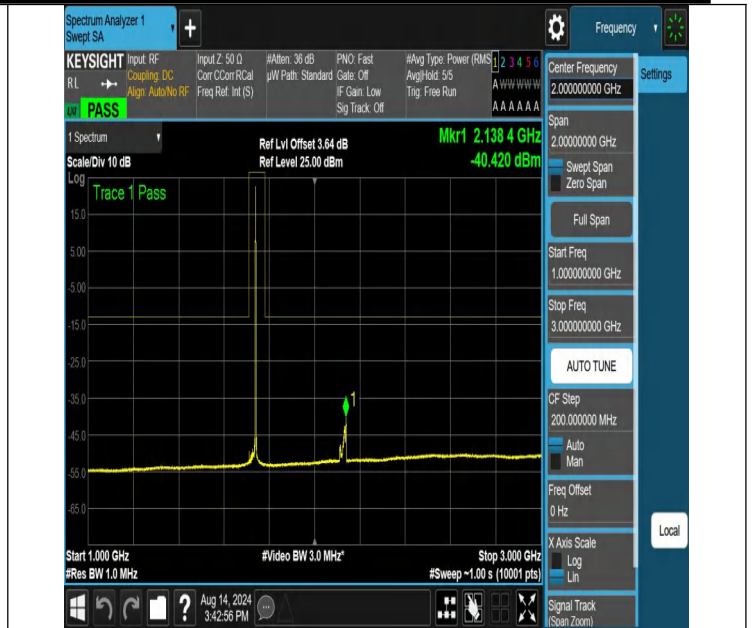
NTNV-N66-PC3-15-30-L-DFT-QPSK-Edge_1RB_Right-1000-3000-Ant1-PASS
