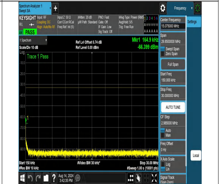
NTNV-N66-PC3-15-30-L-DFT-QPSK-Edge_1RB_Right-0.15-30-A nt1-PASS
