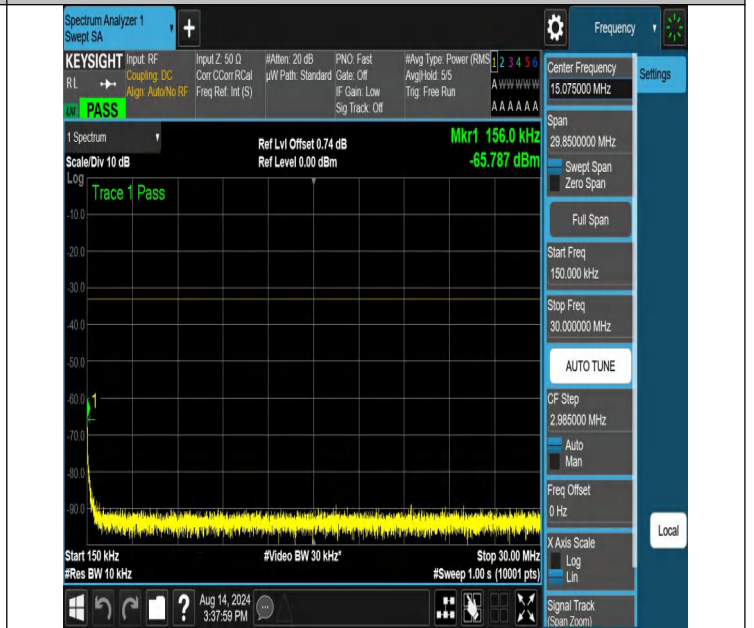
NTNV-N66-PC3-15-25-H-DFT-QPSK-Edge_1RB_Right-0.15-30-A nt1-PASS
