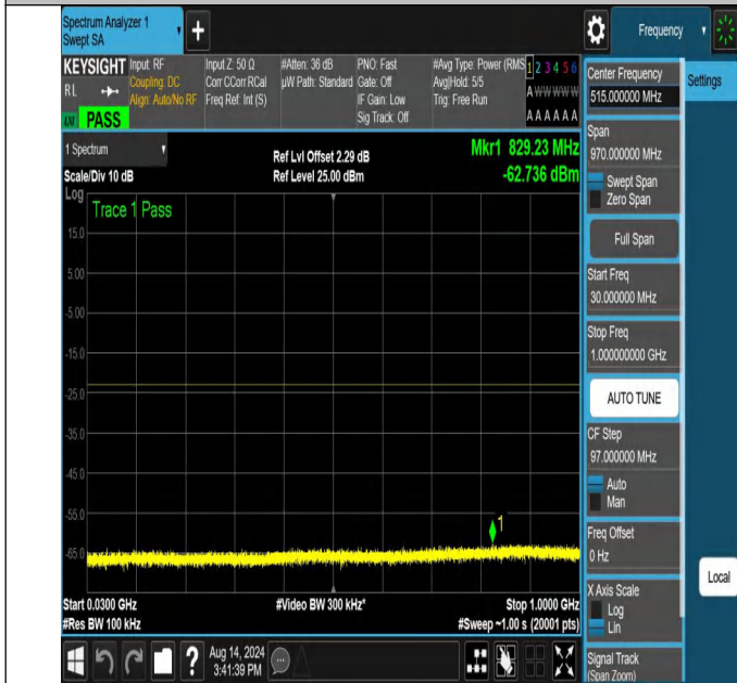
NTNV-N66-PC3-15-30-L-DFT-QPSK-Edge_1RB_Left-30-1000-A nt1-PASS
