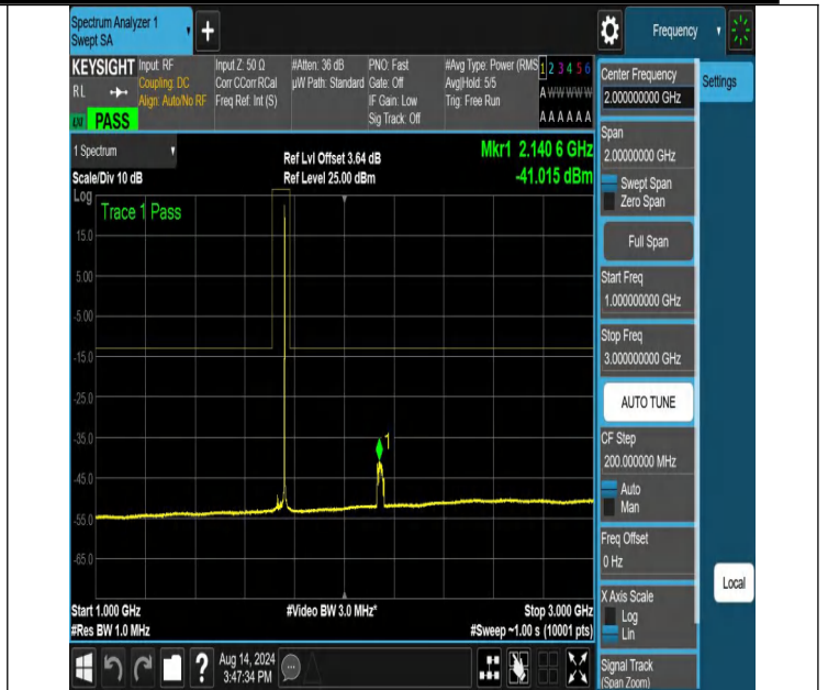
NTNV-N66-PC3-15-30-M-DFT-QPSK-Edge_1RB_Right-1000-300-0-Ant1-PASS
