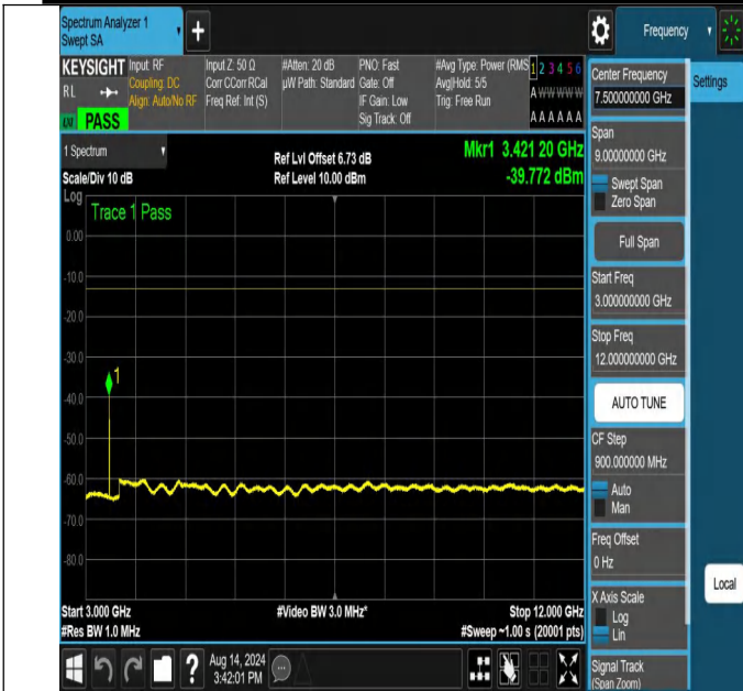
NTNV-N66-PC3-15-30-L-DFT-QPSK-Edge_1RB_Left-3000-1200 0-Ant1-PASS
