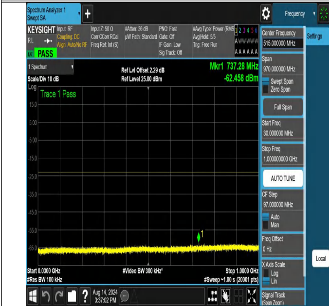
NTNV-N66-PC3-15-25-H-DFT-QPSK-Edge_1RB_Left-30-1000-A nt1-PASS
