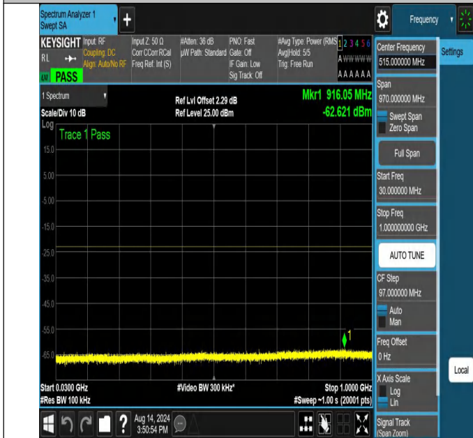
NTNV-N66-PC3-15-30-H-DFT-QPSK-Edge_1RB_Left-30-1000-A nt1-PASS
