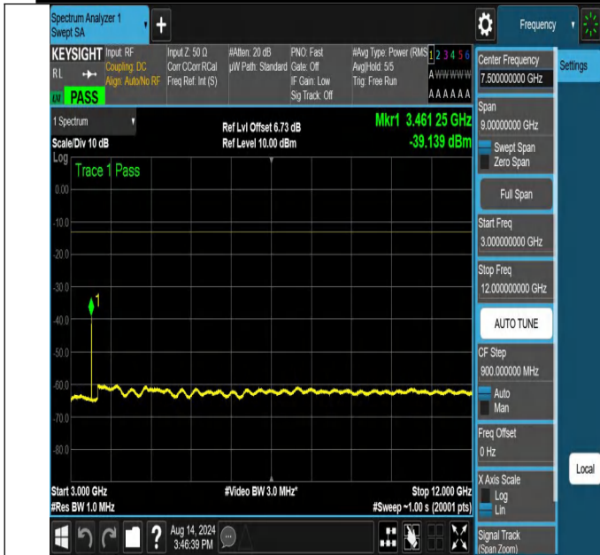
NTNV-N66-PC3-15-30-M-DFT-QPSK-Edge_1RB_Left-3000-1200 0-Ant1-PASS
