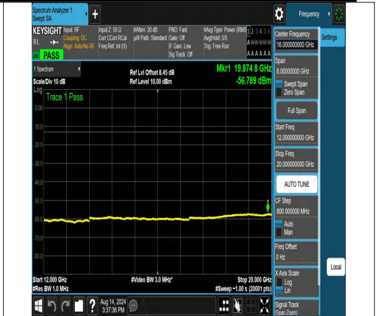
NTNV-N66-PC3-15-25-H-DFT-QPSK-Edge_1RB_Left-12000-2000 0-Ant1-PASS
