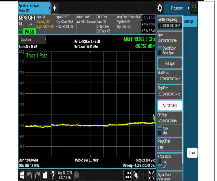
NTNV-N66-PC3-15-30-L-DFT-QPSK-Edge_1RB_Left-12000-2000 0-Ant1-PASS
