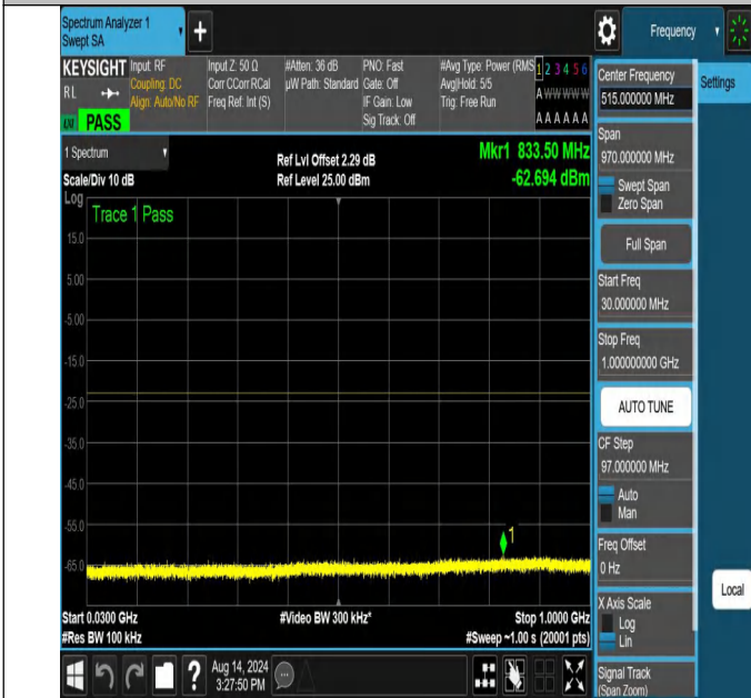
NTNV-N66-PC3-15-25-L-DFT-QPSK-Edge_1RB_Left-30-1000-Ant1-PASS
