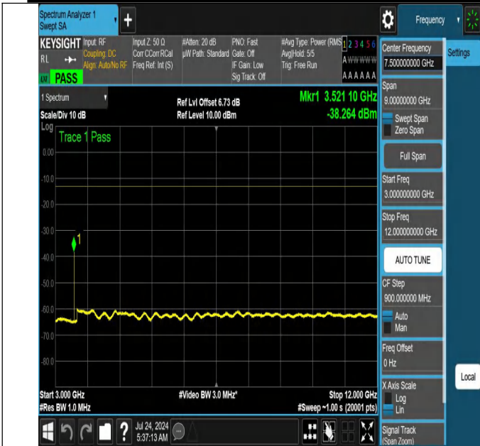
NTNV-N66-PC3-15-20-H-DFT-QPSK-Edge_1RB_Left-3000-1200 0-Ant1-PASS
