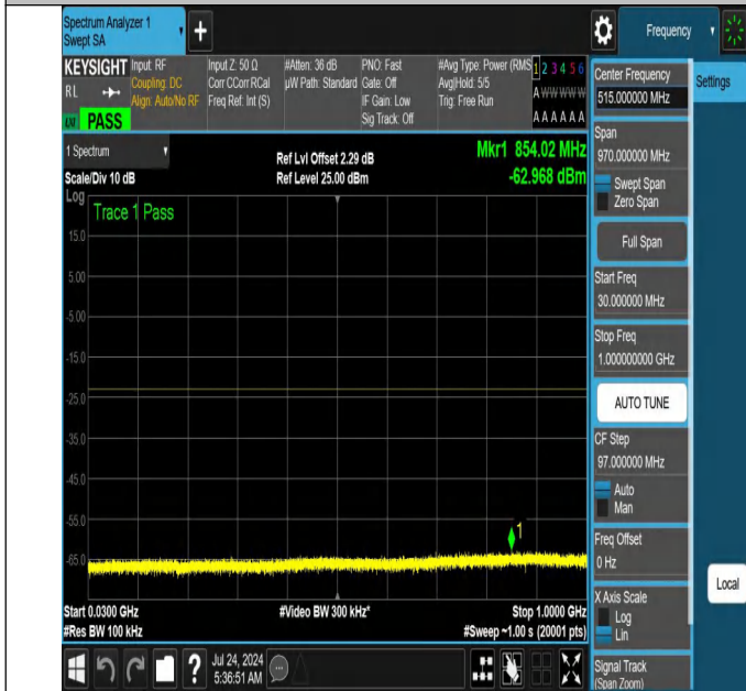
NTNV-N66-PC3-15-20-H-DFT-QPSK-Edge_1RB_Left-30-1000-A nt1-PASS
