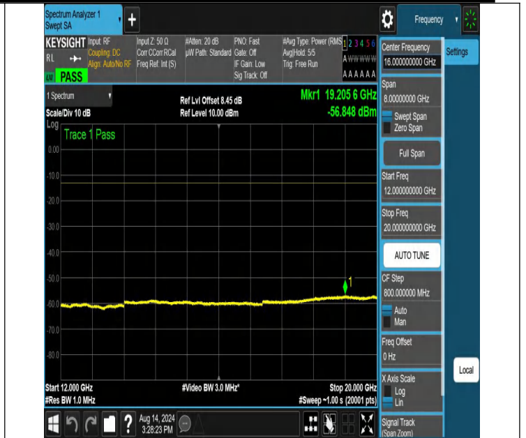
NTNV-N66-PC3-15-25-L-DFT-QPSK-Edge_1RB_Left-12000-2000 0-Ant1-PASS
