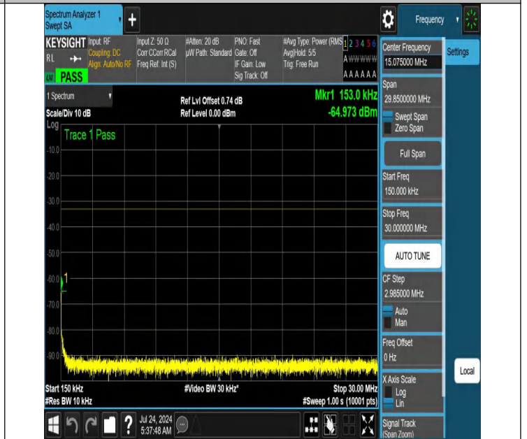
NTNV-N66-PC3-15-20-H-DFT-QPSK-Edge_1RB_Right-0.15-30-A nt1-PASS
