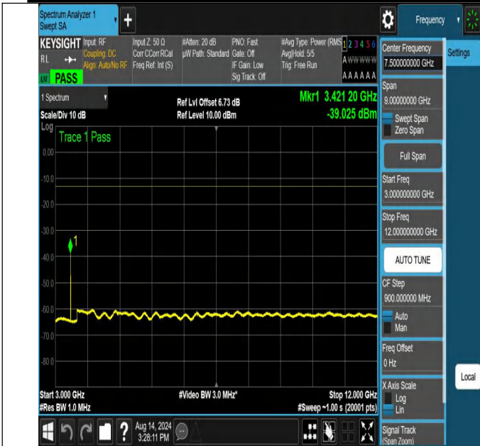
NTNV-N66-PC3-15-25-L-DFT-QPSK-Edge_1RB_Left-3000-1200 0-Ant1-PASS
