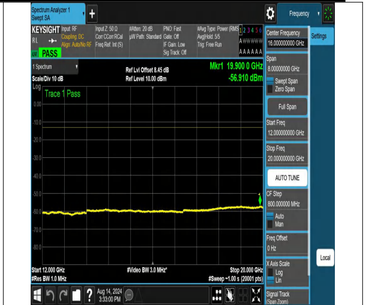
NTNV-N66-PC3-15-25-M-DFT-QPSK-Edge_1RB_Left-12000-200 00-Ant1-PASS
