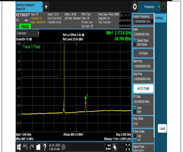
NTNV-N66-PC3-15-20-H-DFT-QPSK-Edge_1RB_Right-1000-300-0-Ant1-PASS
