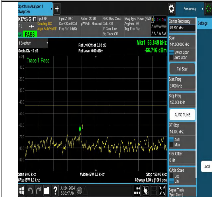
NTNV-N66-PC3-15-20-H-DFT-PI2BPSK-Edge_1RB_Right-0.009- 0.15-Ant1-PASS
