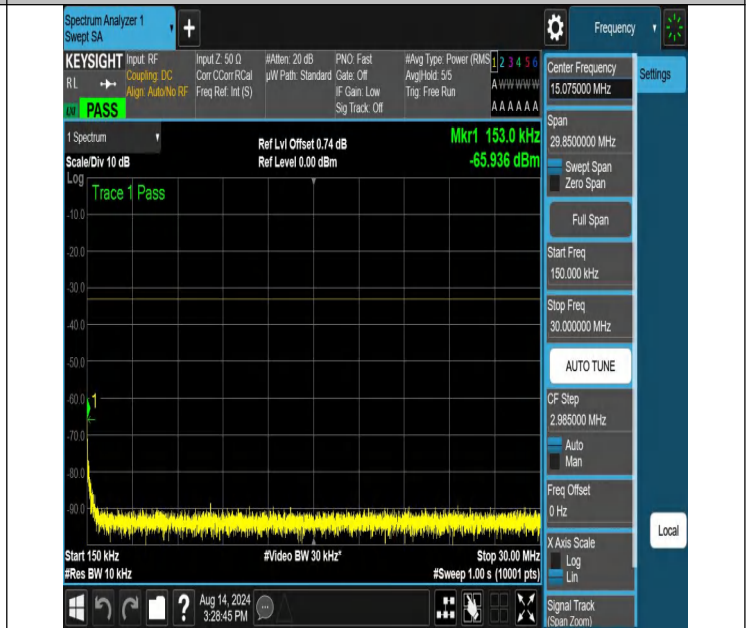
NTNV-N66-PC3-15-25-L-DFT-QPSK-Edge_1RB_Right-0.15-30-A nt1-PASS
