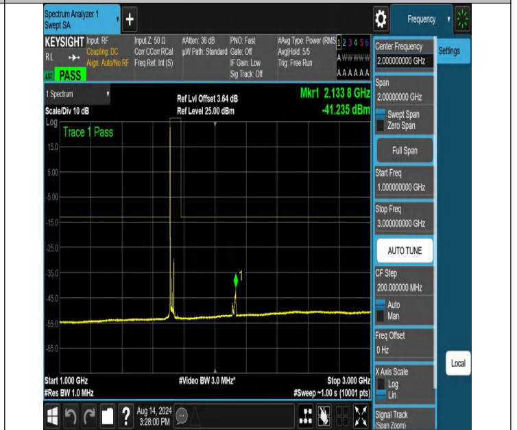
NTNV-N66-PC3-15-25-L-DFT-QPSK-Edge_1RB_Left-1000-3000-Ant1-PASS
