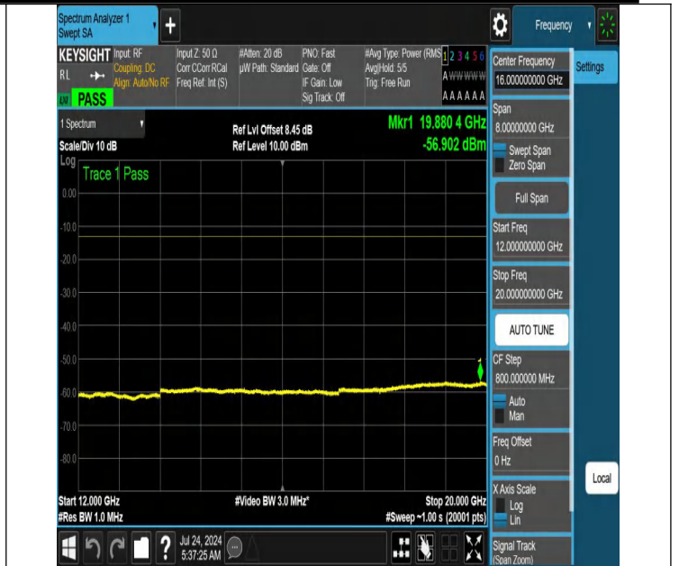
NTNV-N66-PC3-15-20-H-DFT-QPSK-Edge_1RB_Left-12000-2000 0-Ant1-PASS
