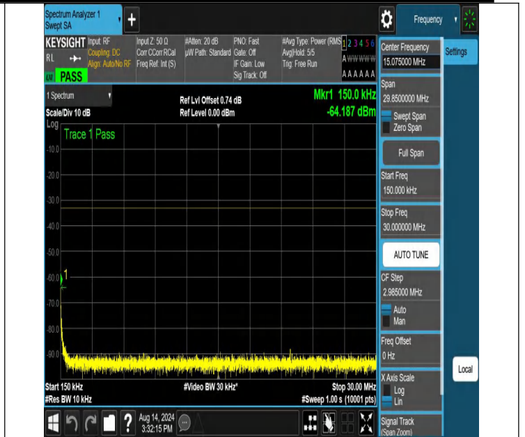
NTNV-N66-PC3-15-25-M-DFT-QPSK-Edge_1RB_Left-0.15-30-Ant 1-PASS
