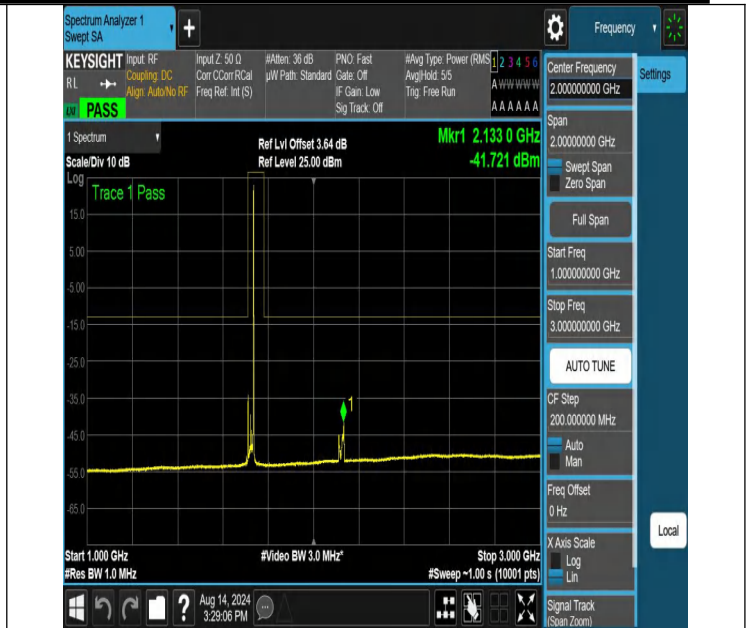
NTNV-N66-PC3-15-25-L-DFT-QPSK-Edge_1RB_Right-1000-3000-Ant1-PASS
