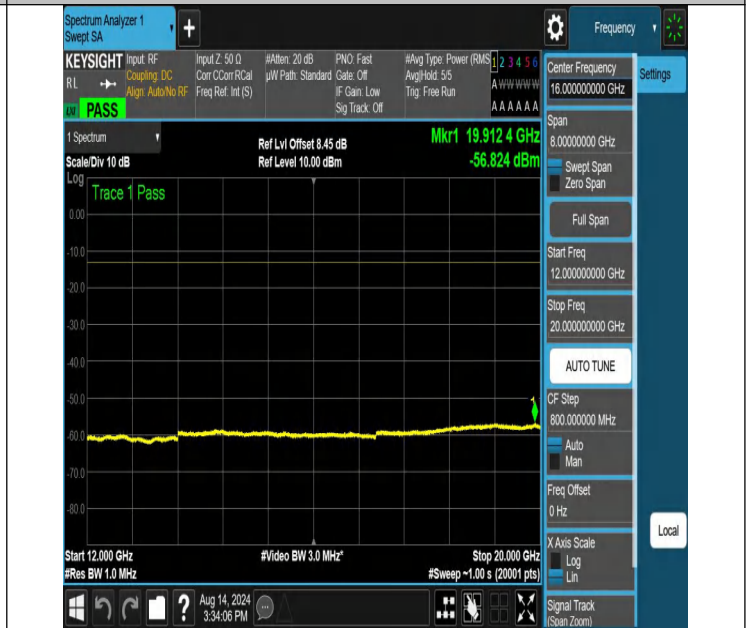
NTNV-N66-PC3-15-25-M-DFT-QPSK-Edge_1RB_Right-12000-20000-Ant1-PASS
