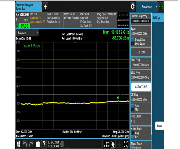
NTNV-N66-PC3-15-20-H-DFT-QPSK-Edge_1RB_Right-12000-20-000-Ant1-PASS
