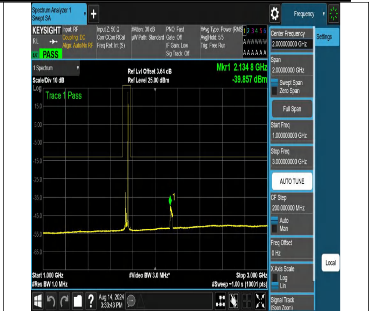
NTNV-N66-PC3-15-25-M-DFT-QPSK-Edge_1RB_Right-1000-300-0-Ant1-PASS
