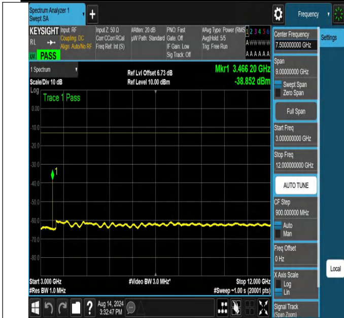
NTNV-N66-PC3-15-25-M-DFT-QPSK-Edge_1RB_Left-3000-1200 0-Ant1-PASS
