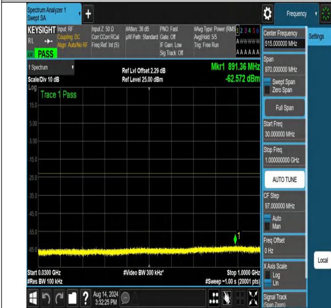
NTNV-N66-PC3-15-25-M-DFT-QPSK-Edge_1RB_Left-30-1000-A nt1-PASS
