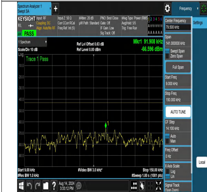
NTNV-N66-PC3-15-25-M-DFT-QPSK-Edge_1RB_Right-0.009-0. 15-Ant1-PASS
