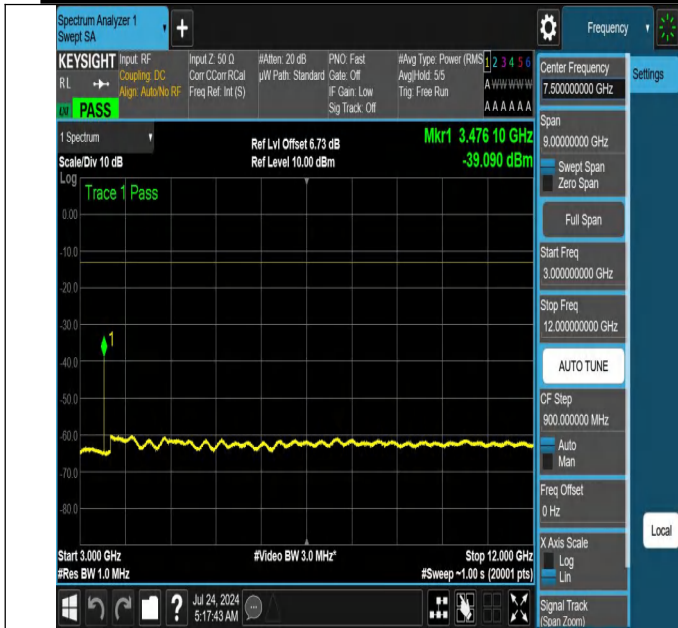
NTNV-N66-PC3-15-15-M-DFT-QPSK-Edge_1RB_Left-3000-1200 0-Ant1-PASS
