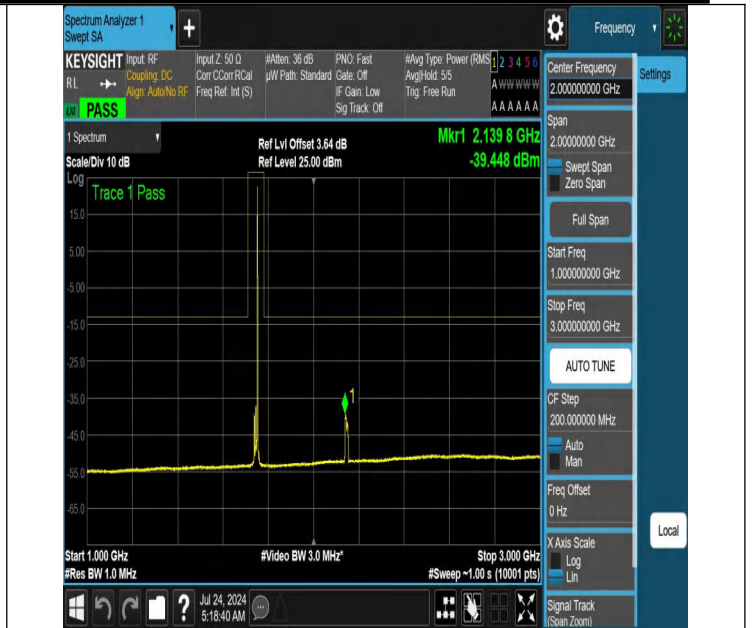
NTNV-N66-PC3-15-15-M-DFT-QPSK-Edge_1RB_Right-1000-300-0-Ant1-PASS
