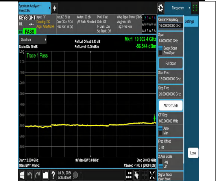
NTNV-N66-PC3-15-20-M-DFT-QPSK-Edge_1RB_Left-12000-200 00-Ant1-PASS
