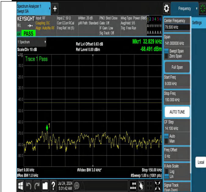
NTNV-N66-PC3-15-20-M-DFT-QPSK-Edge_1RB_Left-0.009-0.15 -Ant1-PASS
