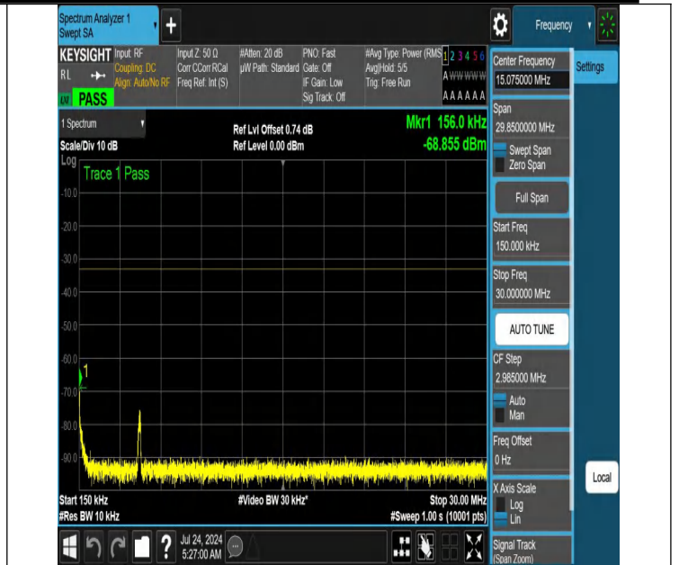
NTNV-N66-PC3-15-20-L-DFT-QPSK-Edge_1RB_Left-0.15-30-Ant 1-PASS
