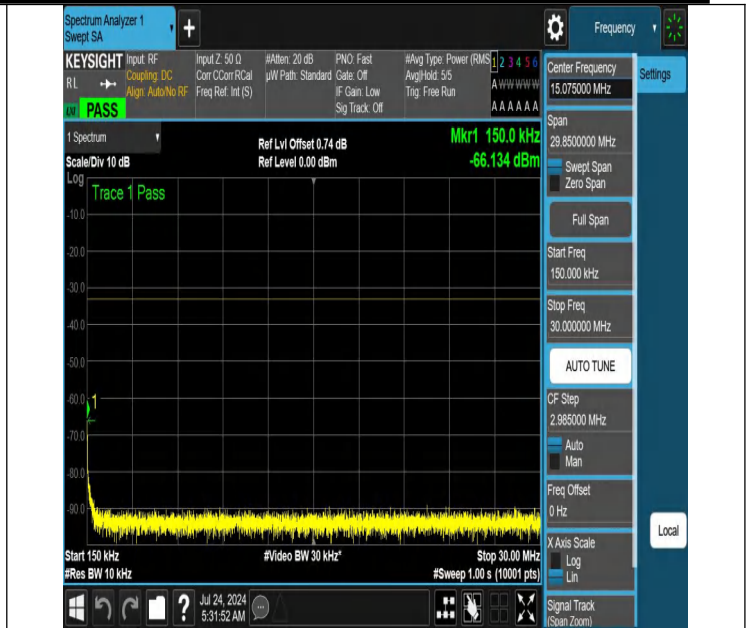
NTNV-N66-PC3-15-20-M-DFT-QPSK-Edge_1RB_Left-0.15-30-Ant 1-PASS
