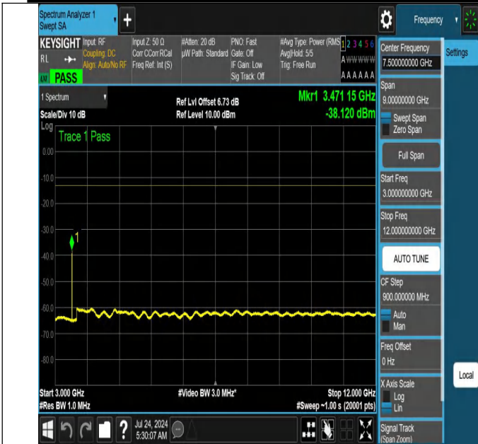
NTNV-N66-PC3-15-20-M-DFT-PI2BPSK-Edge_1RB_Left-3000-1 2000-Ant1-PASS
