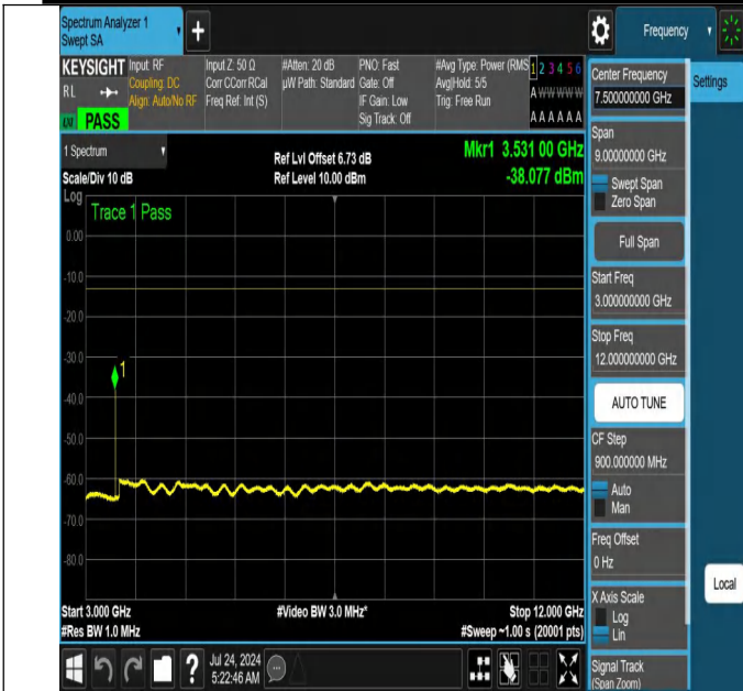
NTNV-N66-PC3-15-15-H-DFT-QPSK-Edge_1RB_Left-3000-1200 0-Ant1-PASS
