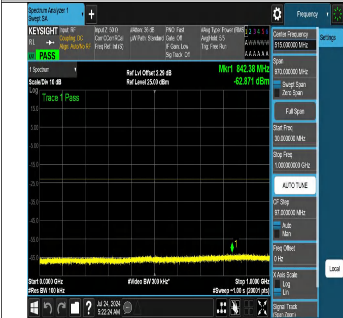
NTNV-N66-PC3-15-15-H-DFT-QPSK-Edge_1RB_Left-30-1000-A nt1-PASS
