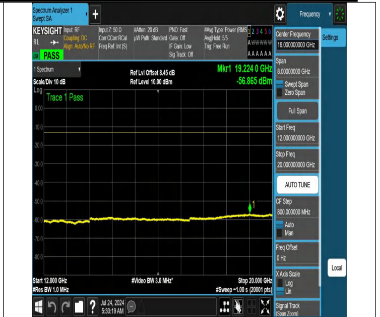
NTNV-N66-PC3-15-20-M-DFT-PI2BPSK-Edge_1RB_Left-12000-2 0000-Ant1-PASS
