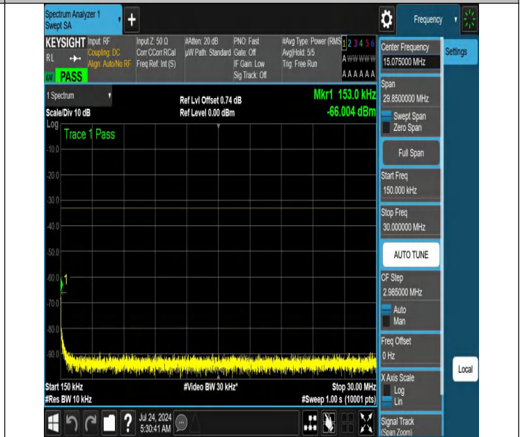
NTNV-N66-PC3-15-20-M-DFT-PI2BPSK-Edge_1RB_Right-0.15-3 0-Ant1-PASS
