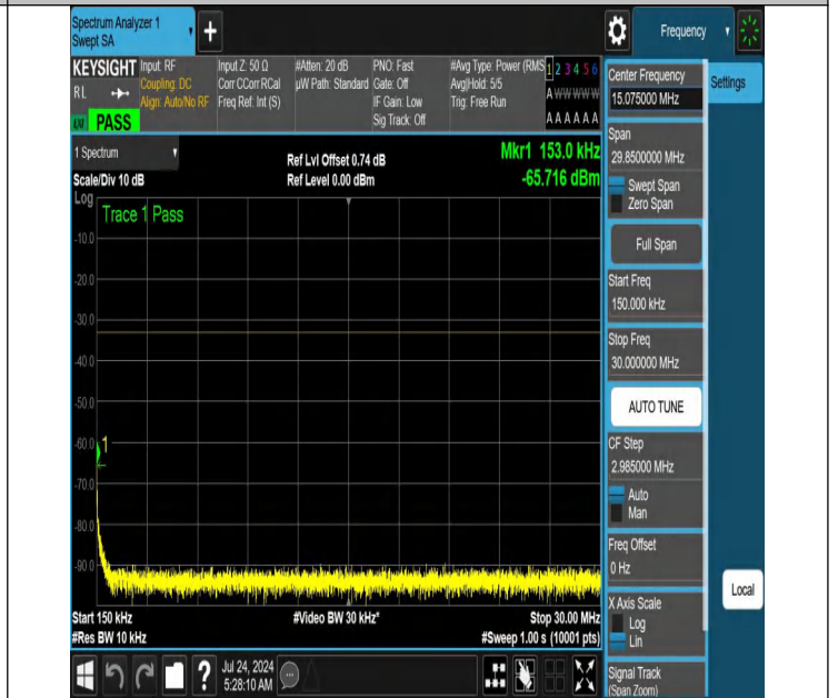
NTNV-N66-PC3-15-20-L-DFT-QPSK-Edge_1RB_Right-0.15-30-A nt1-PASS
