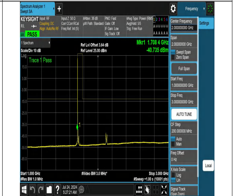
NTNV-N66-PC3-15-20-L-DFT-QPSK-Edge_1RB_Left-1000-3000-Ant1-PASS
