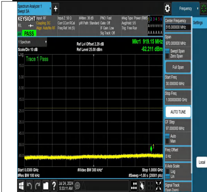
NTNV-N66-PC3-15-20-M-DFT-QPSK-Edge_1RB_Right-30-1000-Ant1-PASS
