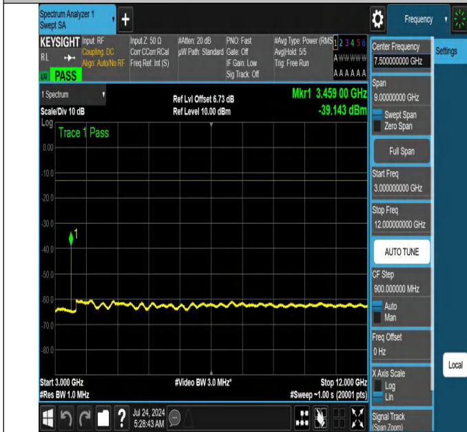
NTNV-N66-PC3-15-20-L-DFT-QPSK-Edge_1RB_Right-3000-12000-Ant1-PASS
