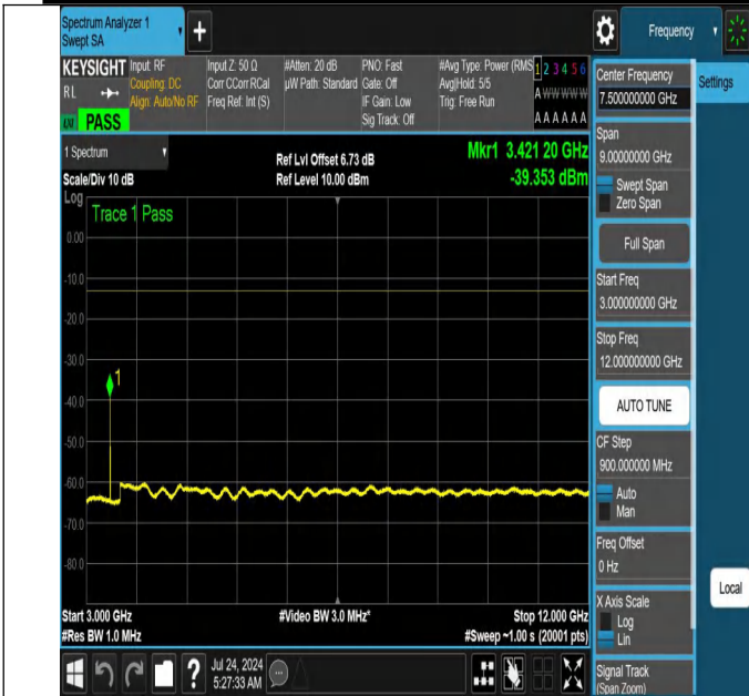
NTNV-N66-PC3-15-20-L-DFT-QPSK-Edge_1RB_Left-3000-1200 0-Ant1-PASS
