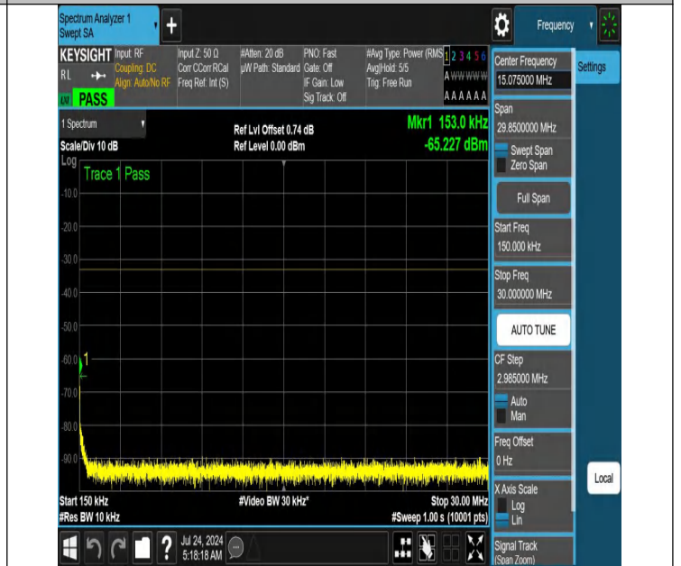
NTNV-N66-PC3-15-15-M-DFT-QPSK-Edge_1RB_Right-0.15-30-A nt1-PASS
