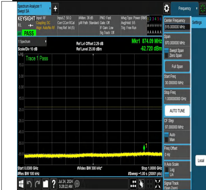
NTNV-N66-PC3-15-20-L-DFT-QPSK-Edge_1RB_Right-30-1000-Ant1-PASS
