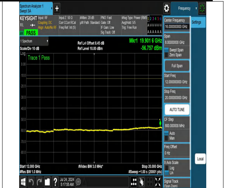
NTNV-N66-PC3-15-15-M-DFT-QPSK-Edge_1RB_Left-12000-200 00-Ant1-PASS
