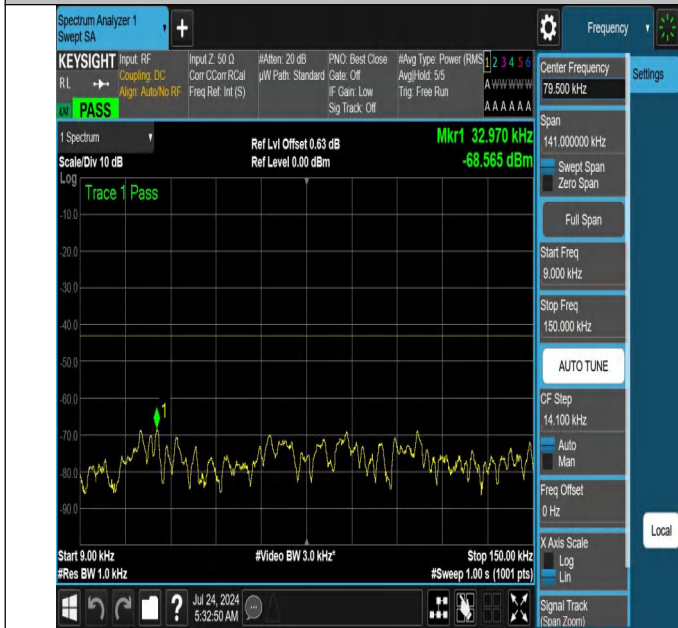
NTNV-N66-PC3-15-20-M-DFT-QPSK-Edge_1RB_Right-0.009-0. 15-Ant1-PASS
