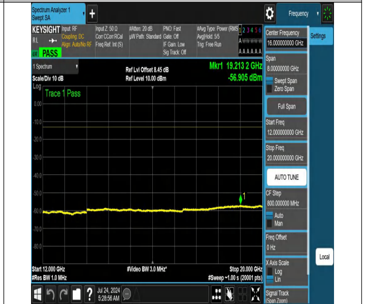
NTNV-N66-PC3-15-20-L-DFT-QPSK-Edge_1RB_Right-12000-20000-Ant1-PASS
