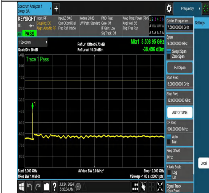
NTNV-N66-PC3-15-20-M-DFT-QPSK-Edge_1RB_Right-3000-12000-Ant1-PASS
