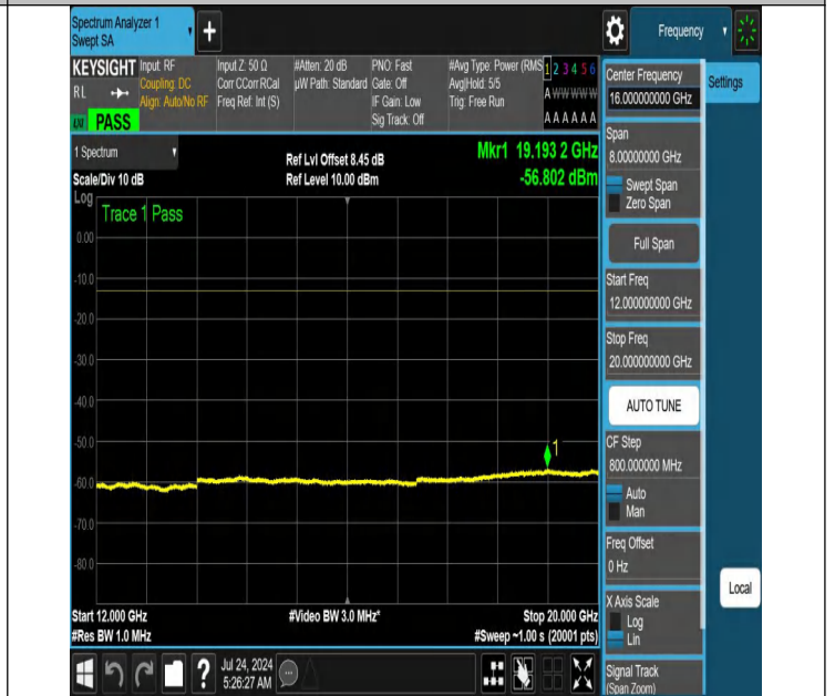
NTNV-N66-PC3-15-20-L-DFT-PI2BPSK-Edge_1RB_Right-12000-20000-Ant1-PASS
