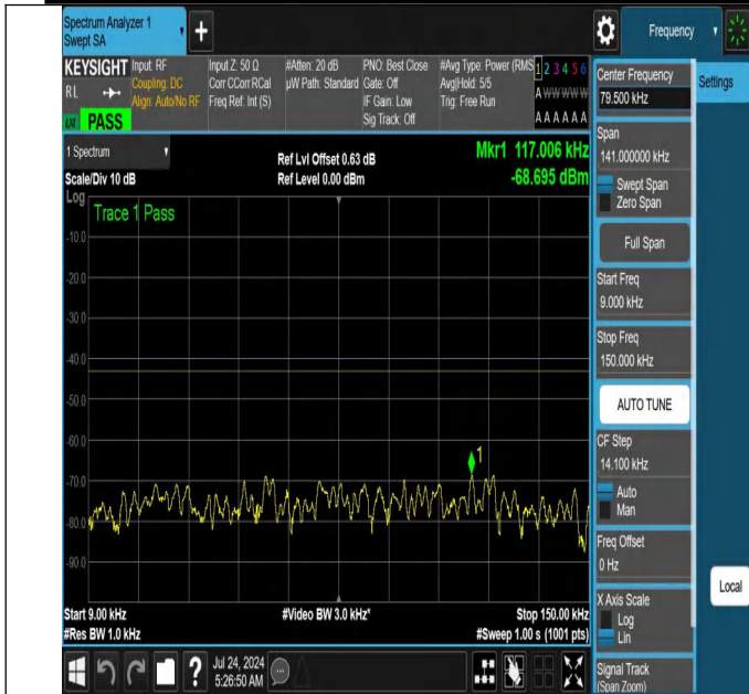
NTNV-N66-PC3-15-20-L-DFT-QPSK-Edge_1RB_Left-0.009-0.15-Ant1-PASS
