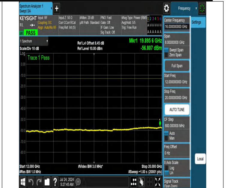
NTNV-N66-PC3-15-20-L-DFT-QPSK-Edge_1RB_Left-12000-2000 0-Ant1-PASS
