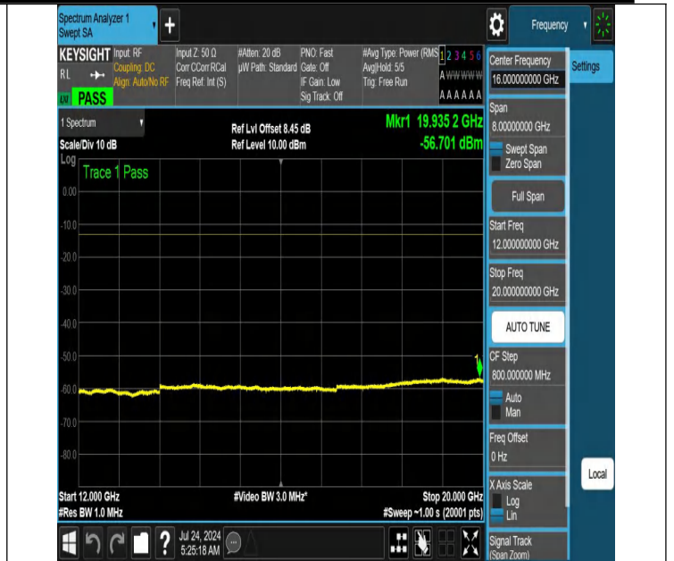
NTNV-N66-PC3-15-20-L-DFT-PI2BPSK-Edge_1RB_Left-12000-20000-Ant1-PASS
