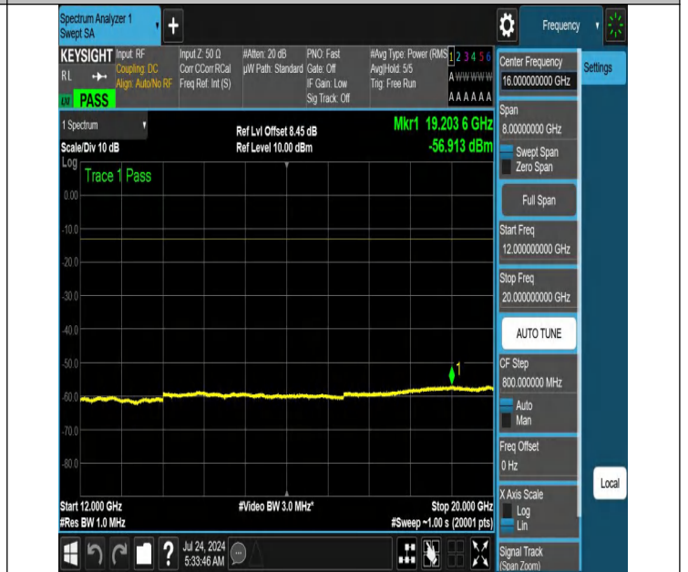
NTNV-N66-PC3-15-20-M-DFT-QPSK-Edge_1RB_Right-12000-20000-Ant1-PASS
