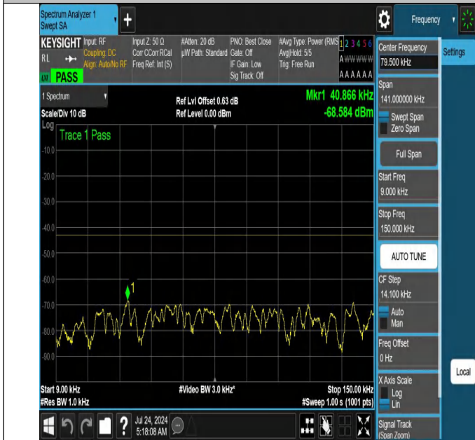
NTNV-N66-PC3-15-15-M-DFT-QPSK-Edge_1RB_Right-0.009-0. 15-Ant1-PASS
