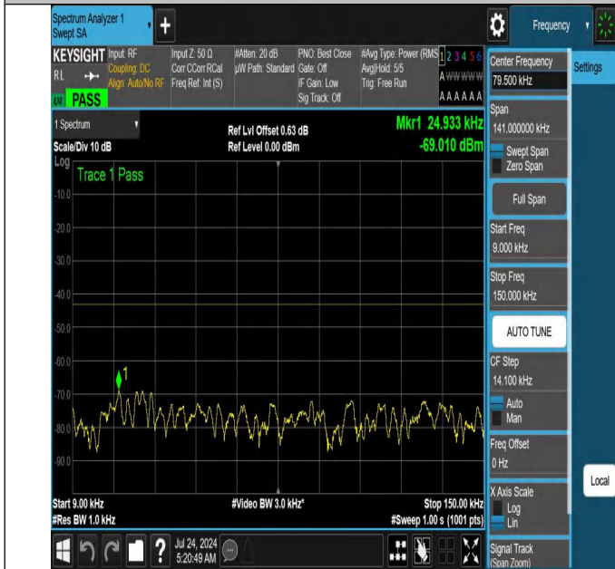
NTNV-N66-PC3-15-15-H-DFT-PI2BPSK-Edge_1RB_Right-0.009- 0.15-Ant1-PASS
