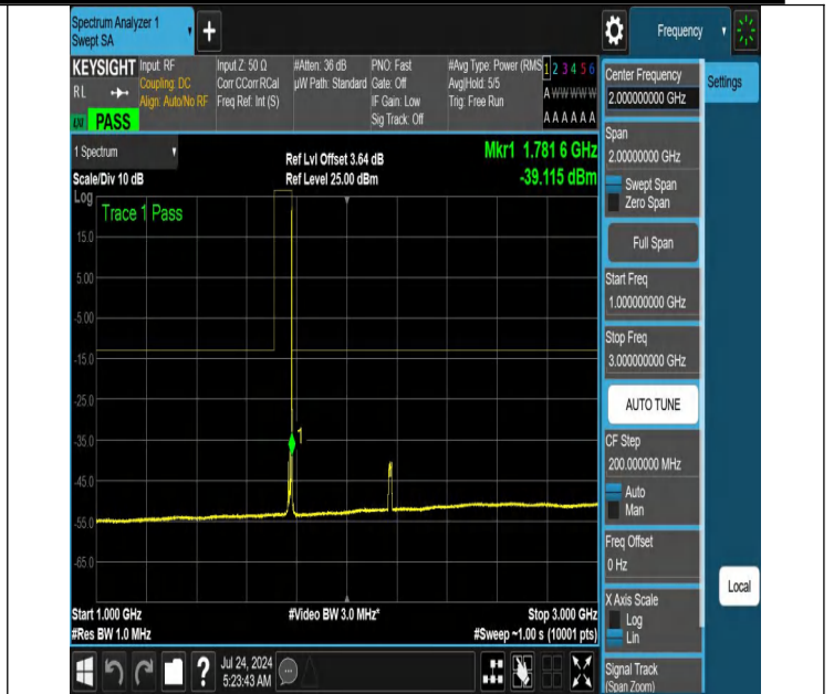
NTNV-N66-PC3-15-15-H-DFT-QPSK-Edge_1RB_Right-1000-300-0-Ant1-PASS
