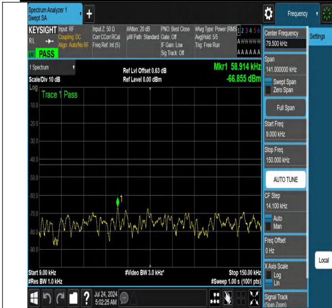
NTNV-N66-PC3-15-10-M-DFT-QPSK-Edge_1RB_Left-0.009-0.15 -Ant1-PASS
