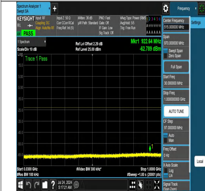
NTNV-N66-PC3-15-15-M-DFT-QPSK-Edge_1RB_Left-30-1000-A nt1-PASS
