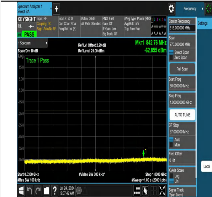
NTNV-N66-PC3-15-10-H-DFT-QPSK-Edge_1RB_Left-30-1000-A nt1-PASS
