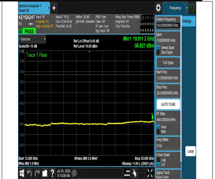
NTNV-N66-PC3-15-15-L-DFT-QPSK-Edge_1RB_Left-12000-2000 0-Ant1-PASS
