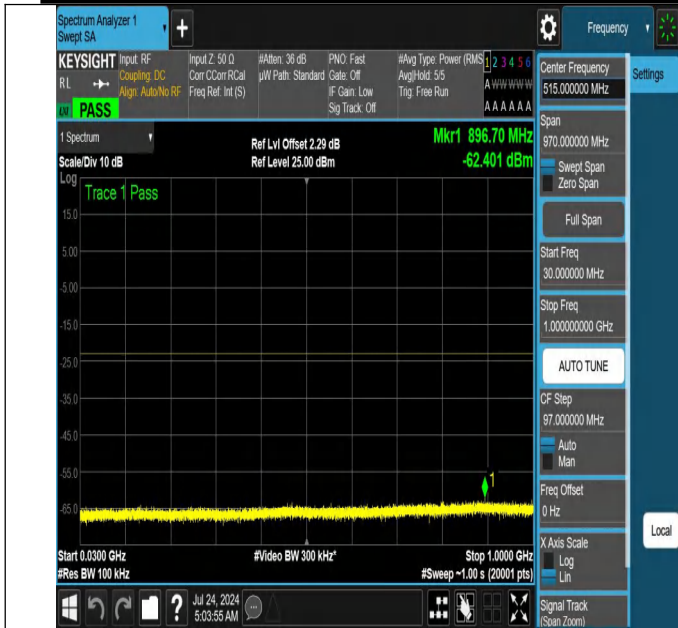
NTNV-N66-PC3-15-10-M-DFT-QPSK-Edge_1RB_Right-30-1000-Ant1-PASS
