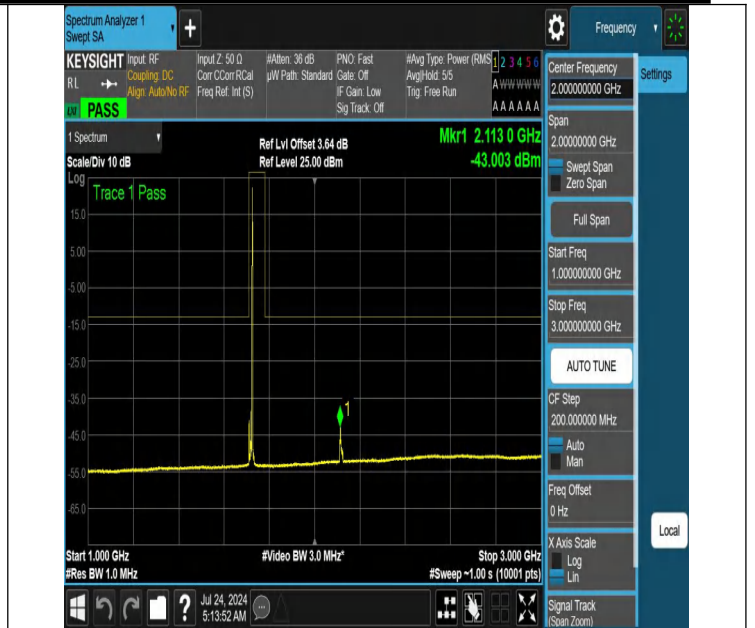
NTNV-N66-PC3-15-15-L-DFT-QPSK-Edge_1RB_Right-1000-3000-Ant1-PASS
