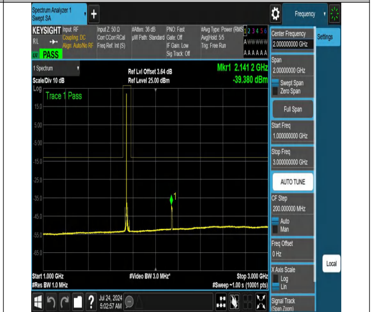
NTNV-N66-PC3-15-10-M-DFT-QPSK-Edge_1RB_Left-1000-3000-Ant1-PASS
