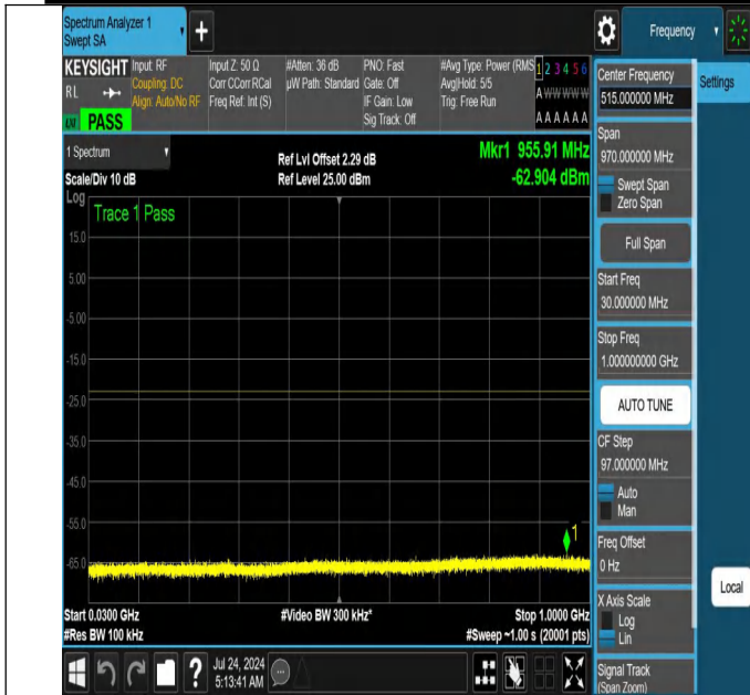
NTNV-N66-PC3-15-15-L-DFT-QPSK-Edge_1RB_Right-30-1000-Ant1-PASS
