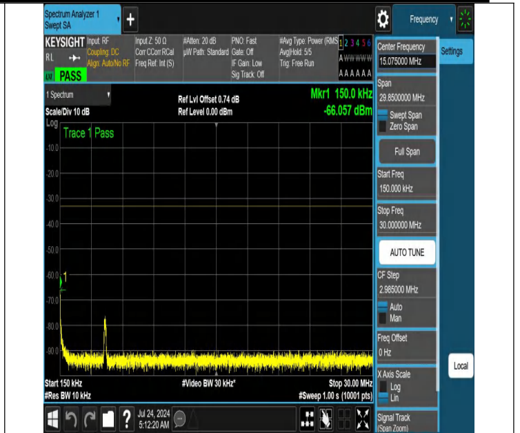
NTNV-N66-PC3-15-15-L-DFT-QPSK-Edge_1RB_Left-0.15-30-Ant 1-PASS
