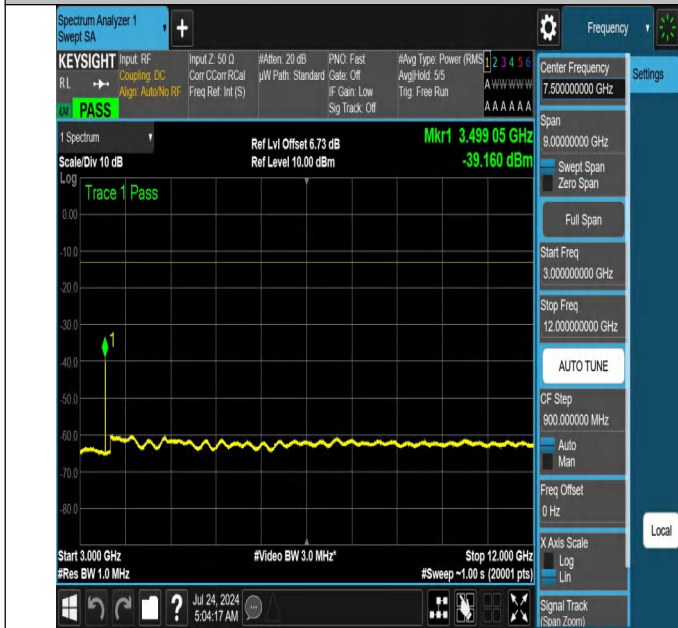
NTNV-N66-PC3-15-10-M-DFT-QPSK-Edge_1RB_Right-3000-12000-Ant1-PASS
