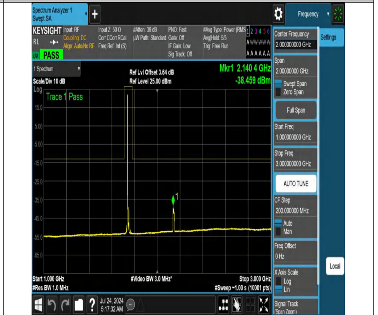
NTNV-N66-PC3-15-15-M-DFT-QPSK-Edge_1RB_Left-1000-3000-Ant1-PASS
