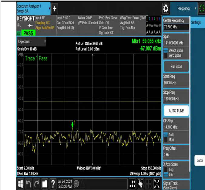
NTNV-N66-PC3-15-10-M-DFT-QPSK-Edge_1RB_Right-0.009-0. 15-Ant1-PASS
