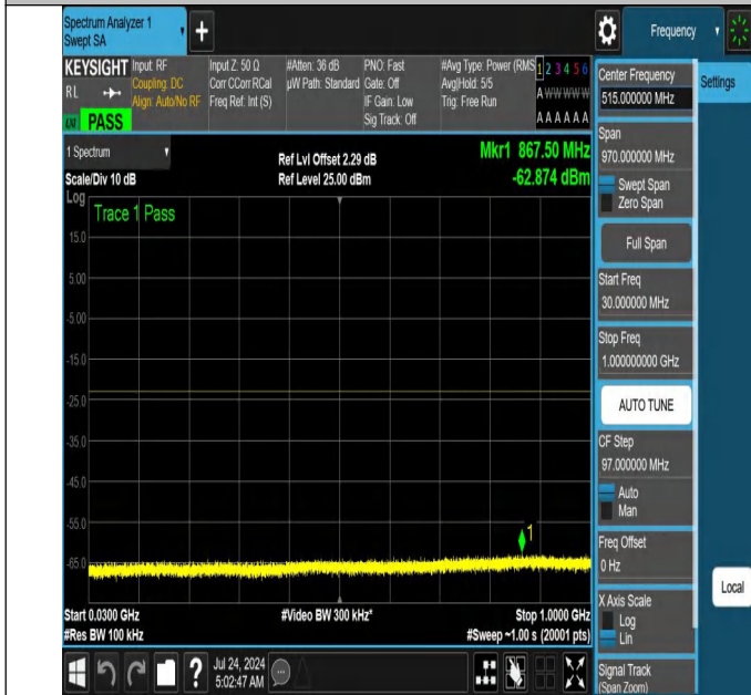
NTNV-N66-PC3-15-10-M-DFT-QPSK-Edge_1RB_Left-30-1000-A nt1-PASS
