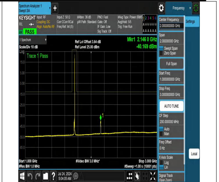
NTNV-N66-PC3-15-10-M-DFT-QPSK-Edge_1RB_Right-1000-300-0-Ant1-PASS
