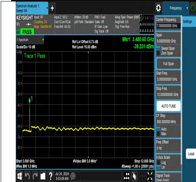
NTNV-N66-PC3-15-10-M-DFT-QPSK-Edge_1RB_Left-3000-1200 0-Ant1-PASS
