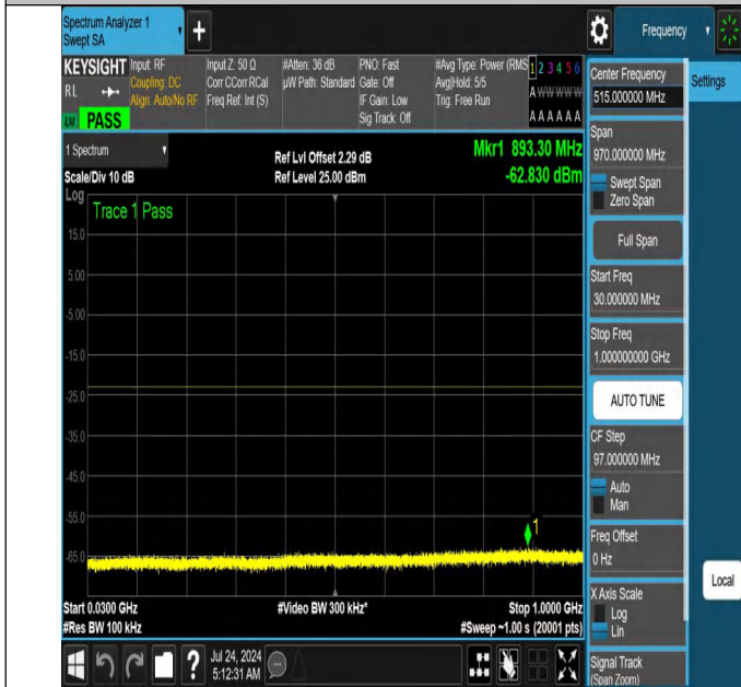
NTNV-N66-PC3-15-15-L-DFT-QPSK-Edge_1RB_Left-30-1000-Ant1-PASS
