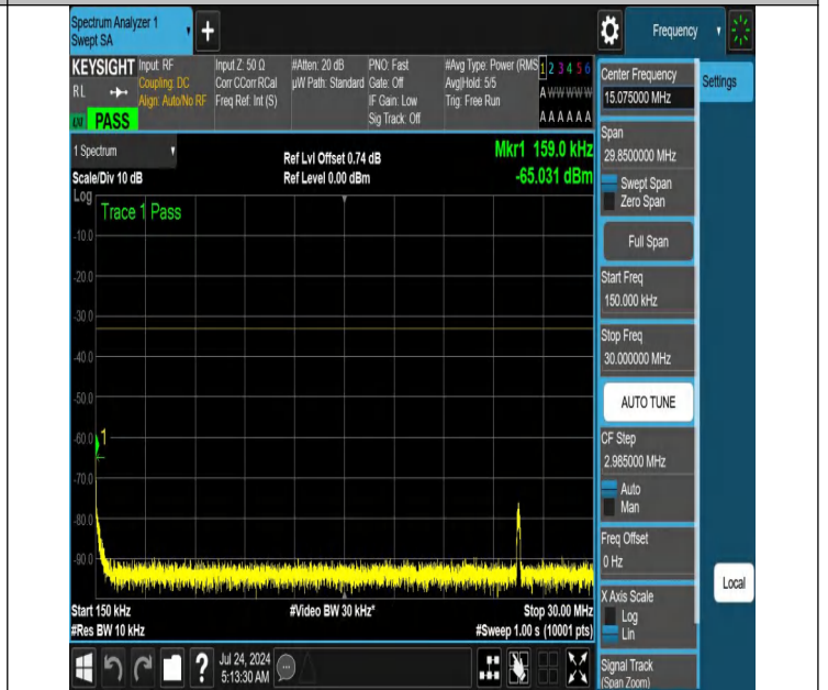
NTNV-N66-PC3-15-15-L-DFT-QPSK-Edge_1RB_Right-0.15-30-A nt1-PASS
