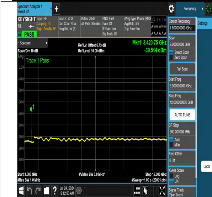
NTNV-N66-PC3-15-15-L-DFT-QPSK-Edge_1RB_Left-3000-1200 0-Ant1-PASS
