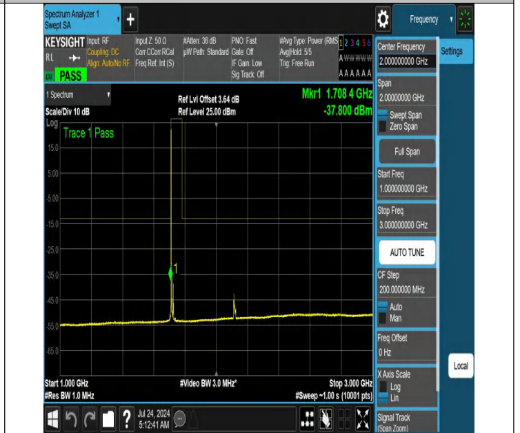
NTNV-N66-PC3-15-15-L-DFT-QPSK-Edge_1RB_Left-1000-3000-Ant1-PASS
