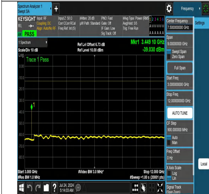
NTNV-N66-PC3-15-15-L-DFT-QPSK-Edge_1RB_Right-3000-12000-Ant1-PASS
