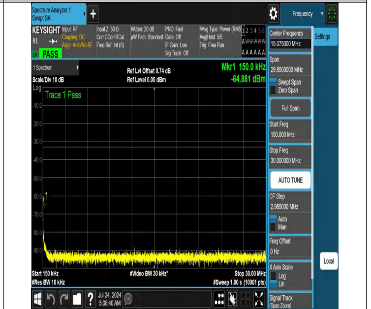
NTNV-N66-PC3-15-10-H-DFT-QPSK-Edge_1RB_Right-0.15-30-A nt1-PASS
